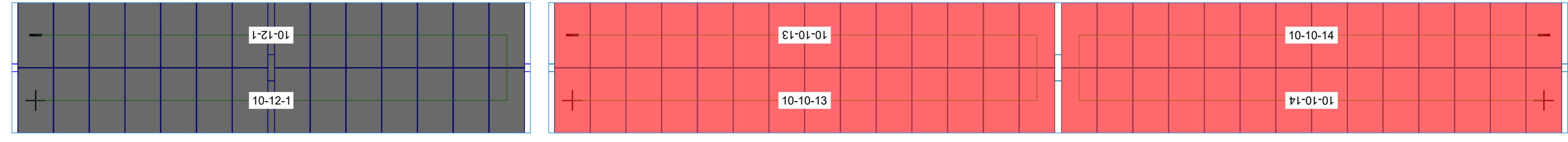
Particolare collegamento stringa - stringbox AREA PS10 (Esempio Campo 10 - String box n°12 - Stringa n°1) Scala 1:100
