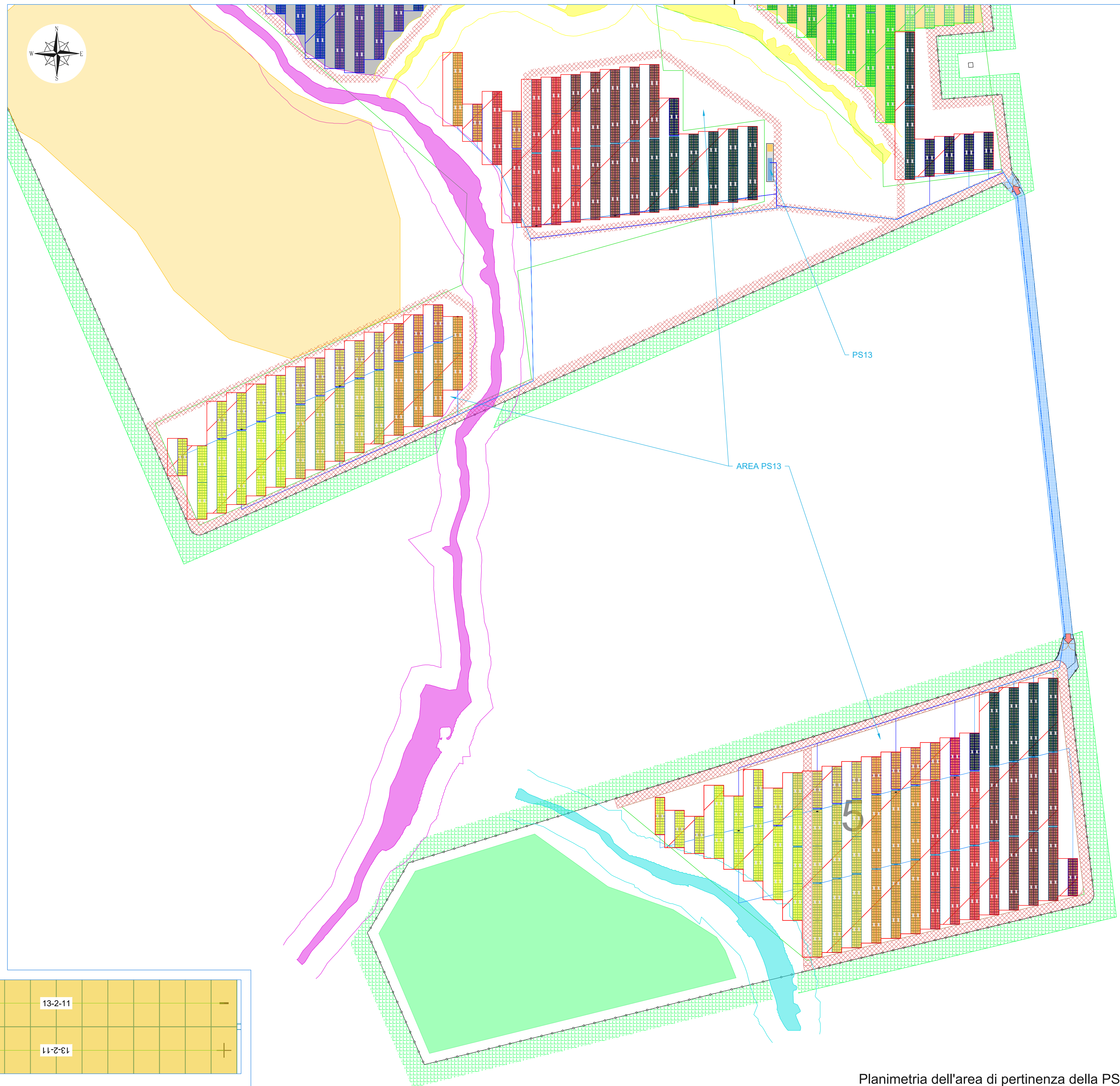
Planimetria dell'area di pertinenza della PS13 Scala 1:1.000
