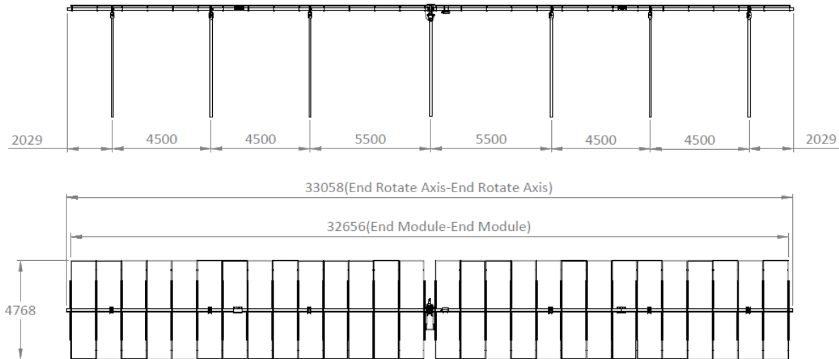
Figura 7: profilo strutturale strutture monoassiali
