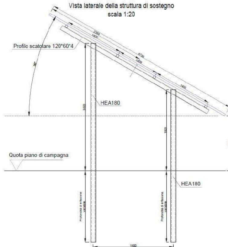
Figura 6: vista laterale struttura di sostegno
