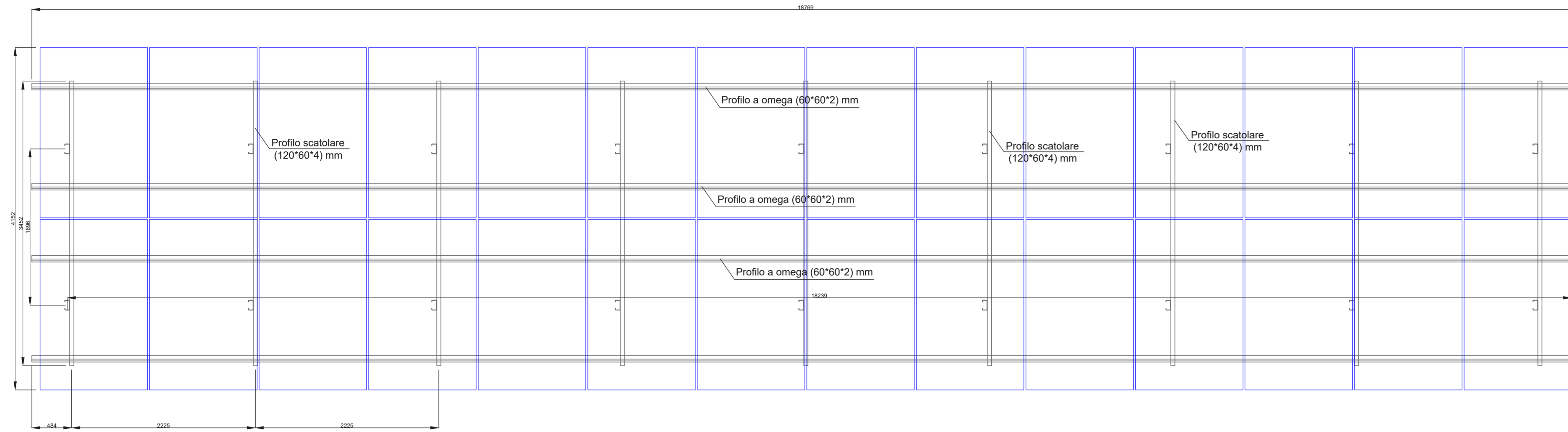
Pianta della struttura di sostegno scala 1:30
