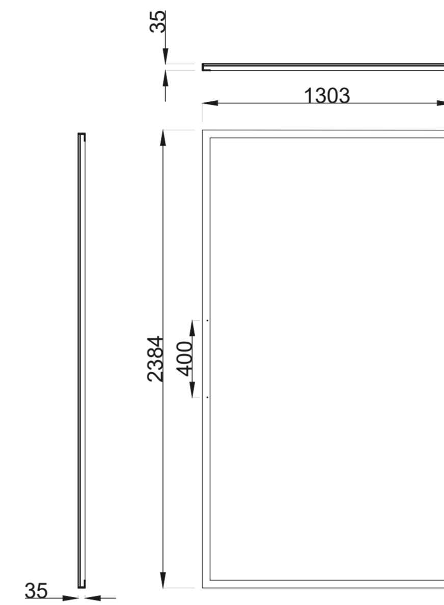
Vista laterale della struttura di sostegno scala 1:20
