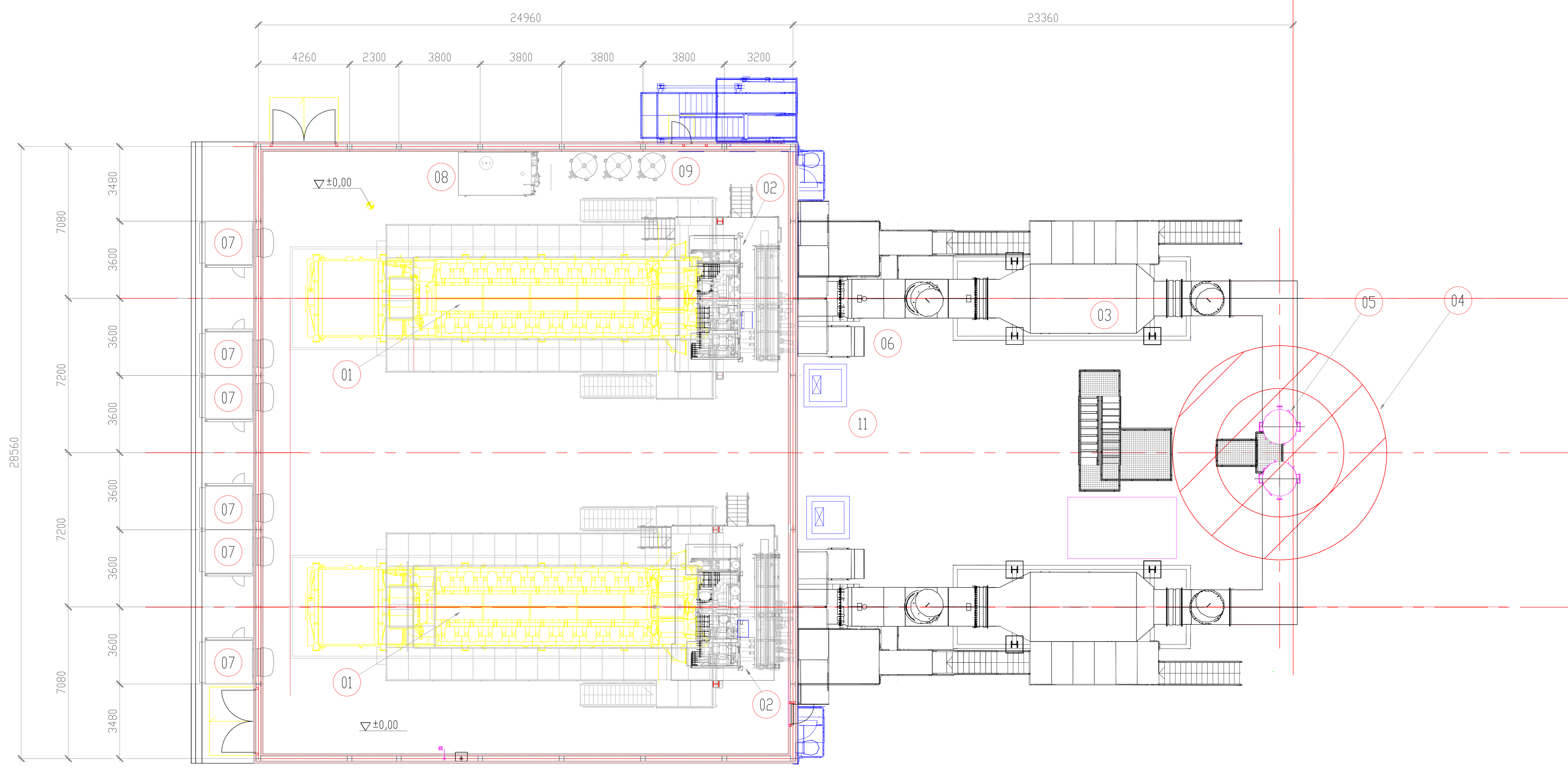
PLANIMETRIA SALA MACCHINE
