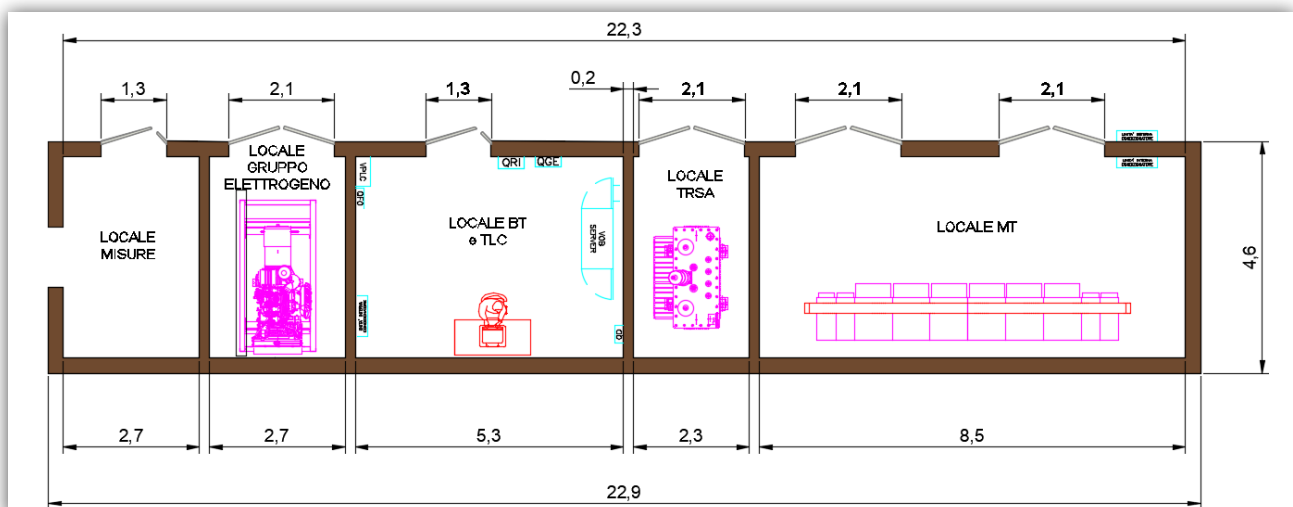
Fig. 30. Pianta dei locali presenti nella SSE Produttore
