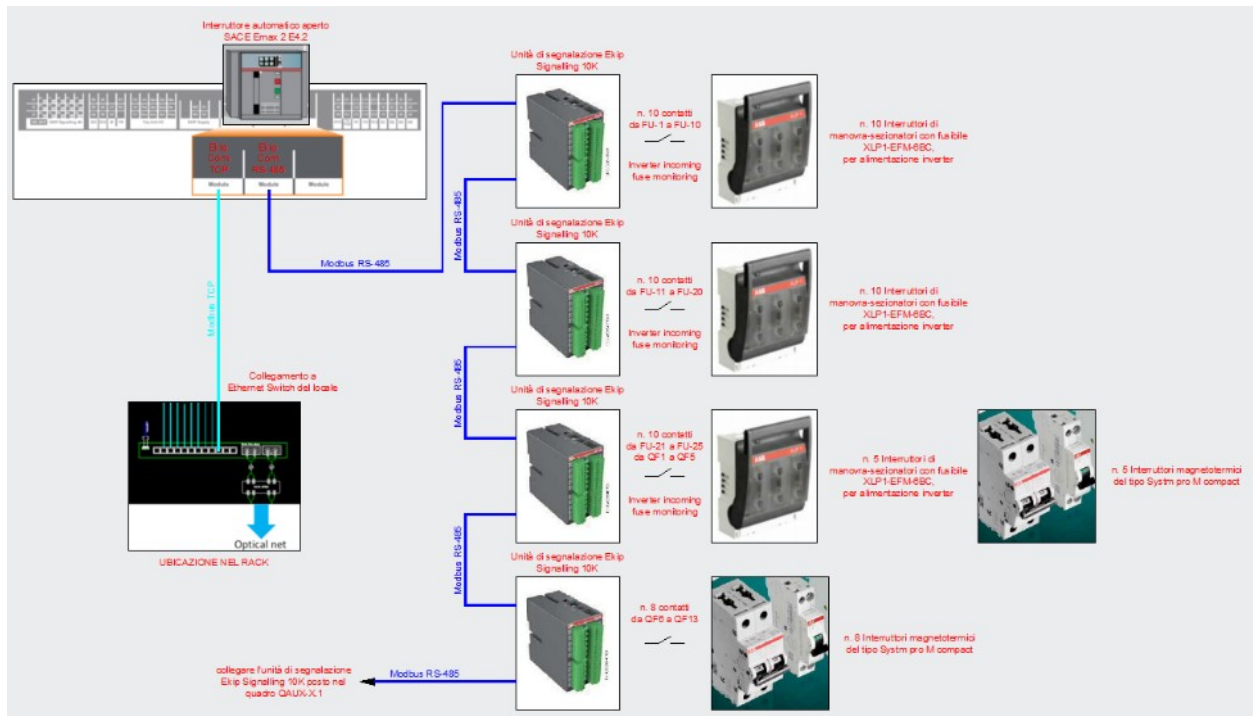
Fig. 41. Architettura del sistema di supervisione e controllo bt
