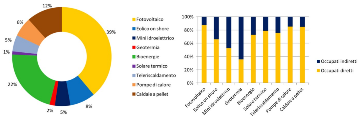
Fig. 43. Ricadute occupazionali delle diverse fonti di energia.
