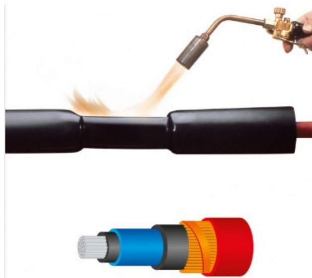
Fig. 23. Schema di esecuzione di un giunto MT.
