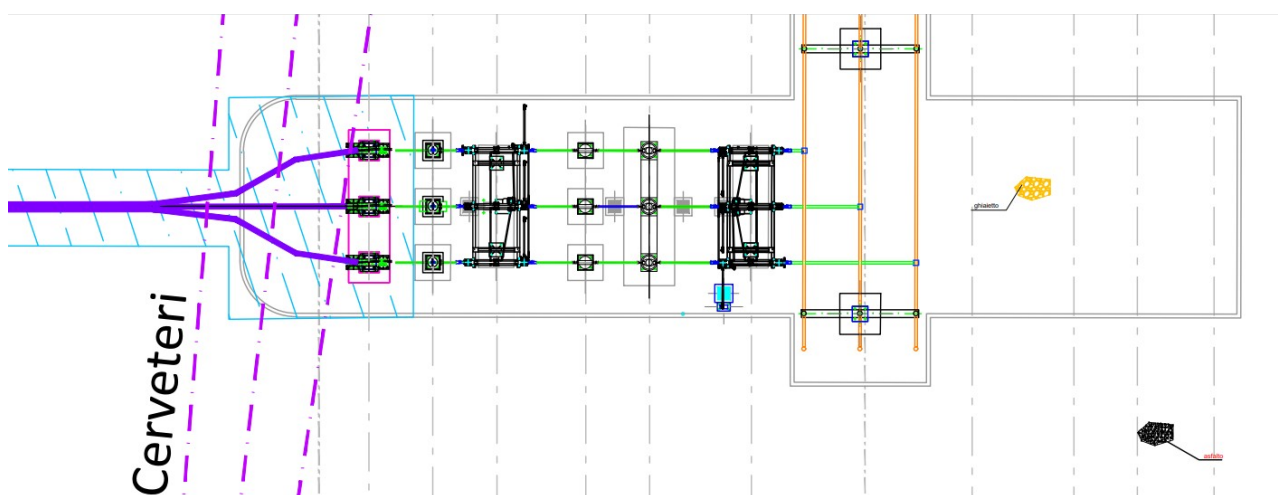
Fig. 34. Stralcio planimetrico dello stallo in area Cabina Primaria Enel
