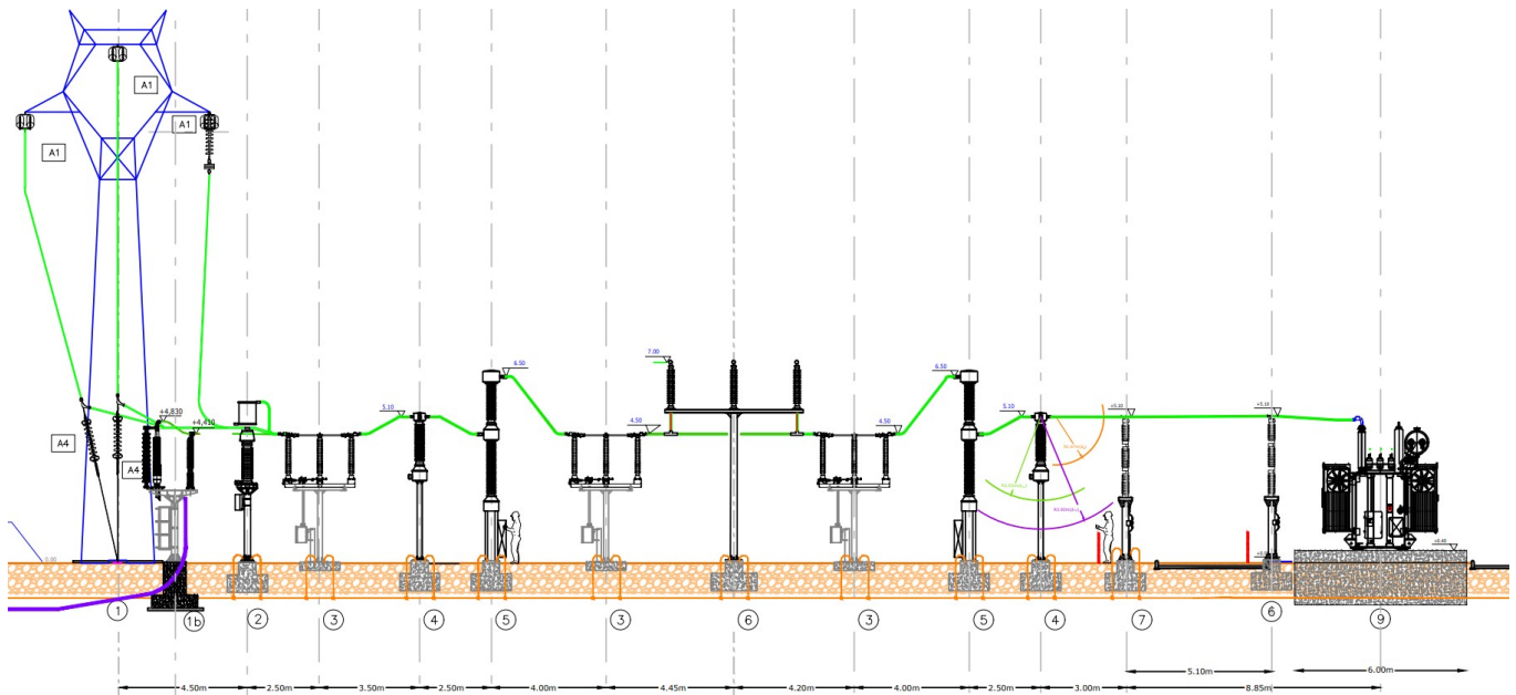
Fig. 35. Sezione elettromeccanica dello stallo in area Cabina Primaria Enel
