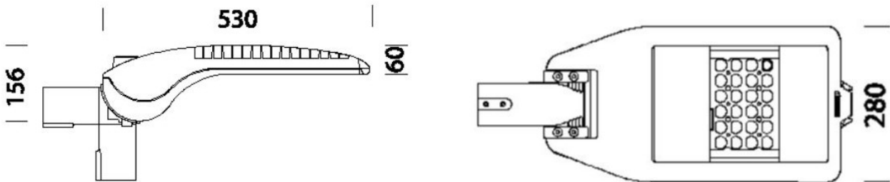
Fig. 38. Tipico apparecchio Illuminante a LED da montaggio a parete.
