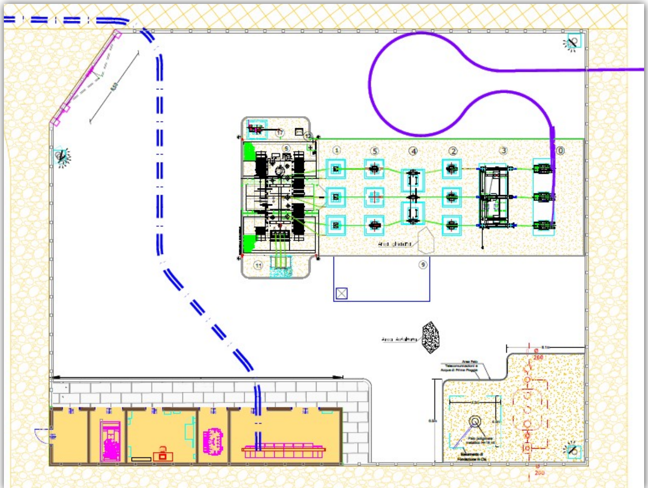
Fig. 28. Planimetria della SSE Produttore.
