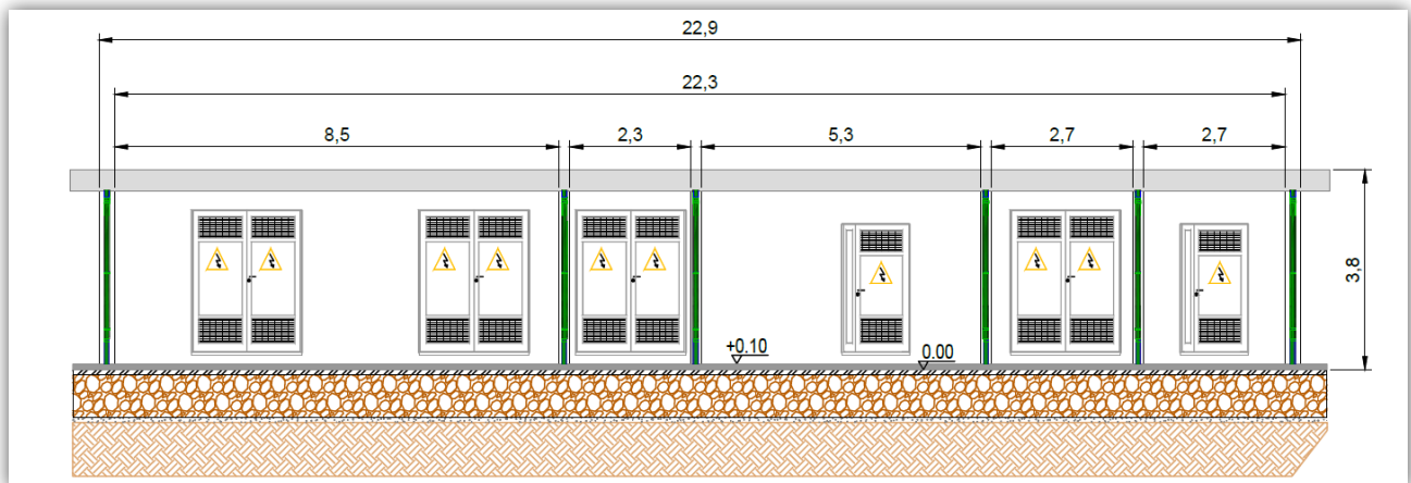
Fig. 32. Prospetto dei locali presenti nella SSE Produttore
