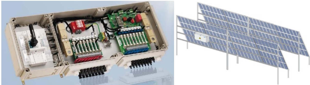
Fig. 14. Particolare di un raccoglitore di stringa e sua collocazione sulle strutture fotovoltaiche
