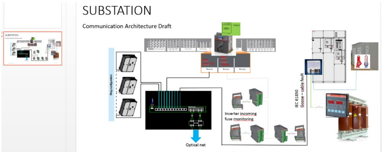
Fig. 40. Architettura del sistema di supervisione e controllo
