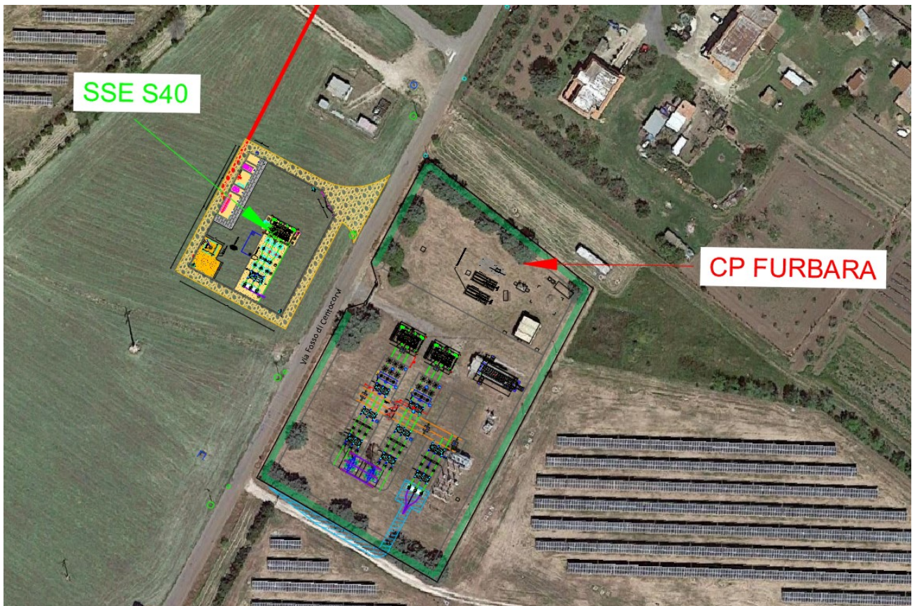
Fig. 27. Inquadramento su ortofoto con ubicazione della Sottostazione Produttore e della CP Enel
