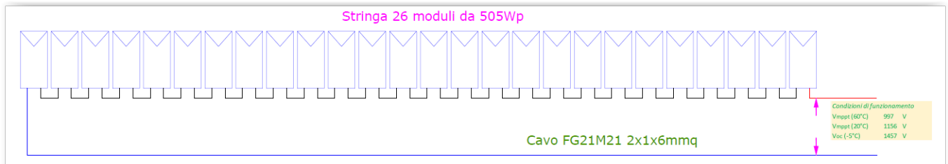
Fig. 13. Particolare serie moduli fotovoltaici.
