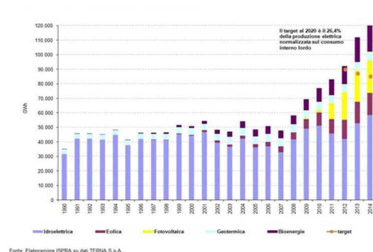
Fig. 44. Produzione lorda di energia da fonti energetiche rinnovabili in equivalente fossile sostituito.
