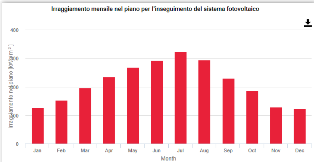
Fig. 6. Grafico andamento irraggiamento mensile nel piano interessato
