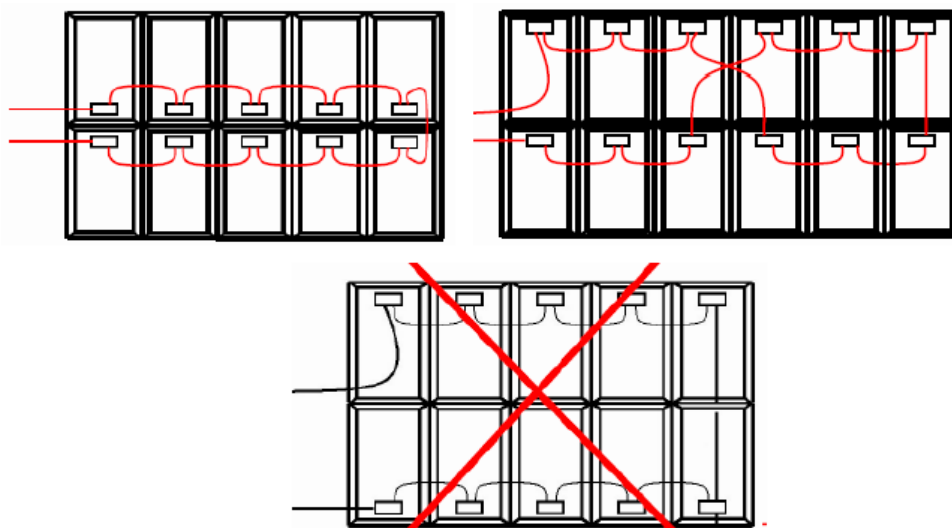
Fig. 42. Estratto dalla guida tecnica CEI 82-25 relativa alla modalità di cablaggio di stringa.
