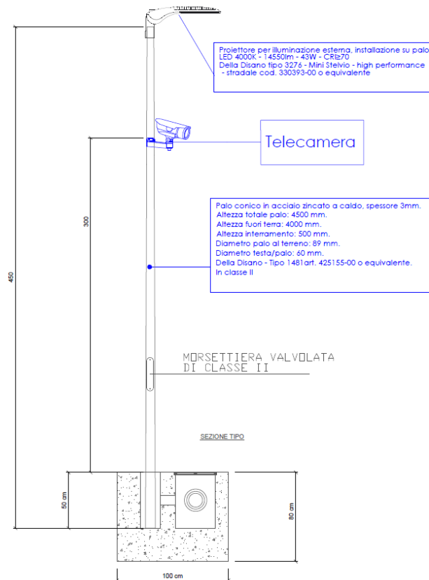
Fig. 39. Installazione telecamera su palo preposto.
