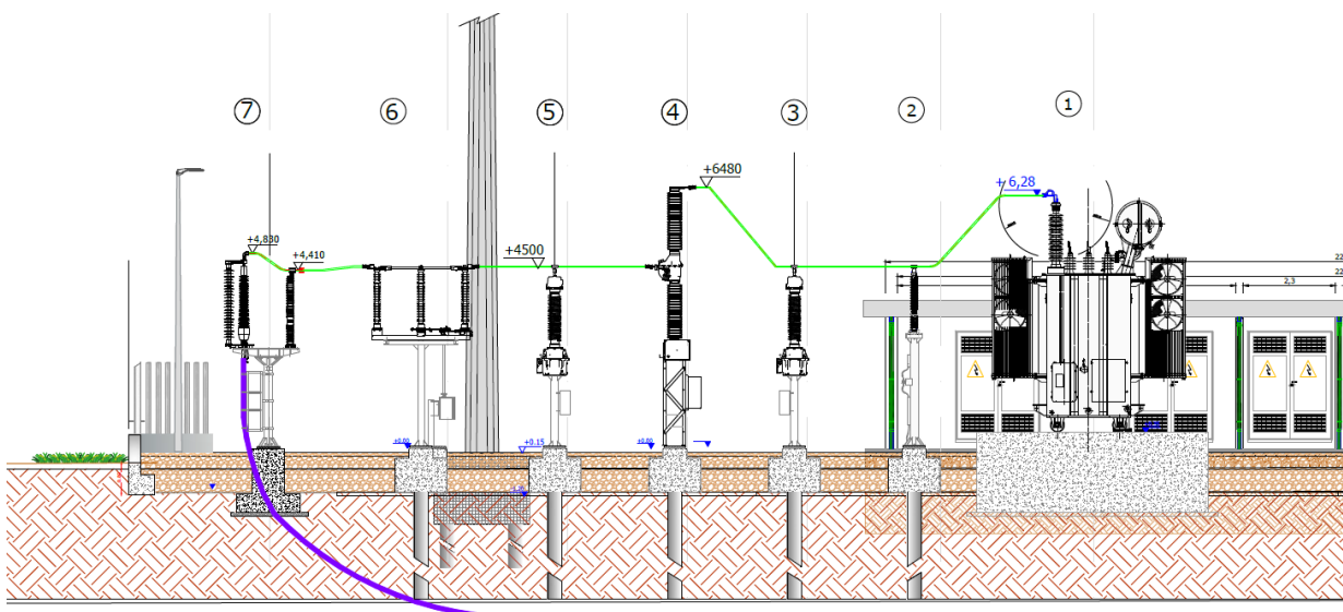
Fig. 29. Sezione elettromeccanica delle apparecchiature nella SSE Produttore
