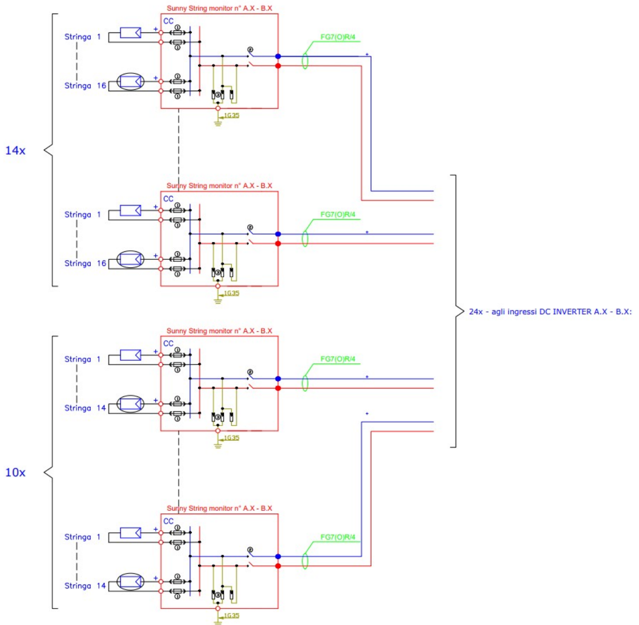
Fig. 4. Schema elettrico del collegamento tra quadri di stringa ed inverter centralizzato.
