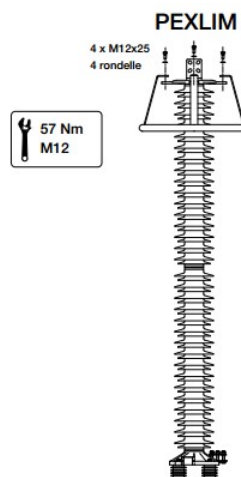
Fig. 19. Particolare di dettaglio dello scaricatore AT
