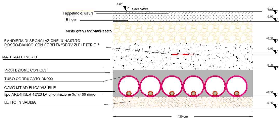
Fig. 16. Particolare scavo dei cavi MT in SSE in ingresso agli edifici quadro MT tipo shelter.
