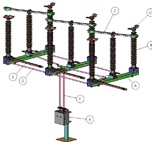
Fig. 20. Parti principali che compongono un sezionatore.
