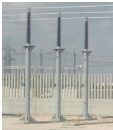
Fig. 24. Particolare in foto di tali supporti
