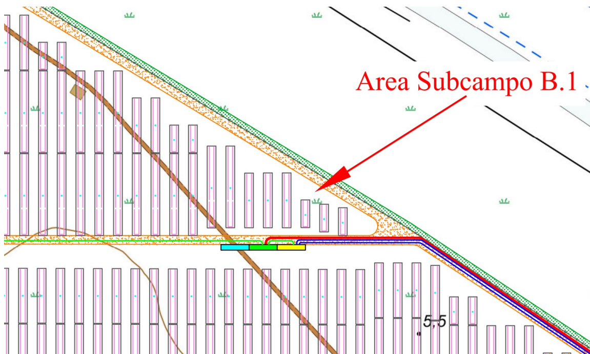
Fig. 7. Dettaglio della CdR: in verde le linee provenienti dai sottocampi e la cabina di raccolta; in rosso la linea dorsale verso la SSE.
