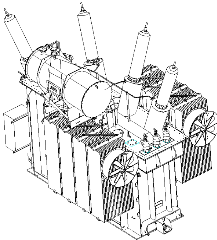
Fig. 25. Vista assometrica del trasformatore di progetto
