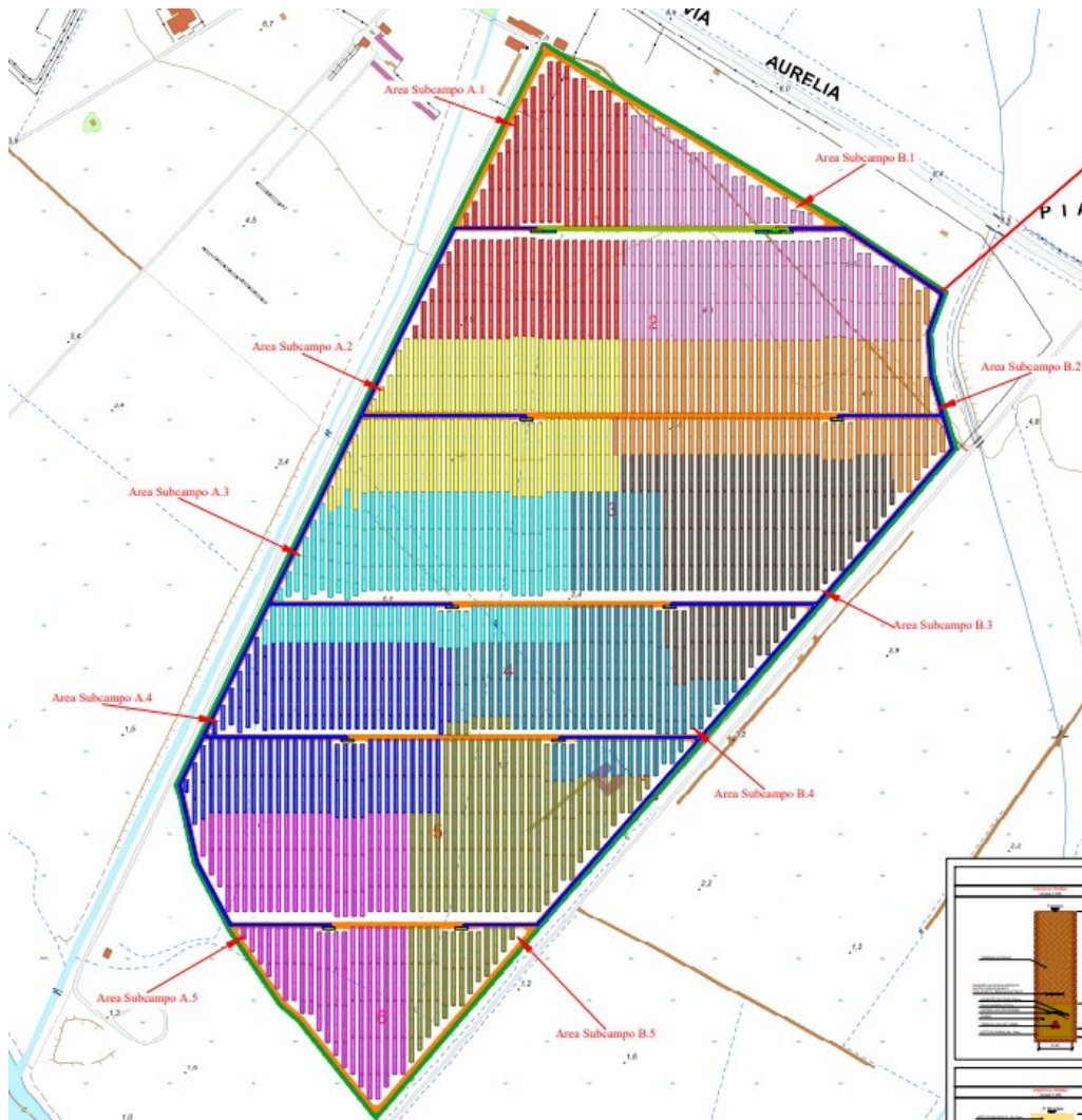
Fig. 6. Posizione della Cabina di raccolta contrassegnata con cerchio rosso; inoltre, vengono rappresentati tutti i sottocampi con colori diversi
