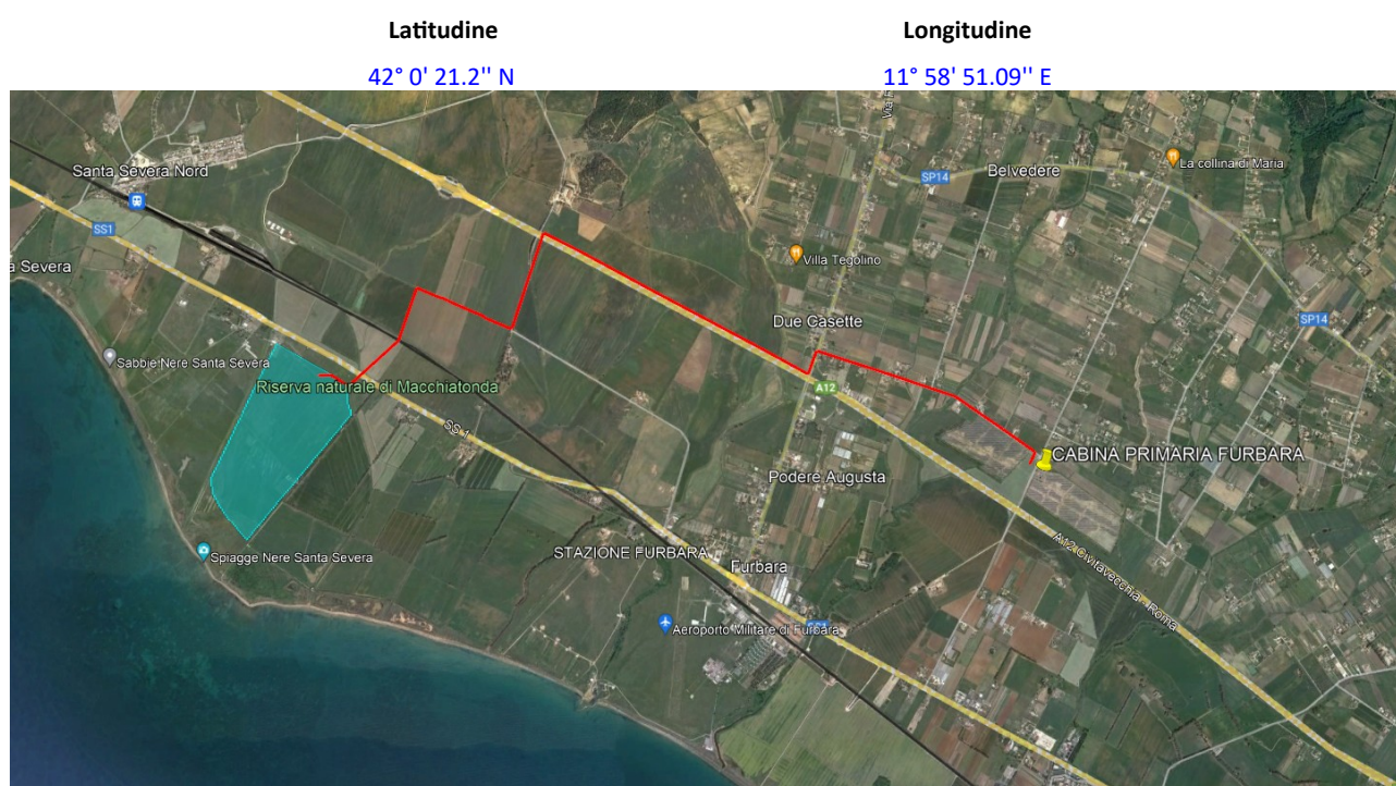
Fig. 1. Planimetria su ortofoto del progettato impianto Fotovoltaico: in colore ciano viene indicata l'area del generatore fotovoltaico, in rosso il cavidotto dorsale MT di collegamento tra il generatore e la Sottostazione Produttore, ubicata in prossimità della Cabina Primaria Enel
