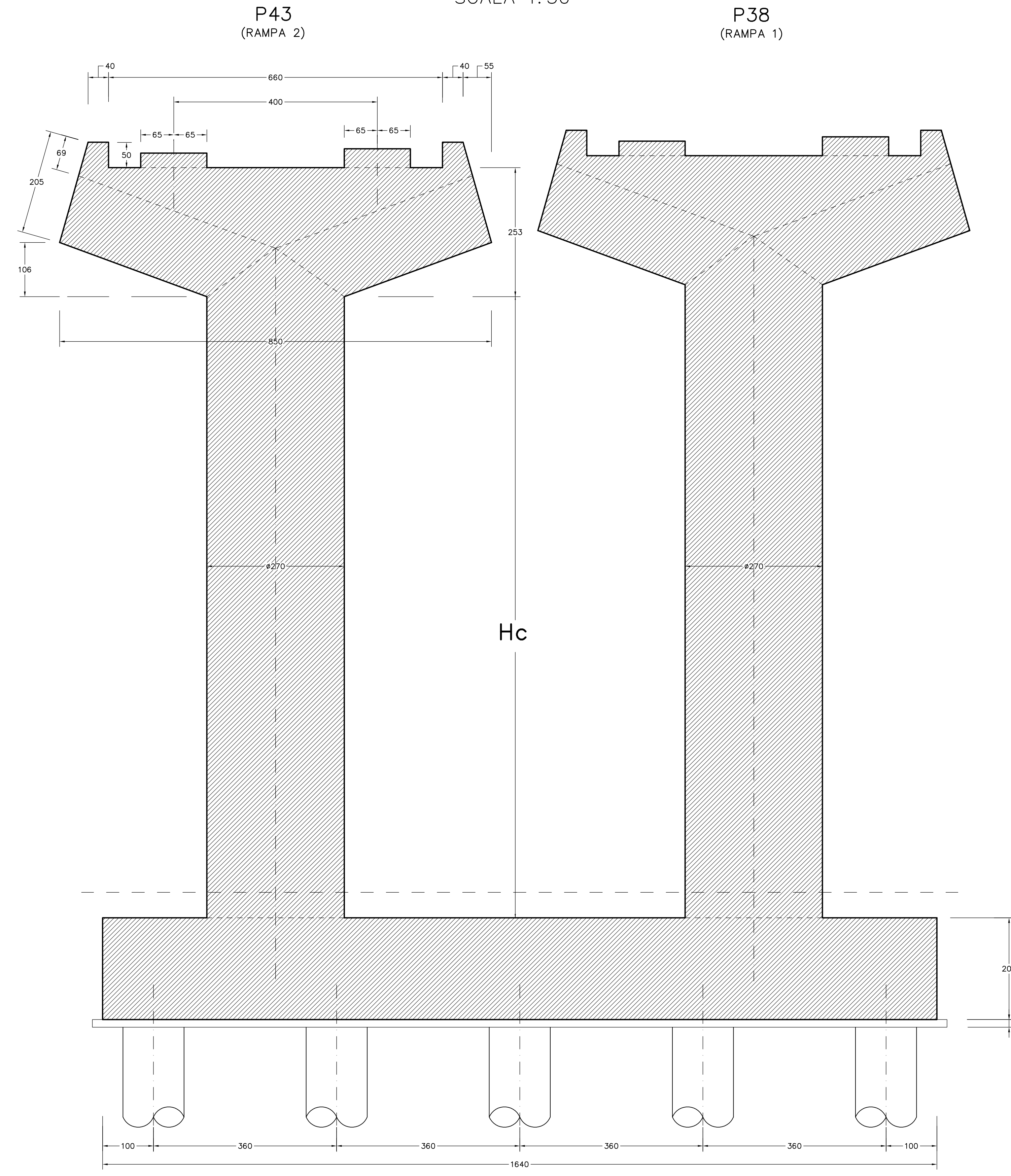
SEZIONE TRASVERSALE SCALA 1:50
