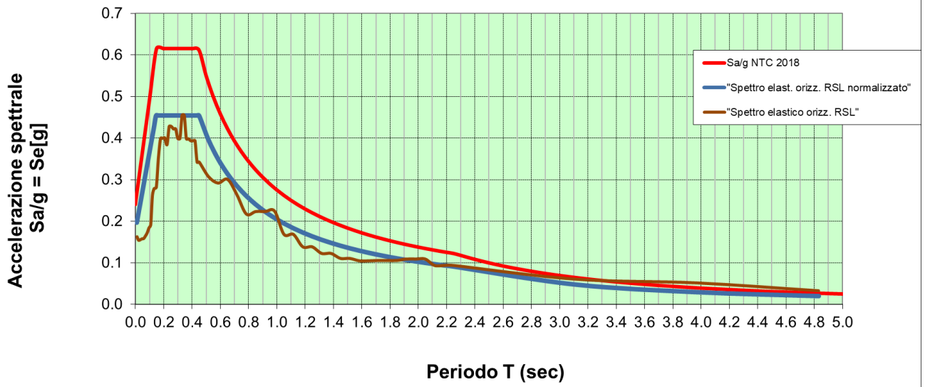
Spettro di risposta elastica per SLV - ( T_R=475 anni - smorzamento 5%) confronto NTC 2018 - RSL e spettro normalizzato da RSL
