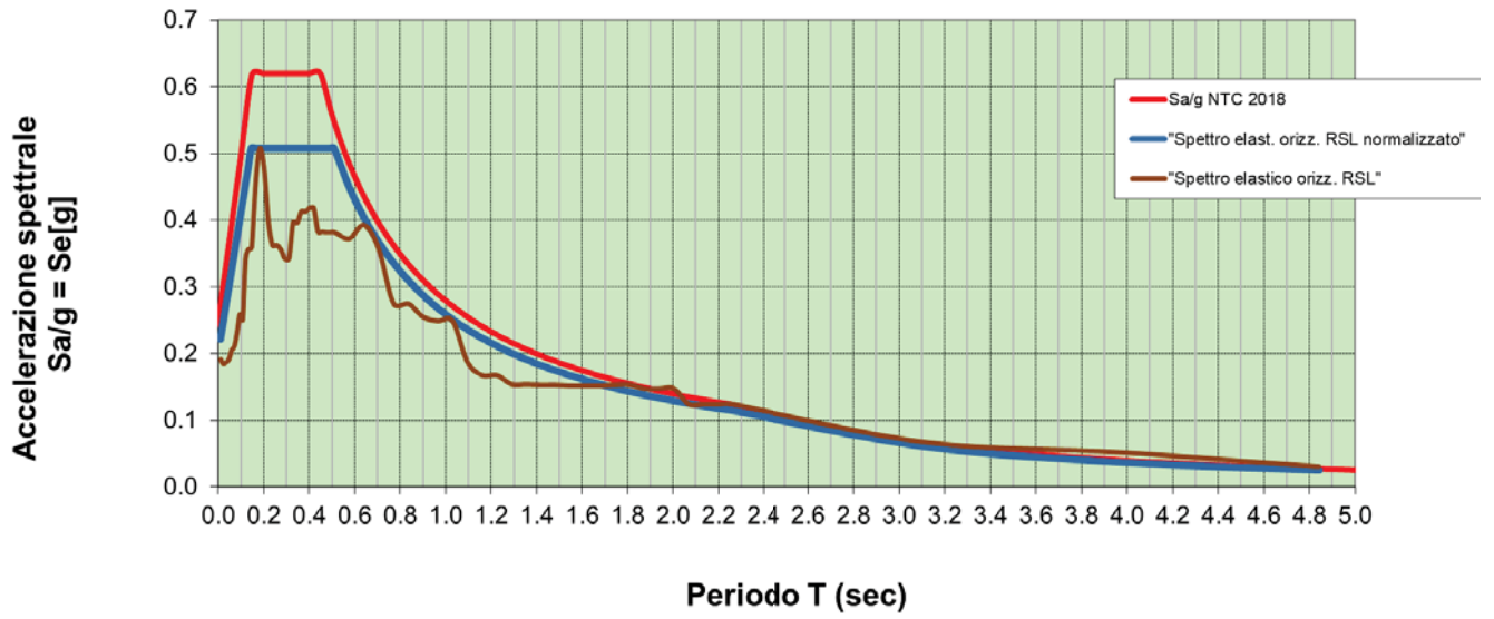
Spettro di risposta elastico per SLV - ( T_R=475 anni - smorzamento 5%) confronto NTC 2018 - RSL e spettro normalizzato da RSL
