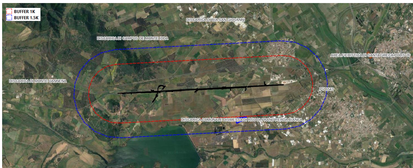
FIGURA 5-4: ASSE DI PROGETTO E SITI CONTAMINATI (DA SARDEGNAGEOPORTALE).
