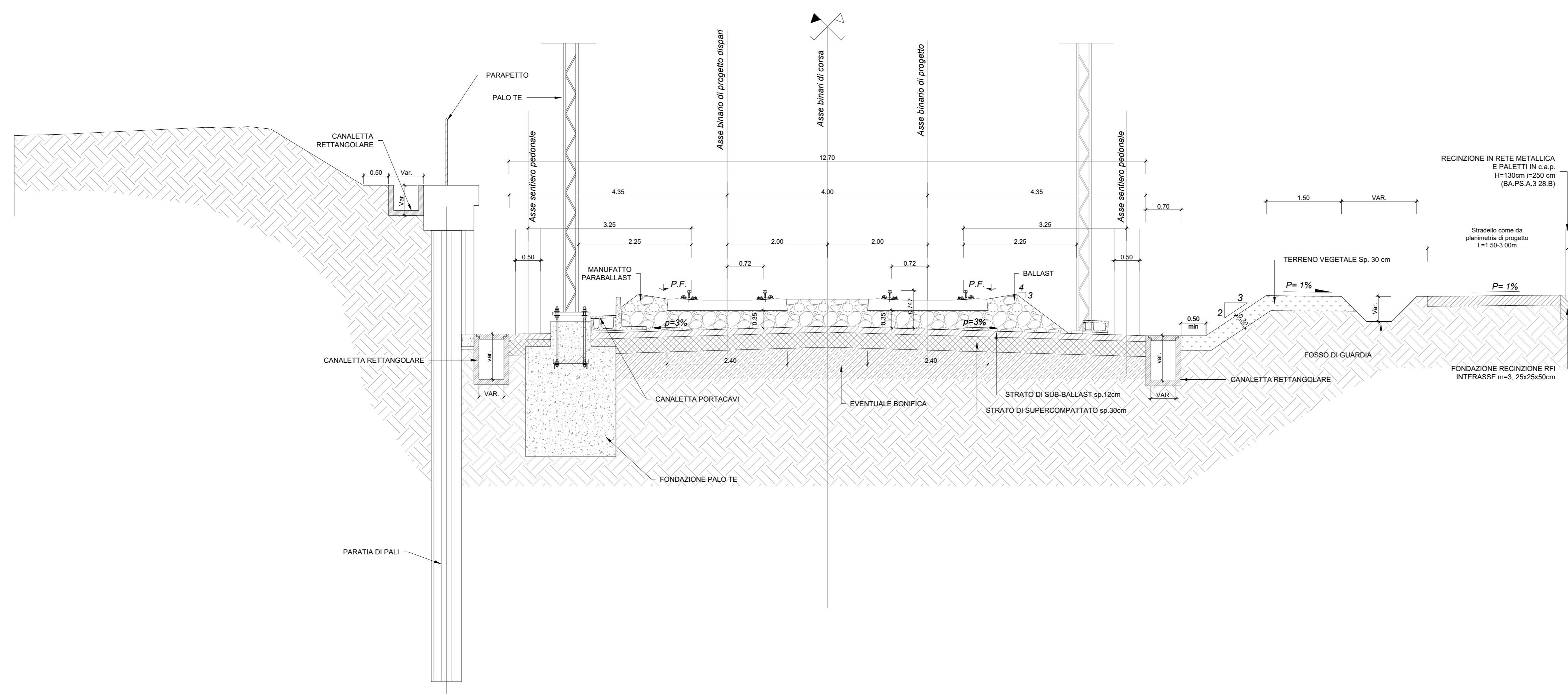
Sezione tipo a doppio binario in trincea con opera di sostegno
