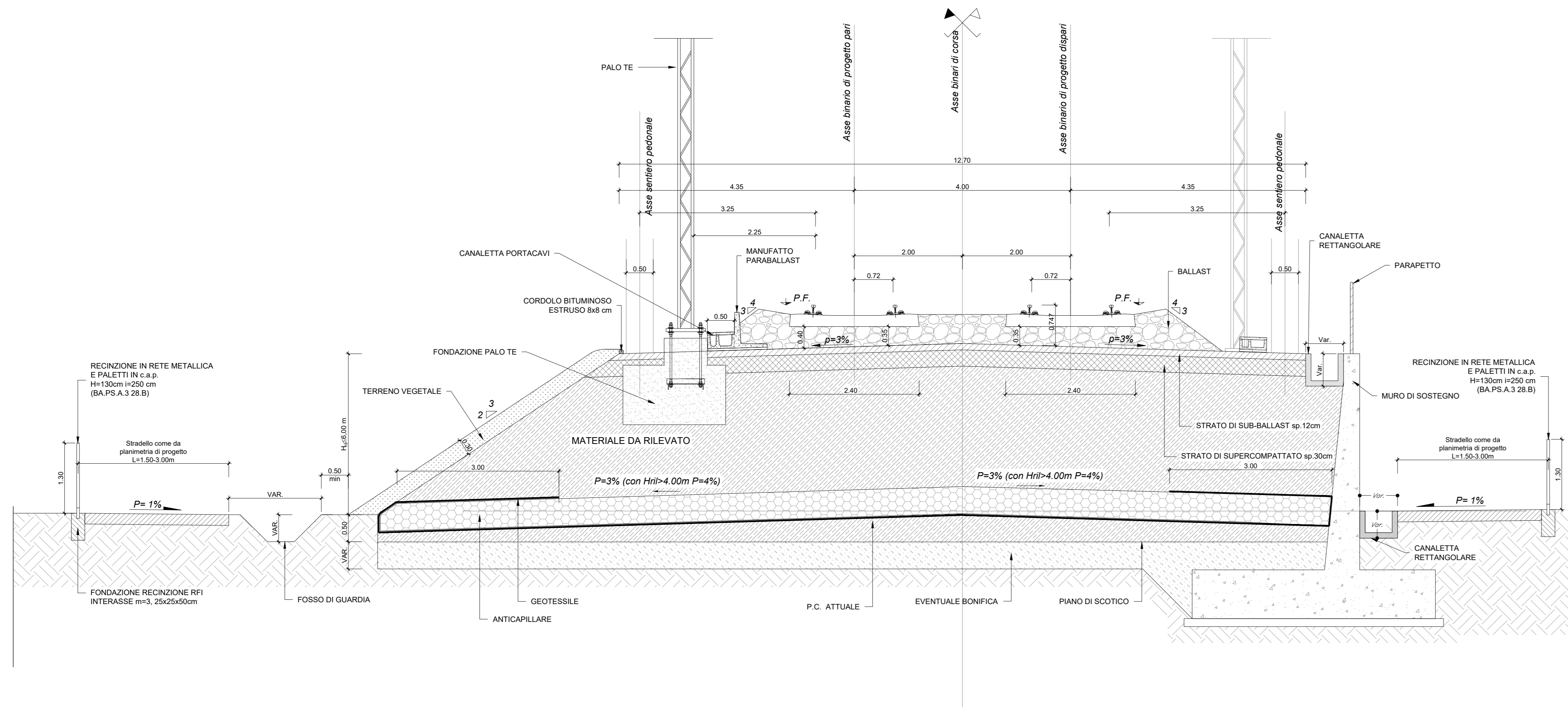
Sezione tipo in rilevato doppio binario con opera di sostegno
