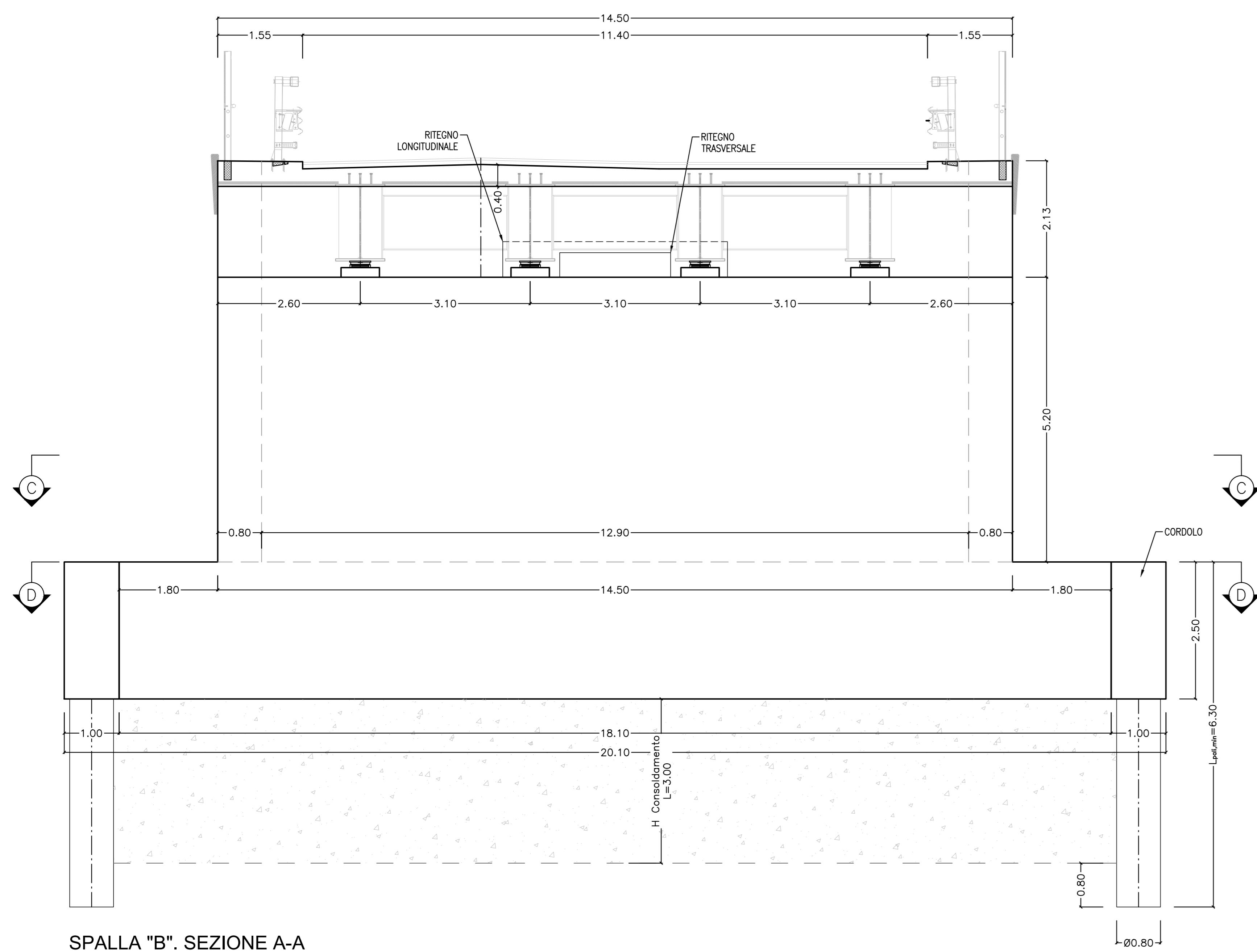
SPALLA "B". SEZIONE A-A SCALA 1:50
