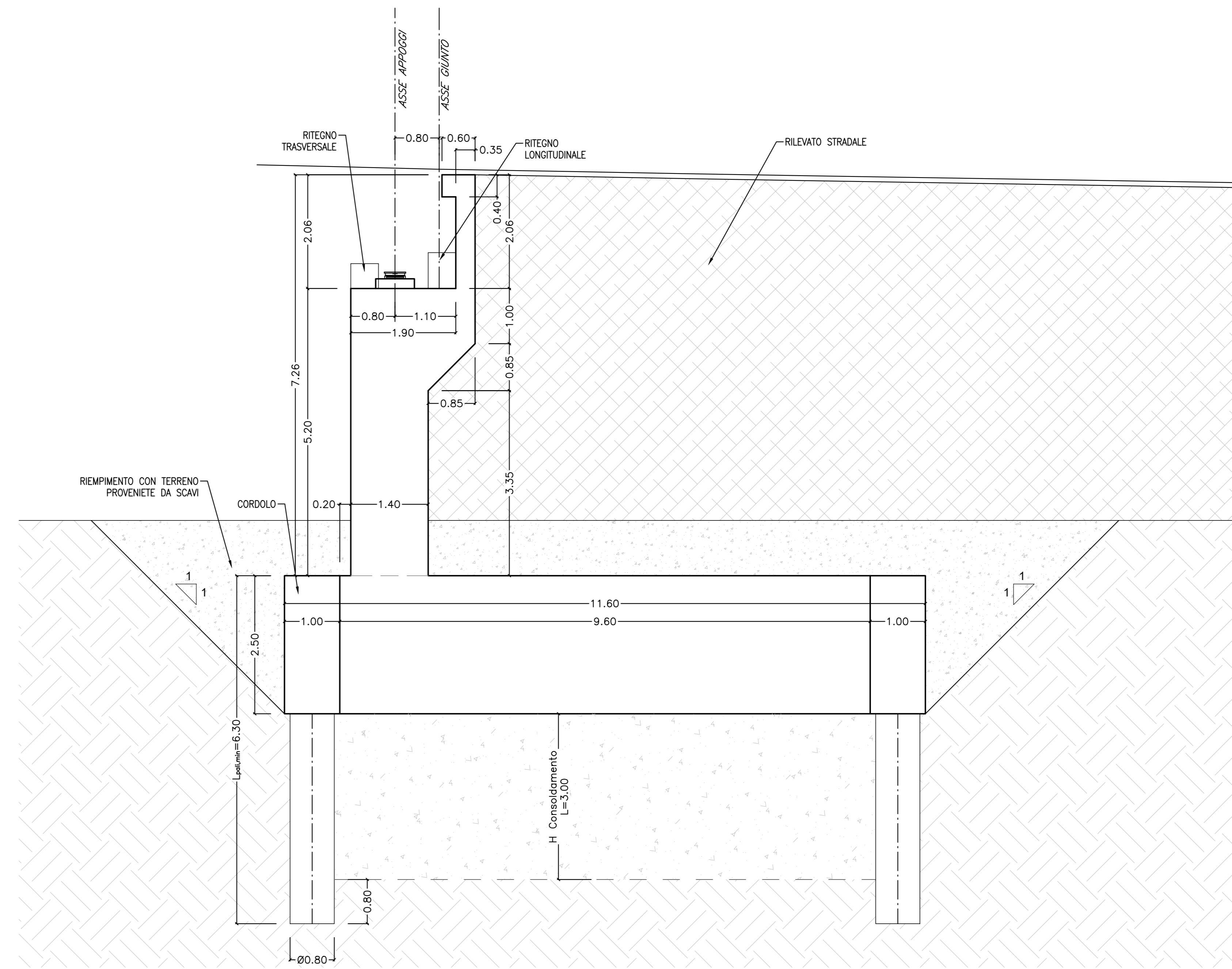
SPALLA "B". SEZIONE B-B SCALA 1:50
