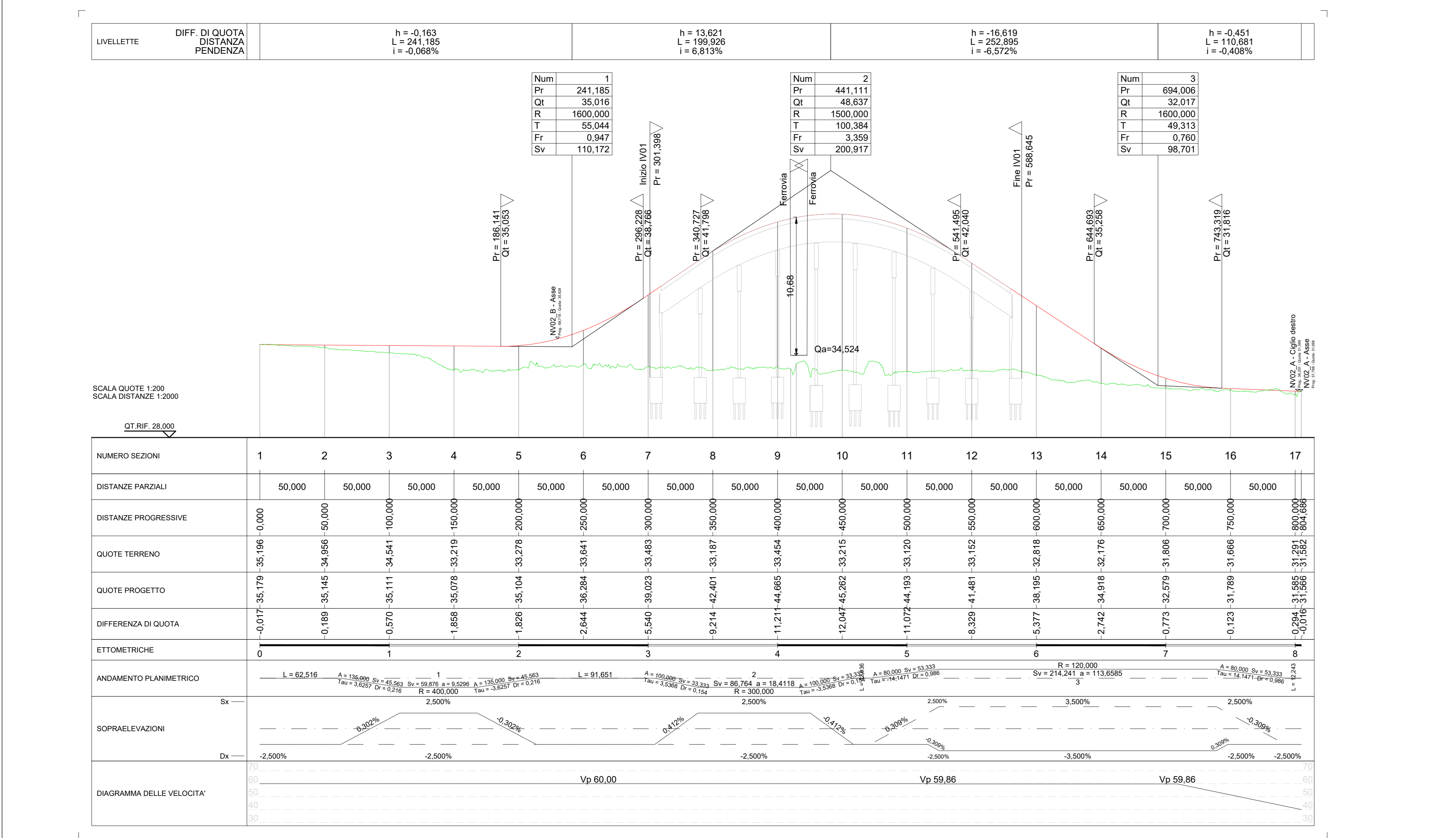
SCALA QUOTE 1:200 SCALA DISTANZE 1:2000
