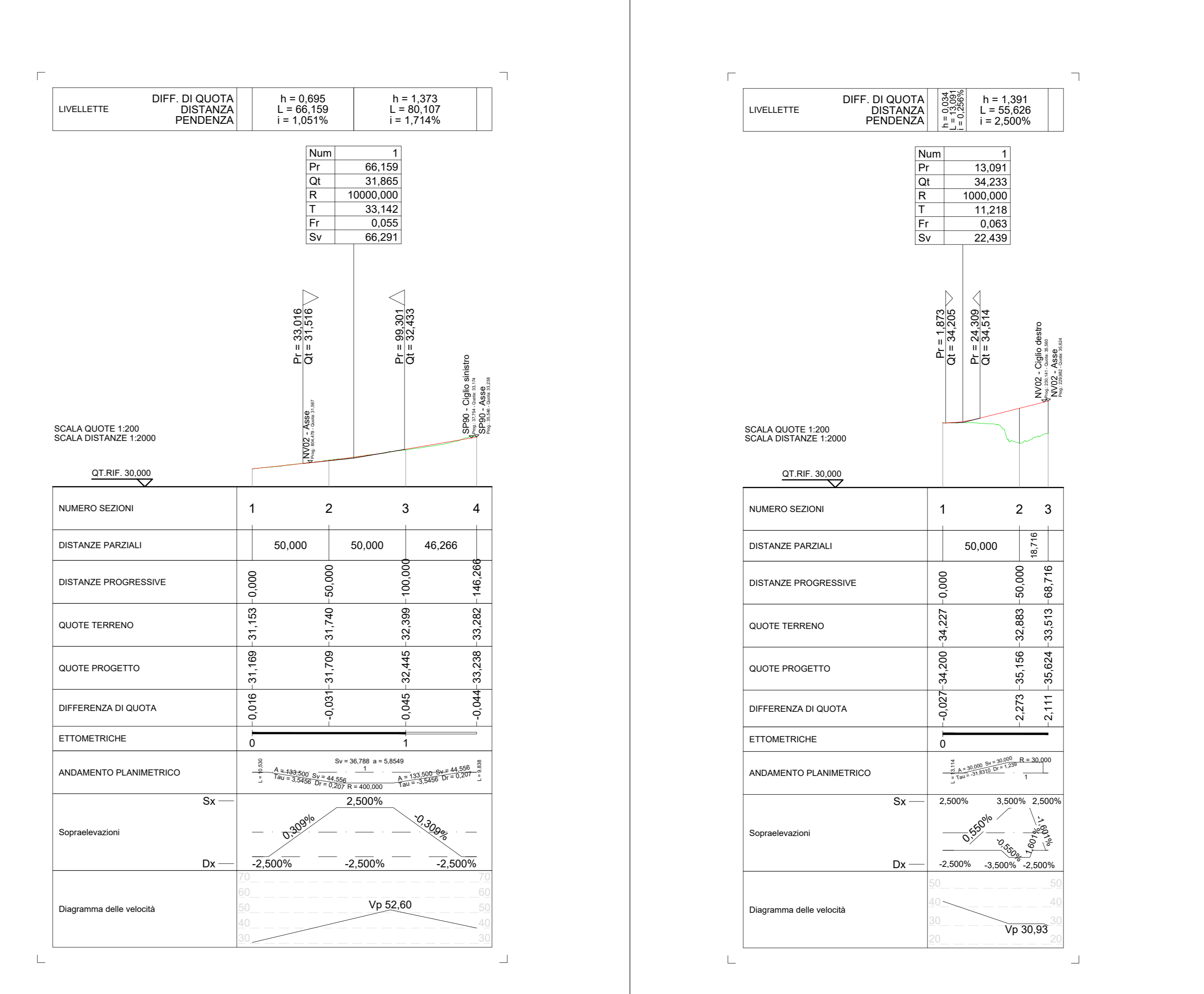
SCALA QUOTE 1:200 SCALA DISTANZE 1:2000
