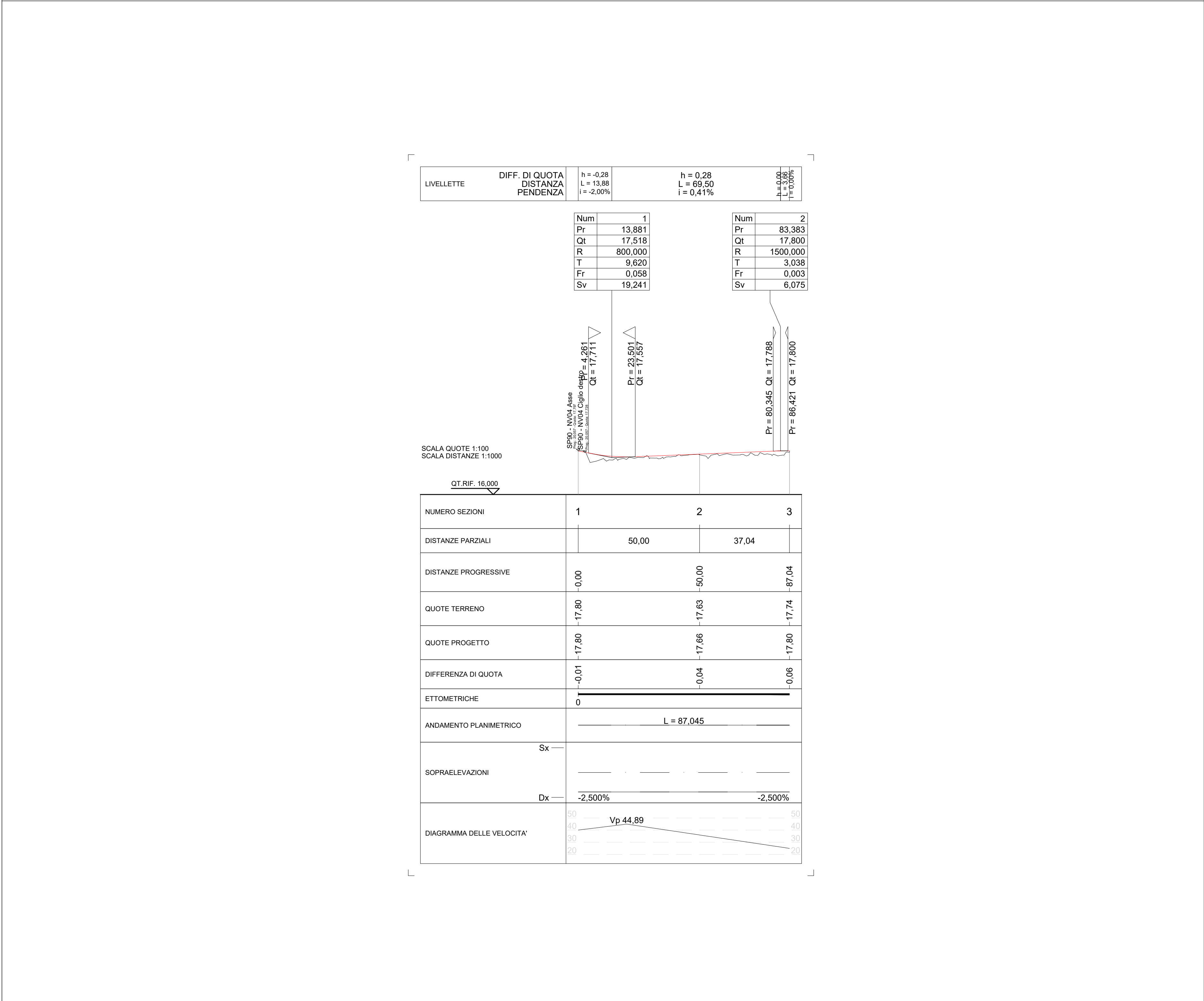
PROFILO LONGITUDINALE NV04
