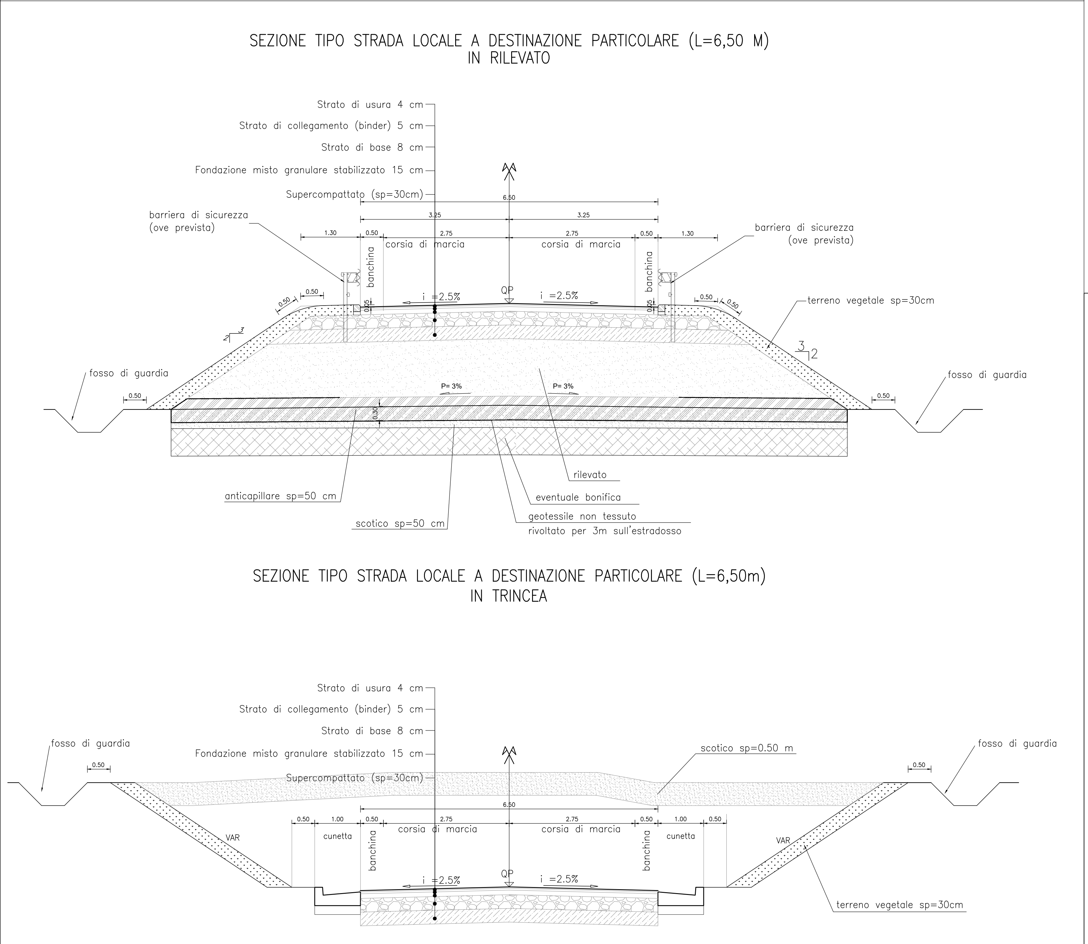
SEZIONI TIPO SCALA 1:50
