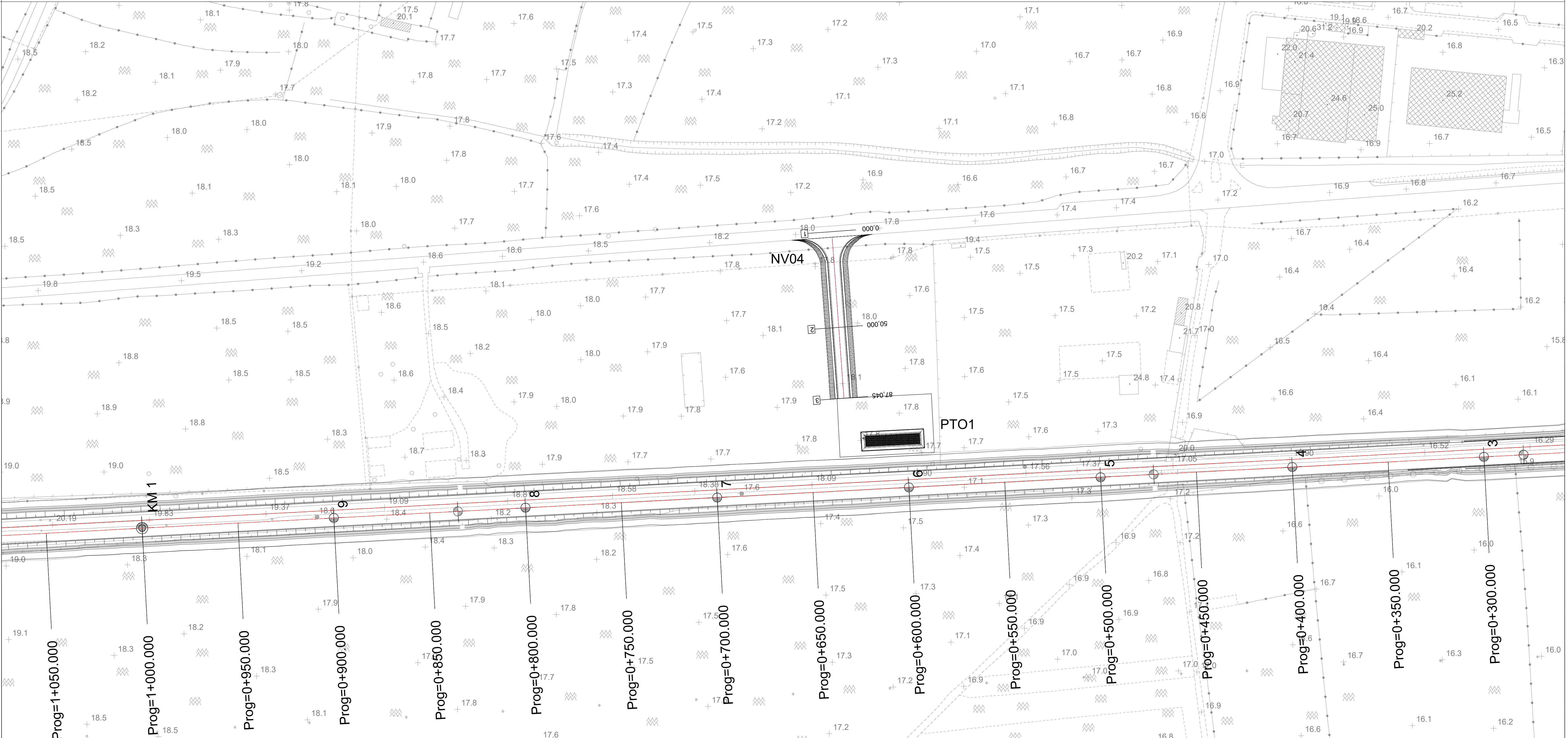
SCALA 1:1000
