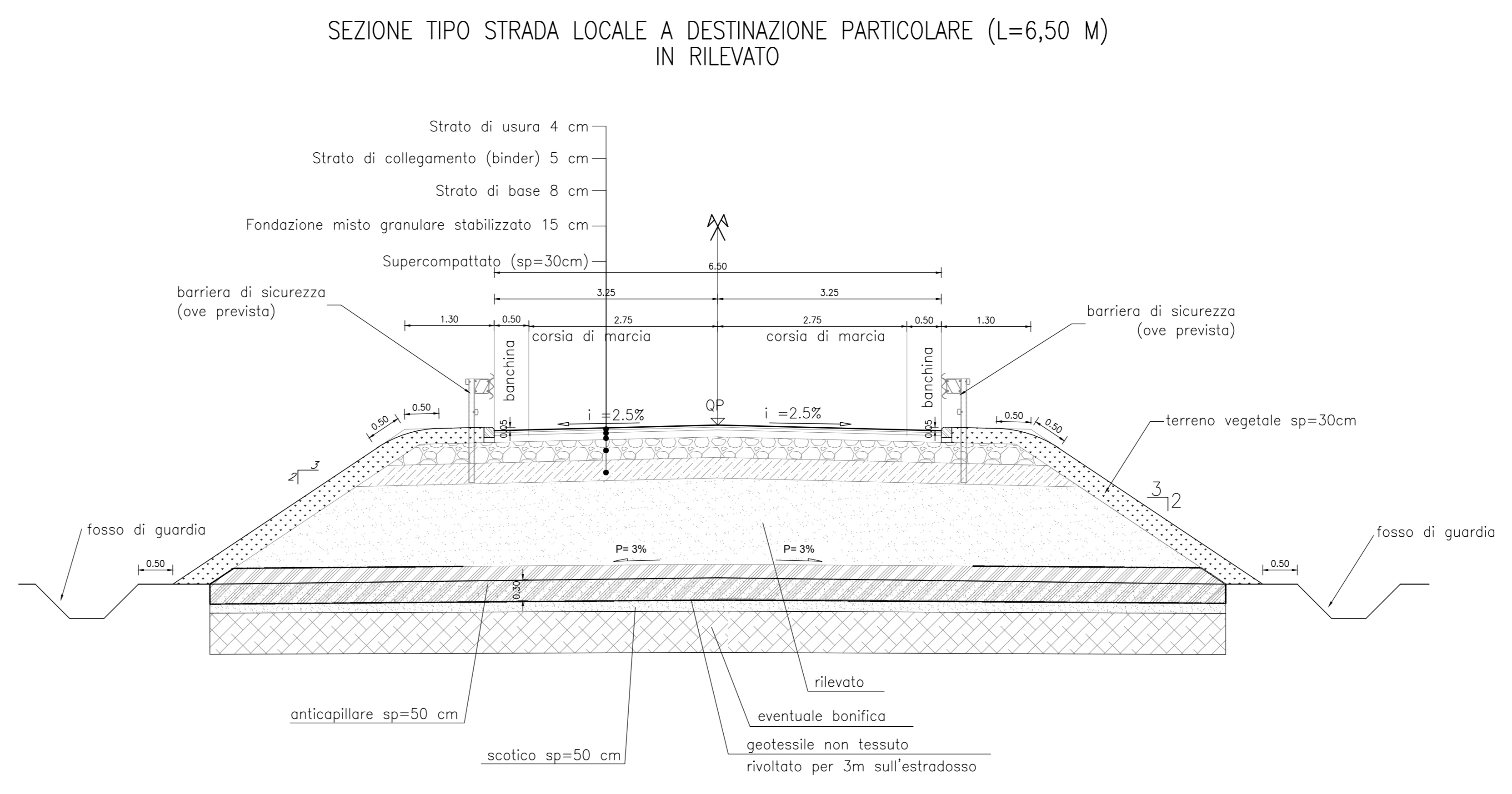
SCALA 1:1000 SEZIONI TIPO
