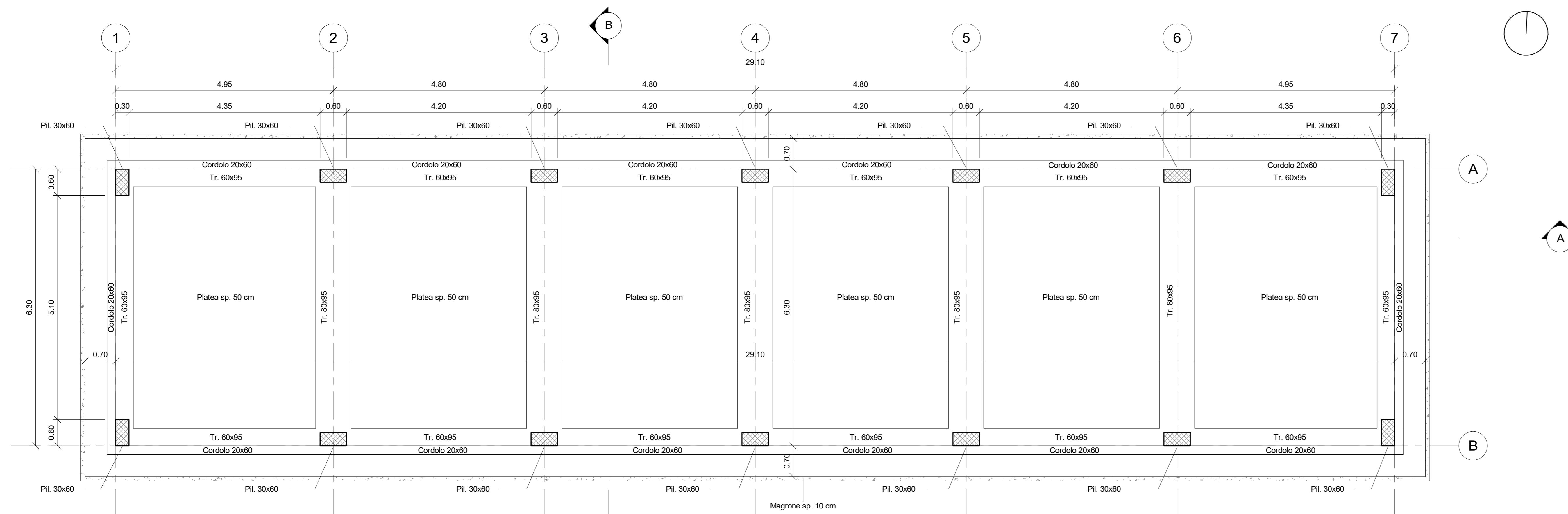
1 Carpenteria Fondazione 1 : 50
