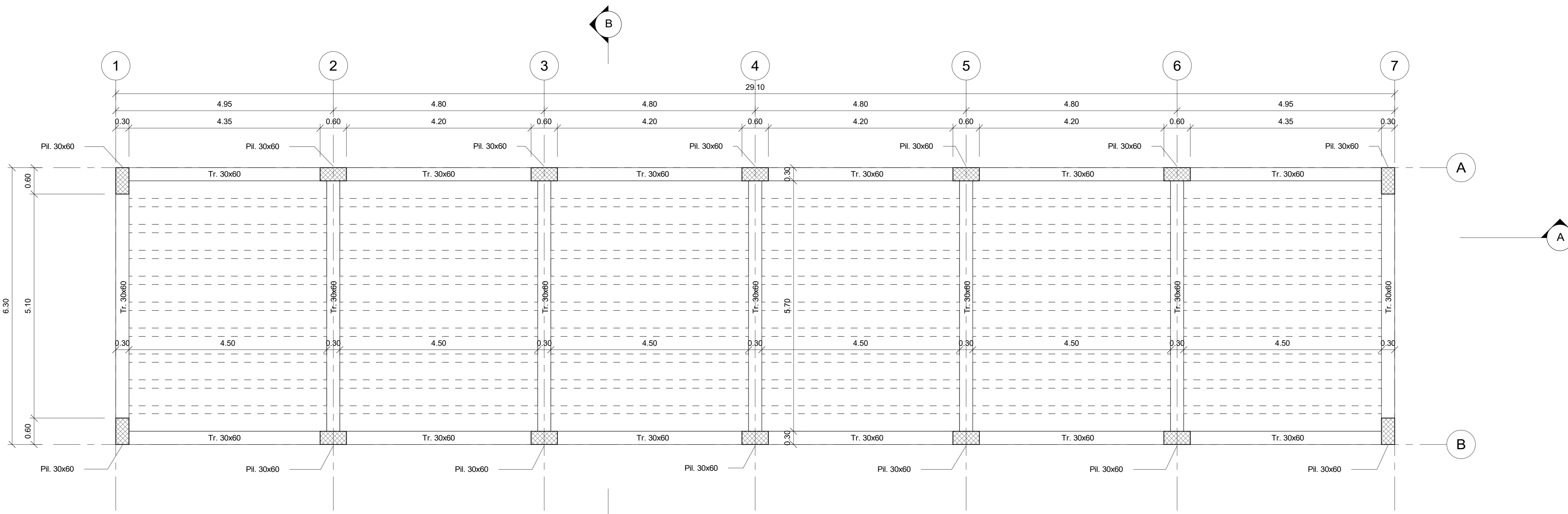
2 Carpenteria Copertura 1 : 50
