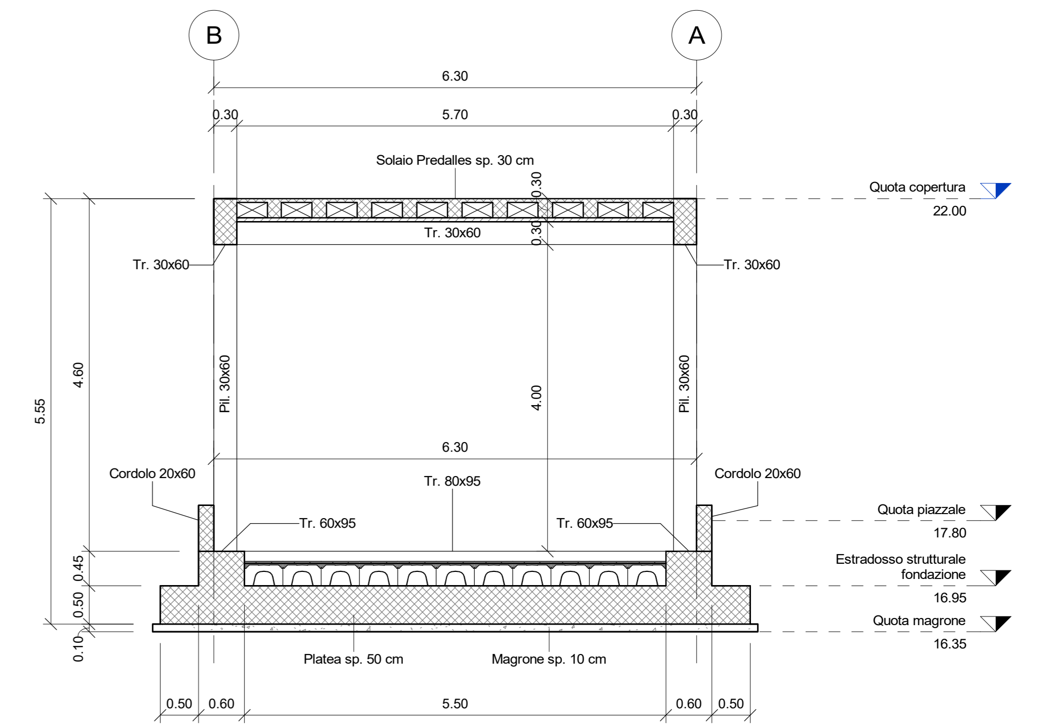
4 Sezione B 1 : 50
