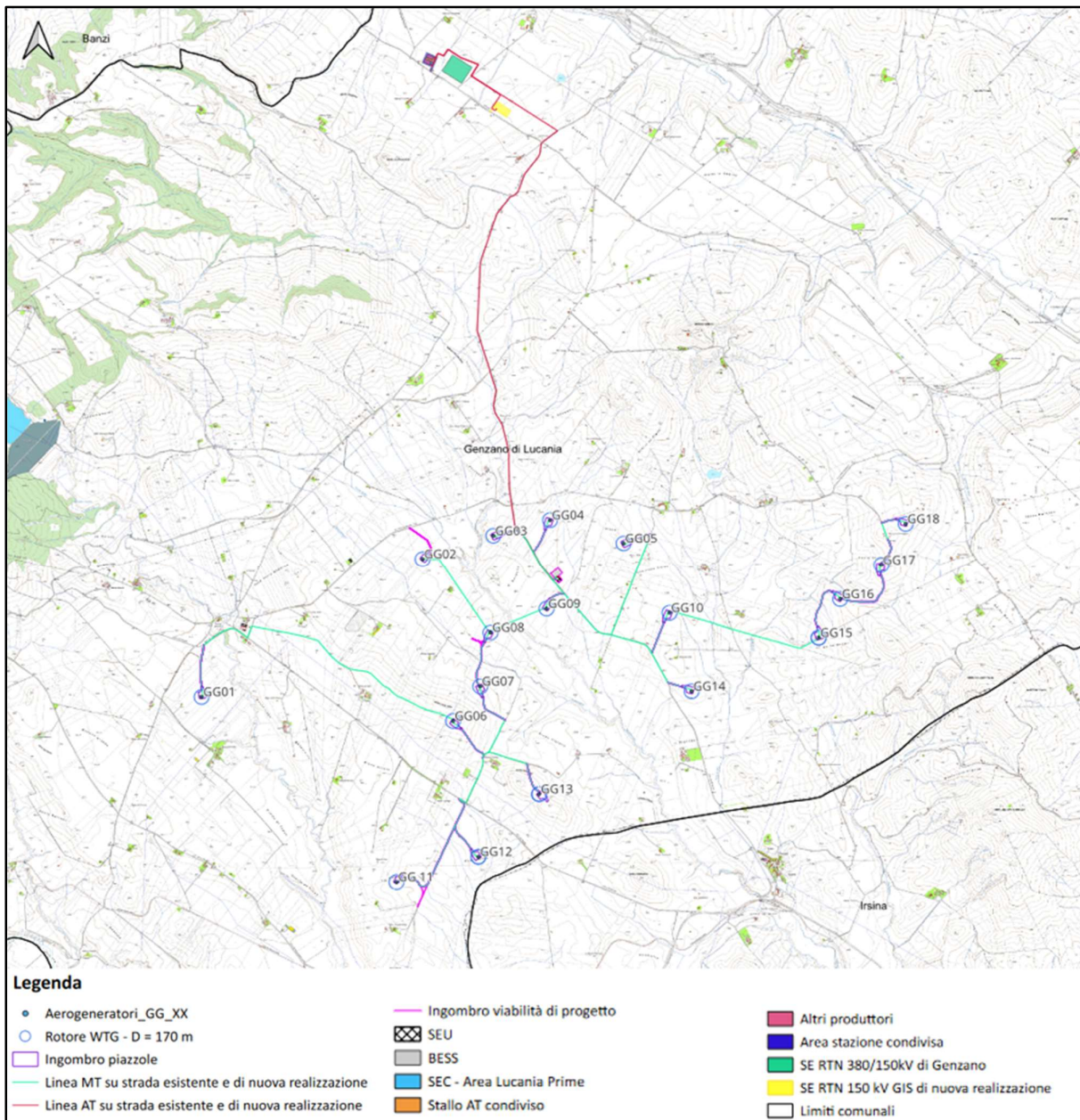
Figura 6.1: Inquadramento territoriale del Parco Eolico Genzano con i limiti amministrativi dei comuni interessati
