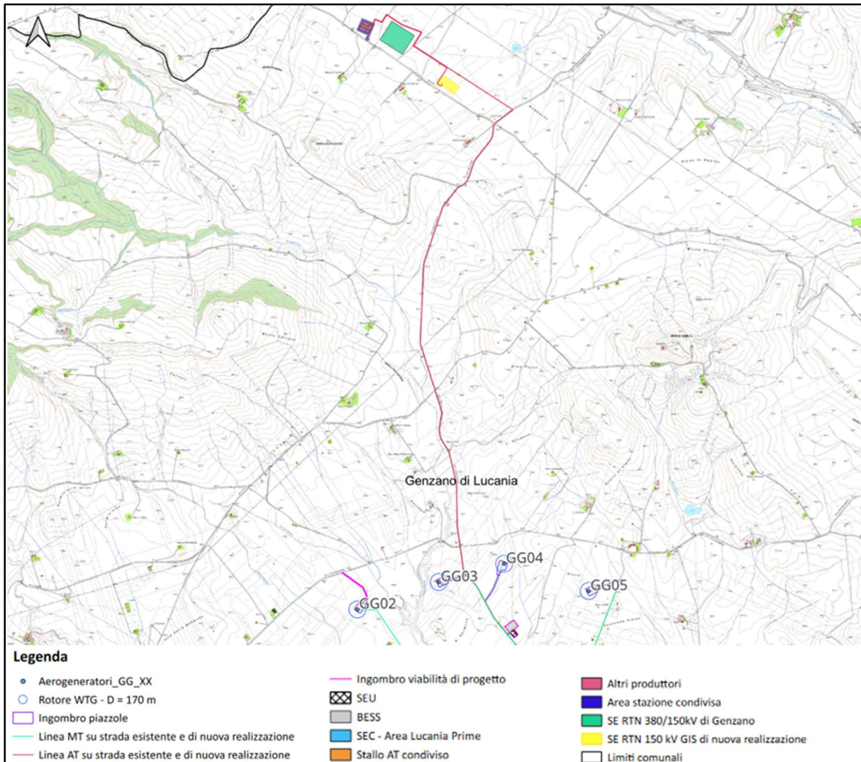
Figura 6.2: Soluzione di connessione a 150 kV in corrispondenza dell'ampliamento della SE RTN Terna 380/150 kV di Genzano
