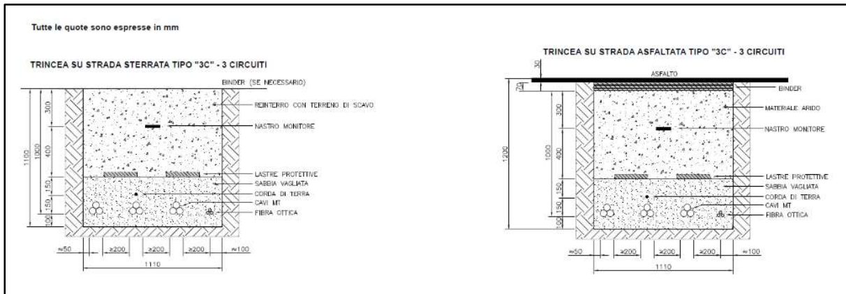
Figura 6.3.4.4: Sezioni tipiche delle trincee cavidotto per tre terne di cavi in parallelo su strada sterrata e asfaltata
