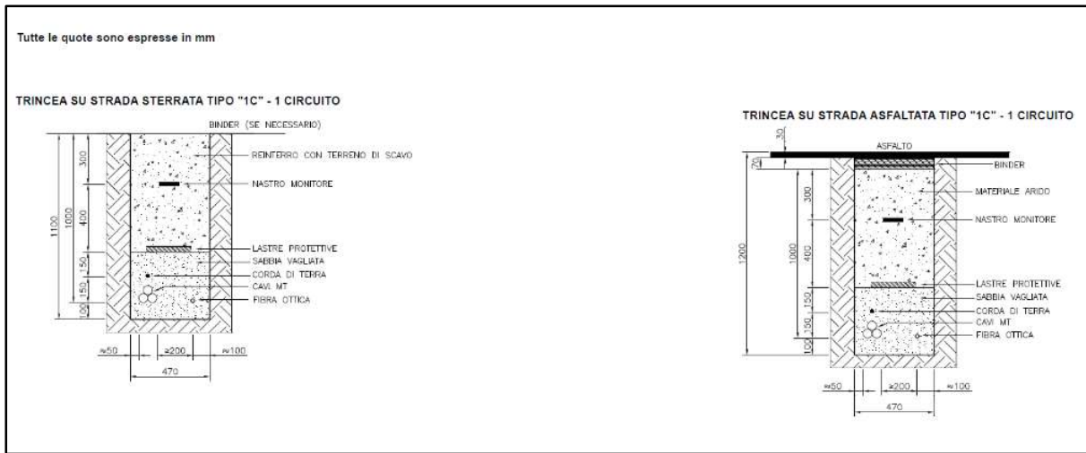
Figura 6.3.4.2: Sezioni tipiche delle trincee cavidotto per una terna di cavi in parallelo su strada sterrata e asfaltata
