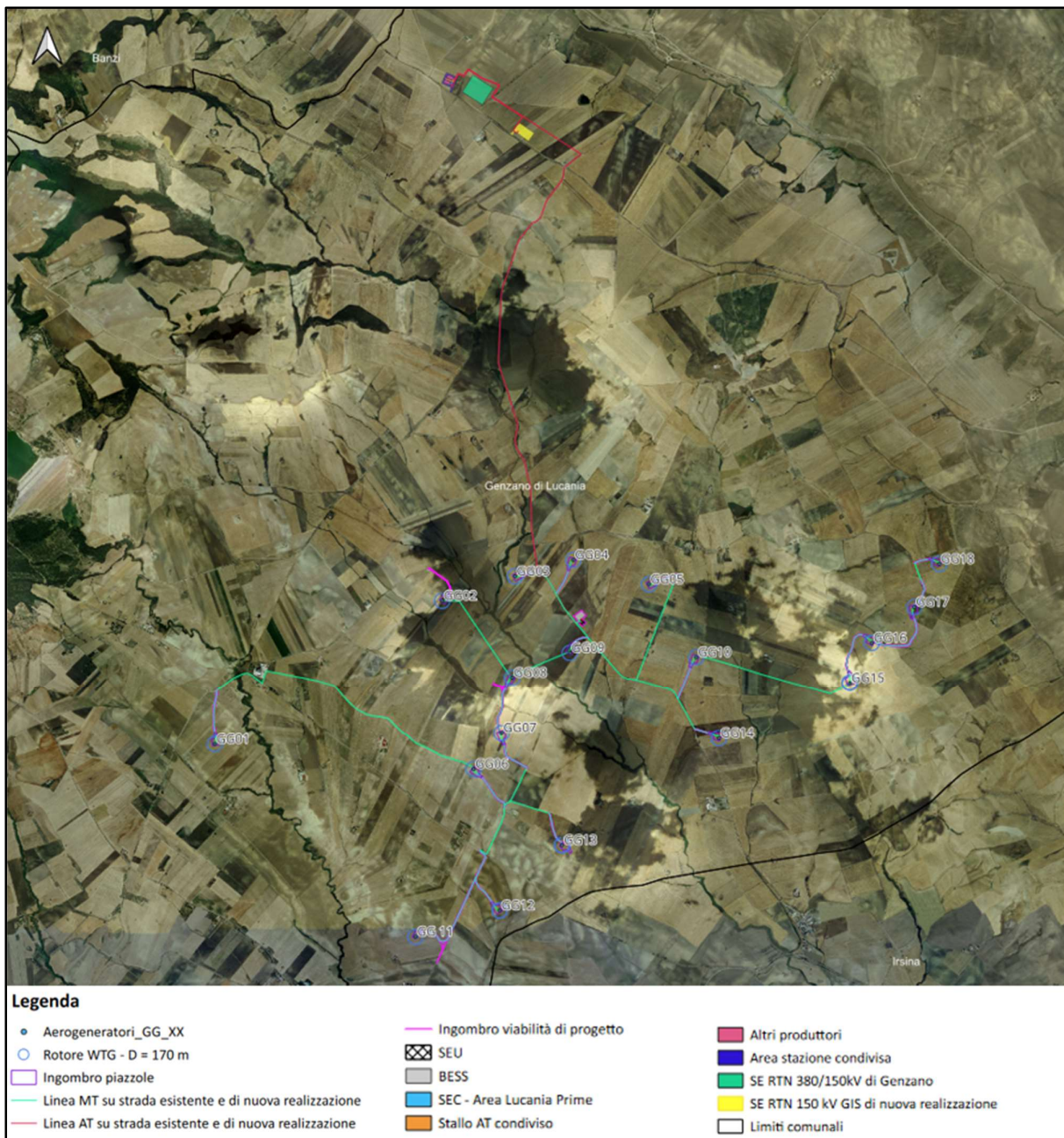
Figura 6.4: Layout d'impianto su ortofoto
