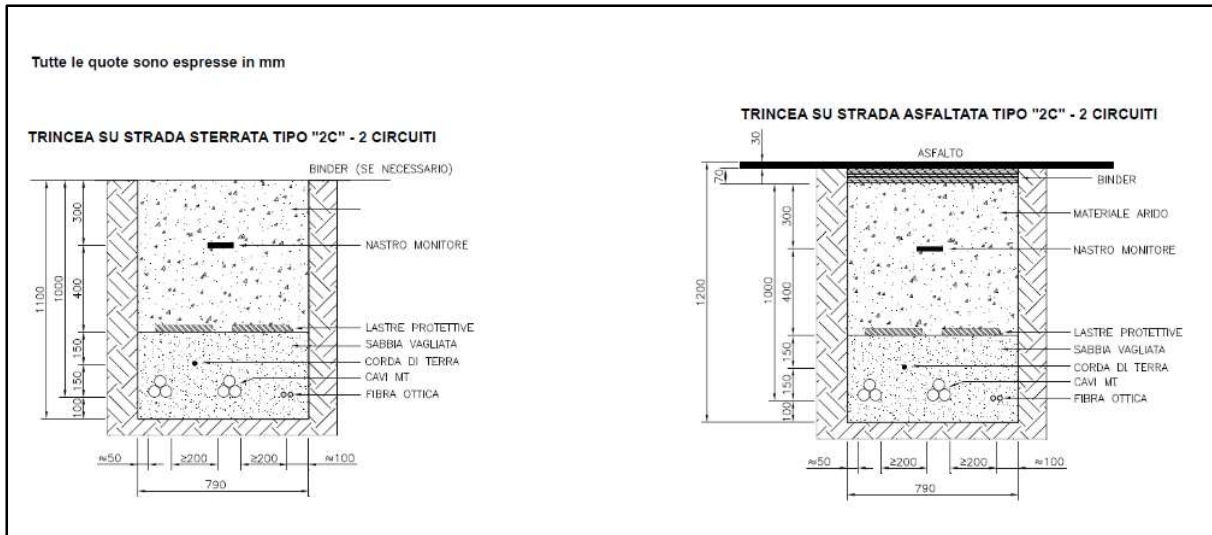
Figura 6.3.4.3: Sezioni tipiche delle trincee cavidotto per due terne di cavi in parallelo su strada sterrata e asfaltata
