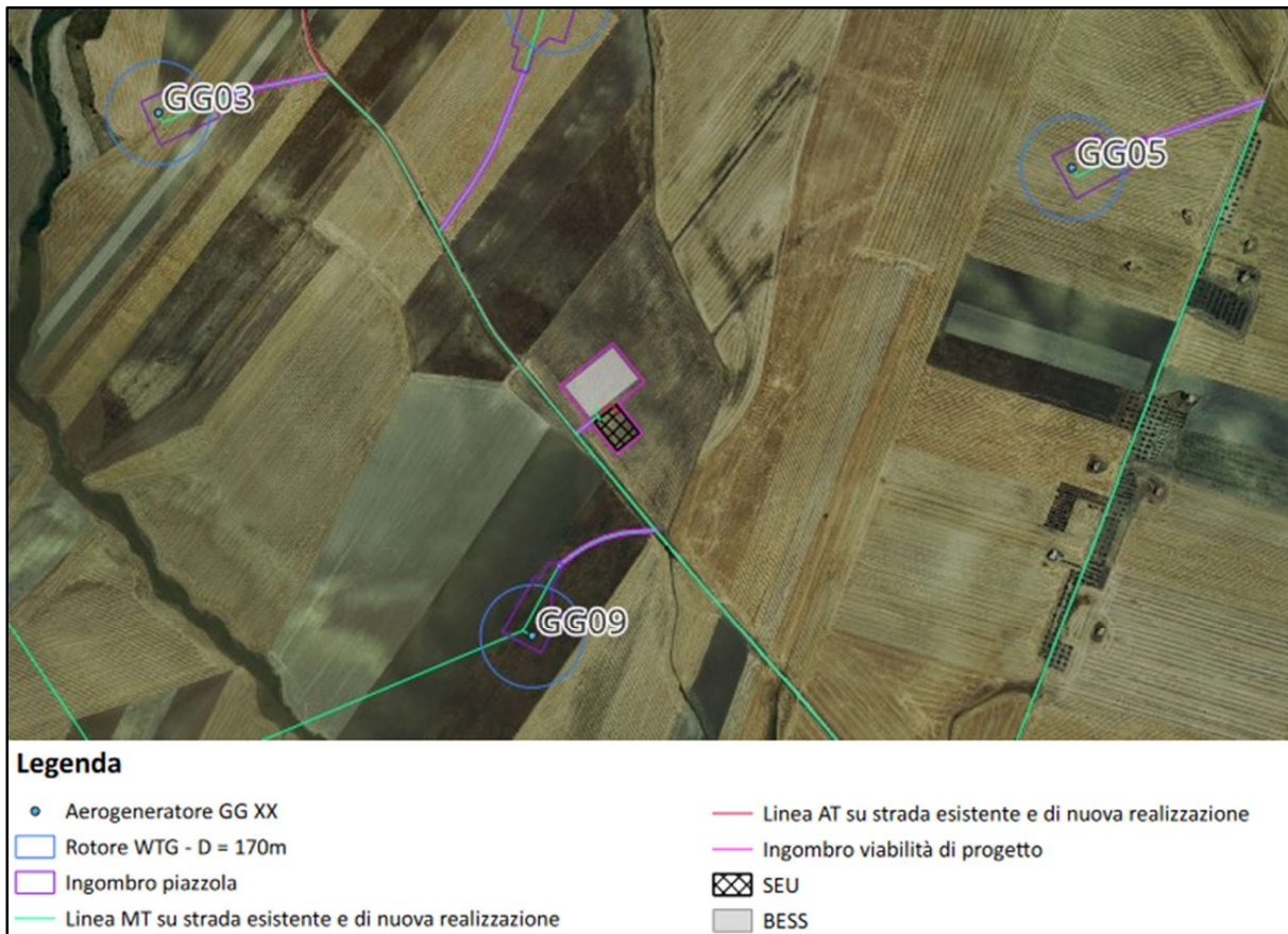
Figura 6.3.3.1: Localizzazione del BESS e della SEU 150/33 kV su ortofoto
