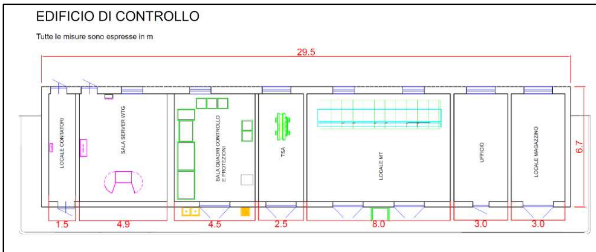
Figura 6.3.2.5: Pianta edificio di controllo SEU 150/33 kV
