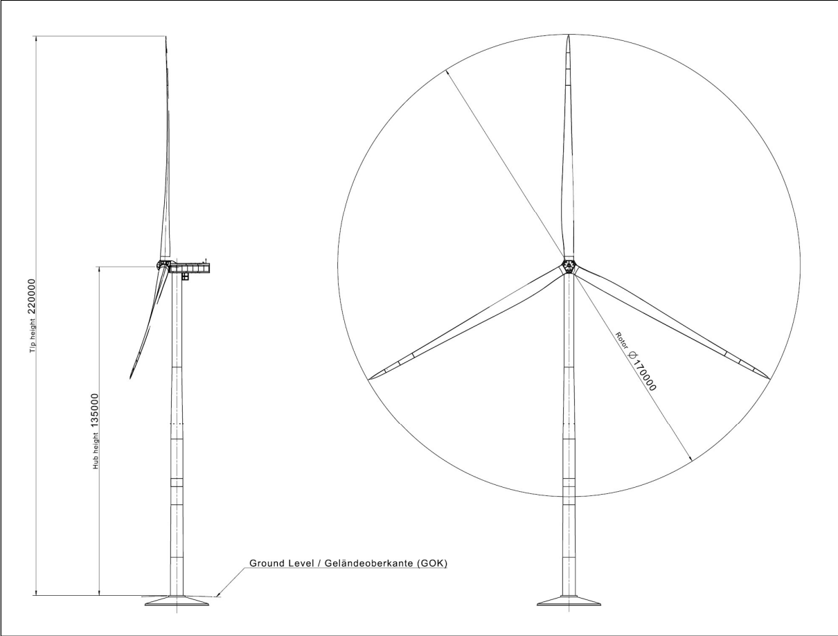
Figura 6.1.1: Profilo aerogeneratore SG170 – 6,2 MWp – HH= 135 m – D=170 m
