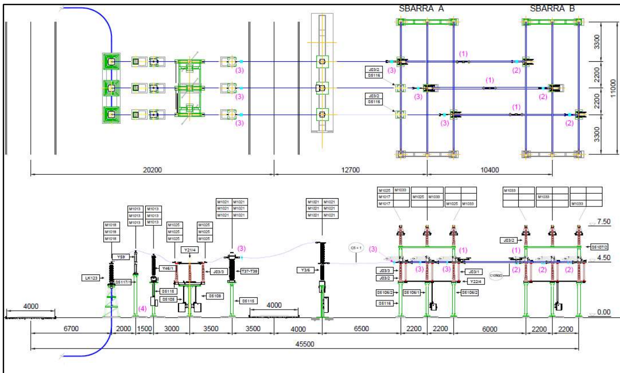
Figura 6.3.7.3: Planimetria e sezione elettromeccanica relativa alle apparecchiature dello stallo 150 kV nella stazione Terna
