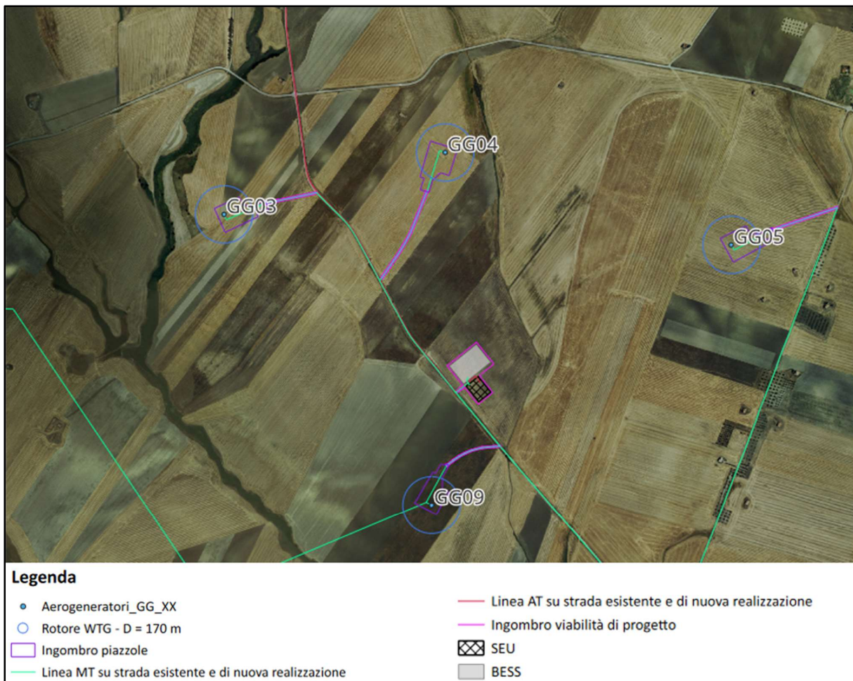
Figura 6.3.2.2: Localizzazione della SEU 150/33 kV e del BESS su ortofoto
