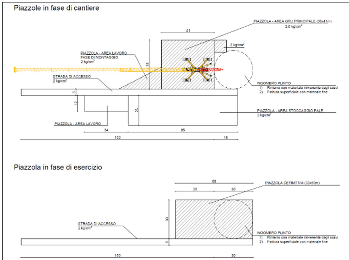
Figura 6.2.2: Planimetria piazzola tipo per le fasi di installazione e di esercizio e manutenzione
