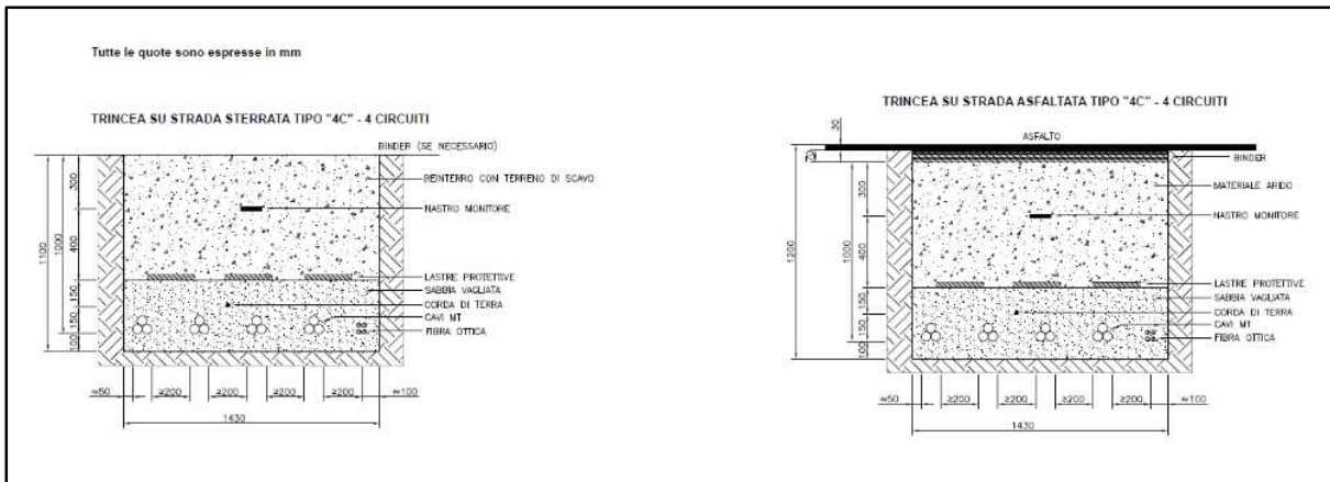
Figura 6.3.4.5: Sezioni tipiche delle trincee cavidotto per quattro terne di cavi in parallelo su strada sterrata e asfaltata
