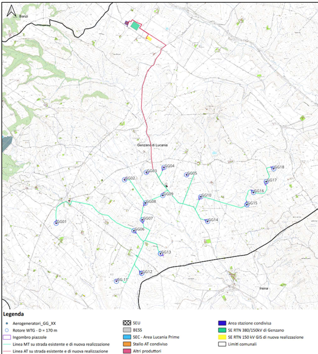
Figura 6.3.2.3: Localizzazione della SEU 150/33 kV, del BESS, della Stazione Elettrica Condivisa (SEC), della SE RTN 380/150 kV di Genzano e della SE GIS di nuova realizzazione (ampliamento della SE RTN) su CTR
