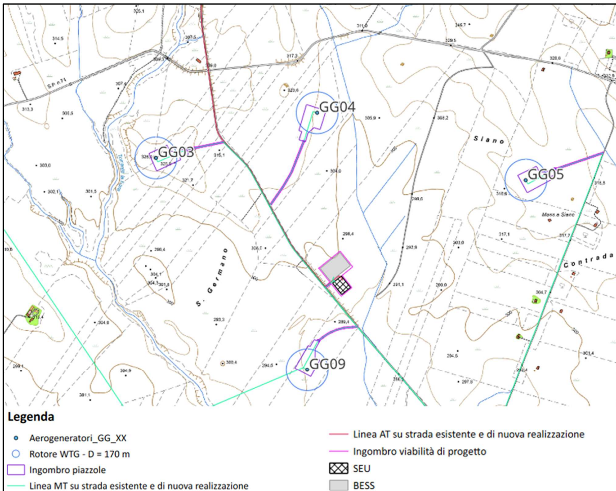
Figura 6.3.2.1: Localizzazione della SEU 150/33 kV e del BESS su CTR
