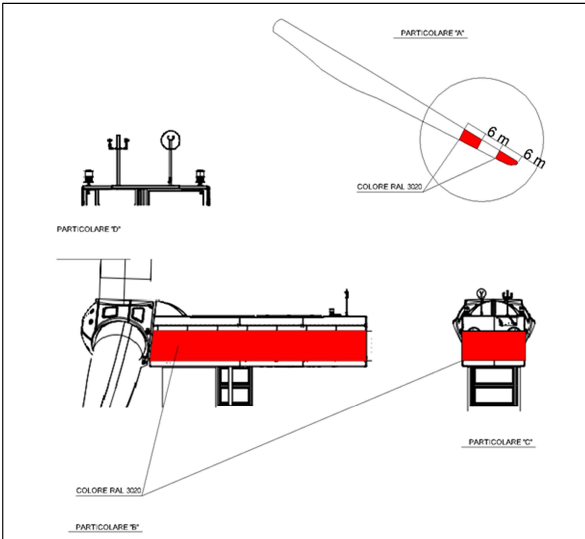
Figura 6.1.2: Particolari aerogeneratore SG170 – 6,2 MWp di cui alla Figura 2.1.1
