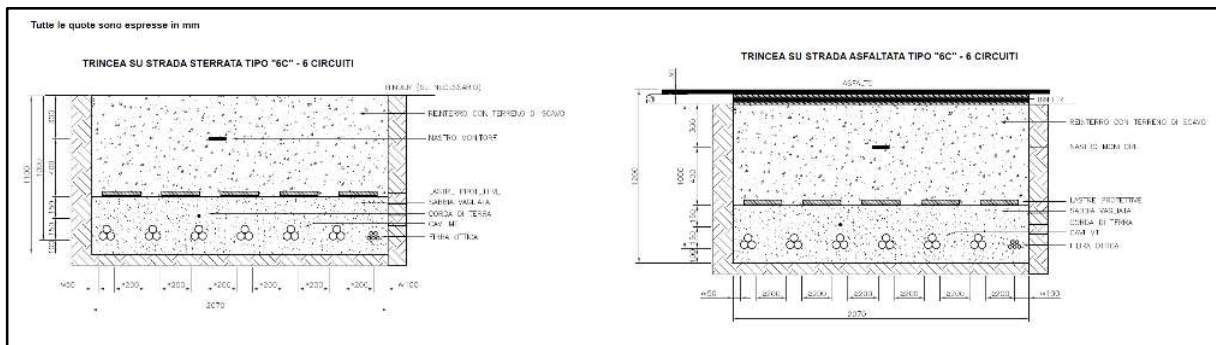
Figura 6.3.4.7: Sezioni tipiche delle trincee cavidotto per sei terne di cavi in parallelo su strada sterrata e asfaltata
