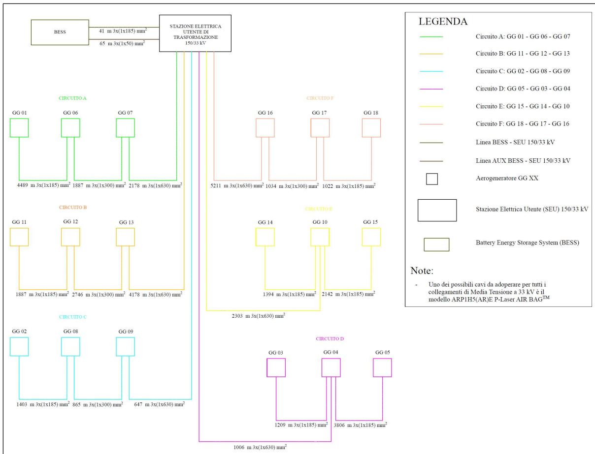
Figura 6.3.4.1: Schema a blocchi del Parco Eolico Genzano
