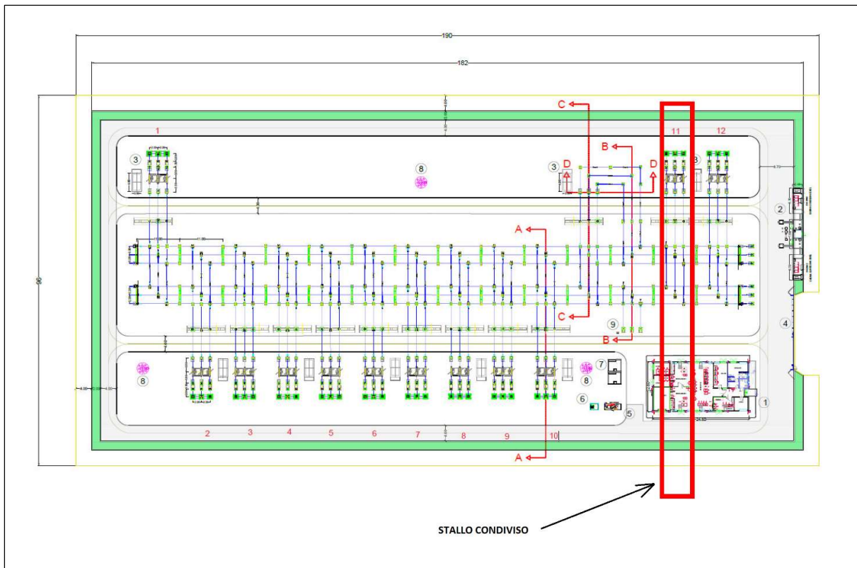
Figura 6.3.7.2: Planimetria elettromeccanica ed evidenziazione dello stallo riservato all'impianto in progetto e condiviso con altri produttori
