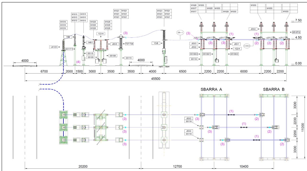
Figura 11.3: Planimetria e sezione elettromeccanica relativa alle apparecchiature dello stallo 150 kV nella stazione Terna
