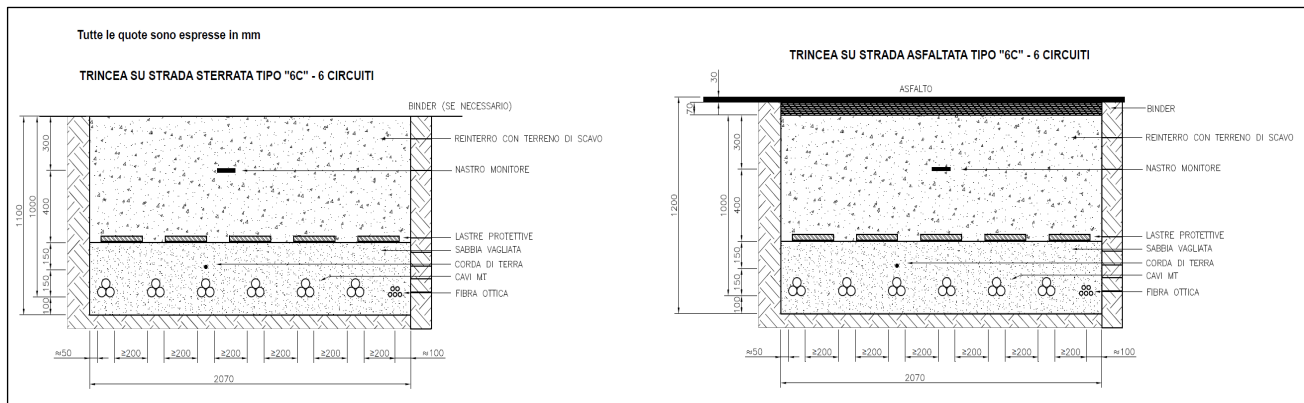
Figura 5.3.6: Sezioni tipiche delle trincee di cavidotto per sei terne di cavi in parallelo su strada sterrata e asfaltata
