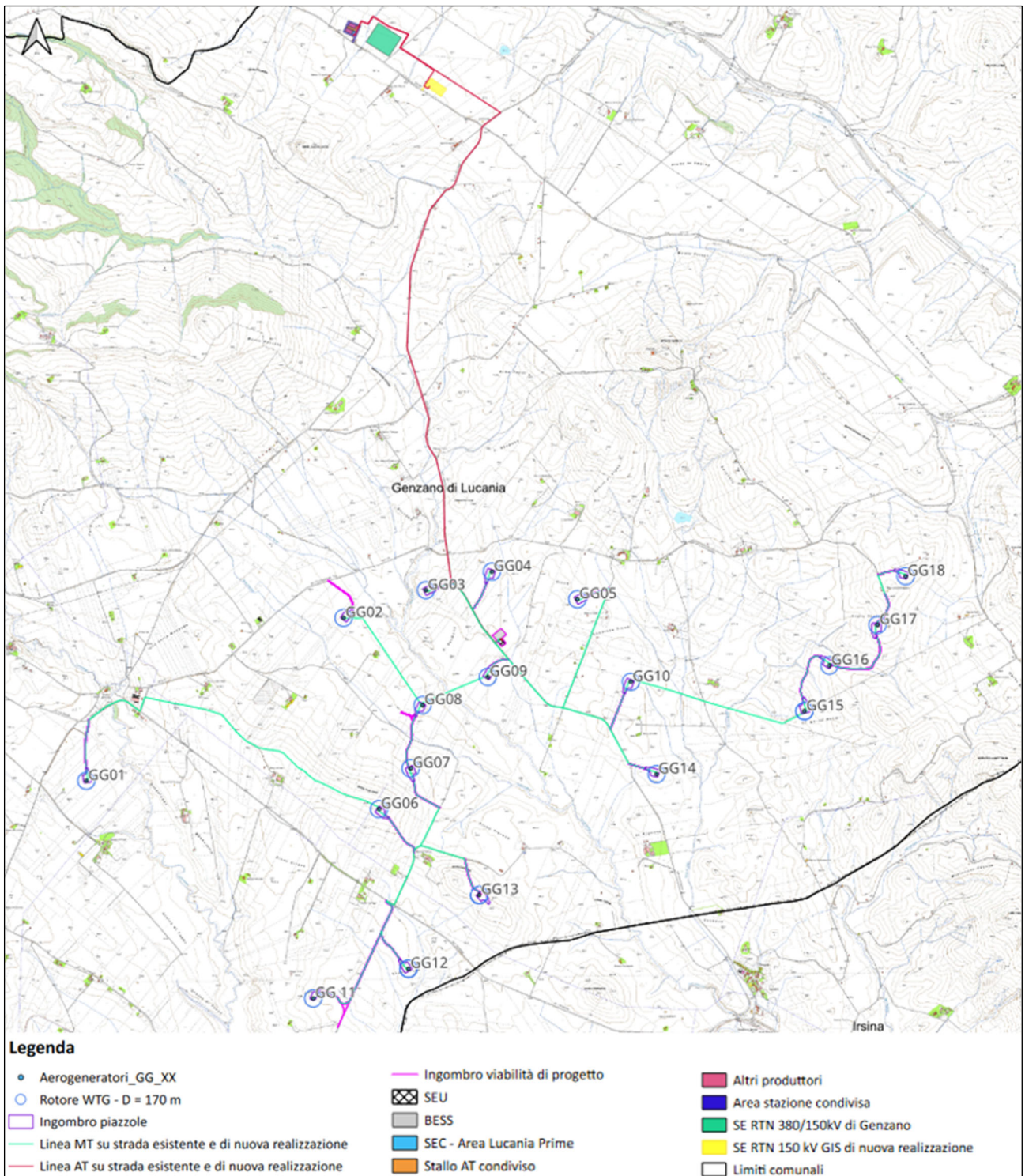
Figura 2.2: Layout d'impianto con viabilità di progetto su CTR
