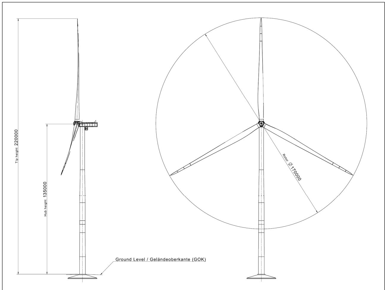
Figura 2.1: Profilo aerogeneratore SG170 – 6,2 MWp – HH= 135 m – D=170 m
