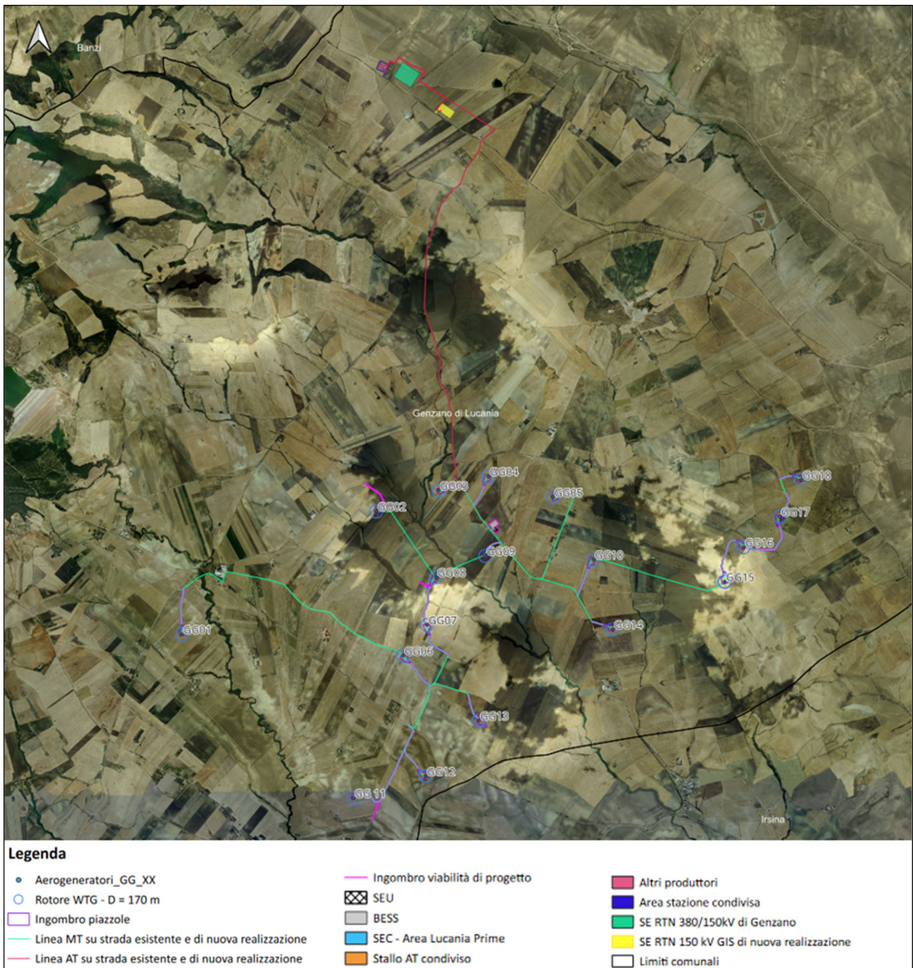
Figura 2.3: Layout dell'impianto su ortofoto
