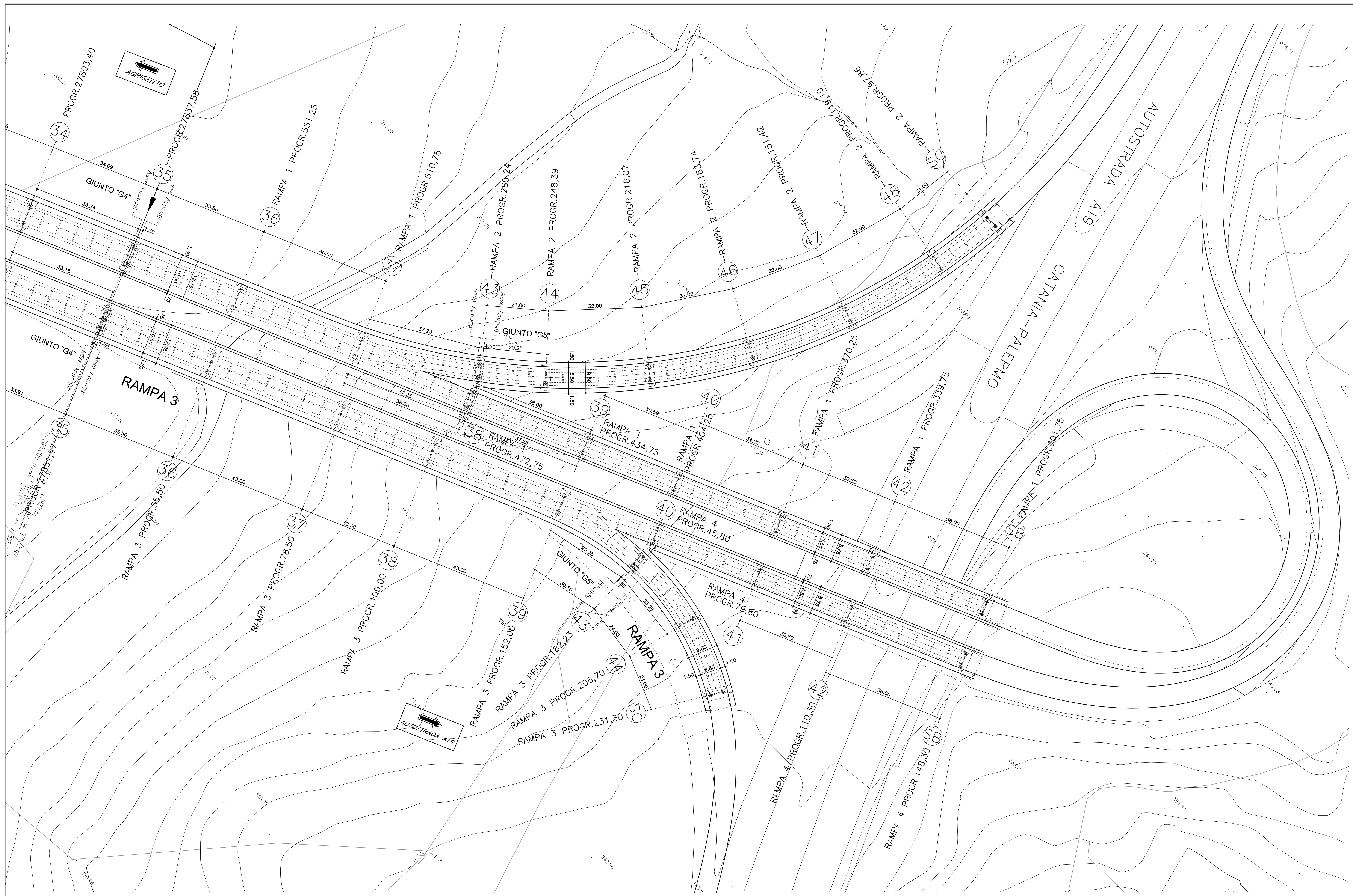
PIANTA IMPALCATO SCALA 1 : 500
