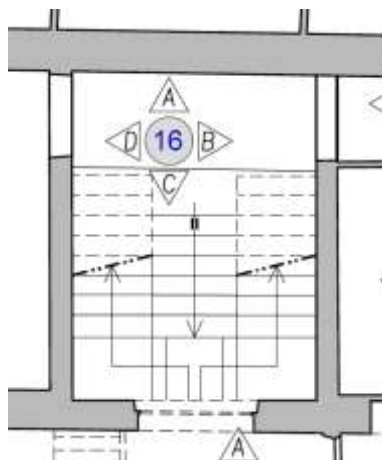
Figura 4-157. PALAZZO PARETO – P1 – Particolare Planimetria Vano 15
