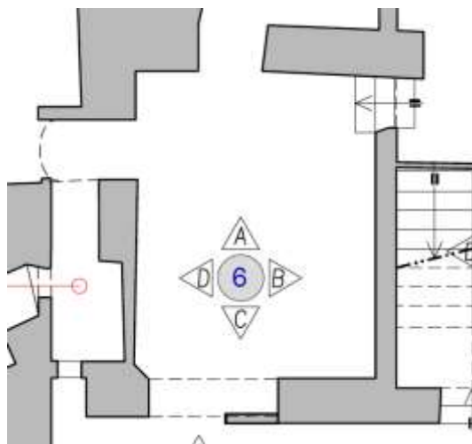
Figura 4-25. PALAZZO PARETO – PT – Particolare Planimetria Vano 6
