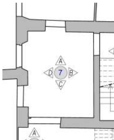
Figura 4-109. PALAZZO PARETO – P1 – Particolare Planimetria Vano 7
