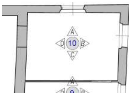
Figura 4-125. PALAZZO PARETO – P1 – Particolare Planimetria Vano 10
