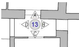
Figura 4-140. PALAZZO PARETO – P1 – Particolare Planimetria Vano 13
