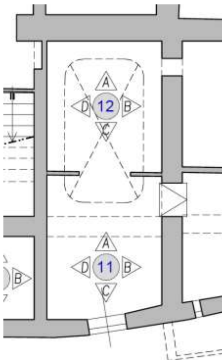
Figura 4-59. PALAZZO PARETO – PT – Particolare Planimetria Vano 12
