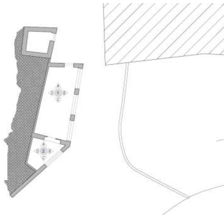
Figura 3-4. SERRA E TORRE - Pianta Piano Terra
