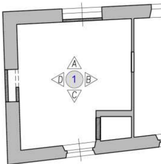
Figura 4-74. PALAZZO PARETO – P1 – Particolare Planimetria Vano 1
