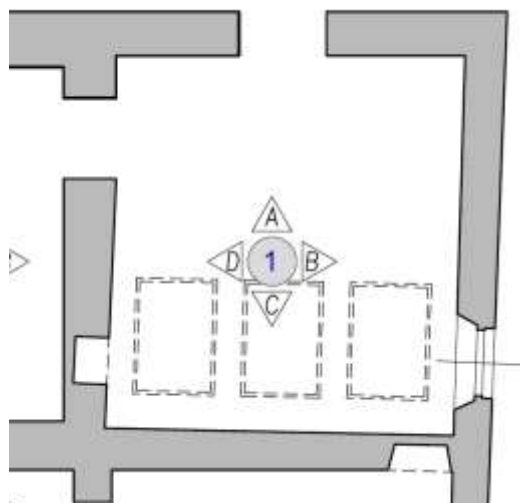
Figura 4-1. PALAZZO PARETO – PT – Particolare Planimetria Vano 1
