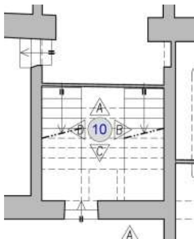
Figura 4-50. PALAZZO PARETO – PT – Particolare Planimetria Vano 10
