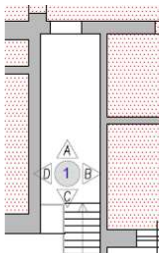
Figura 4-165. PALAZZO PARETO – P2 –Particolare planimetria Vano 1
