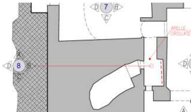
Figura 4-52. PALAZZO PARETO – PT – Particolare Planimetria Vano 8
