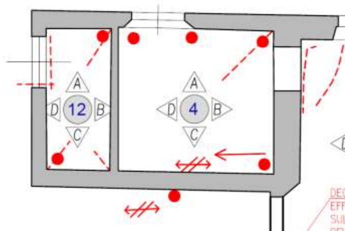
Figura 4-177. PALAZZO PARETO – P1 – Particolare Planimetria Vano 12
