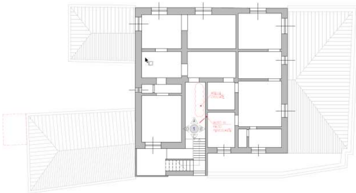
Figura 3-3. PALAZZO PARETO - Pianta Piano Secondo
