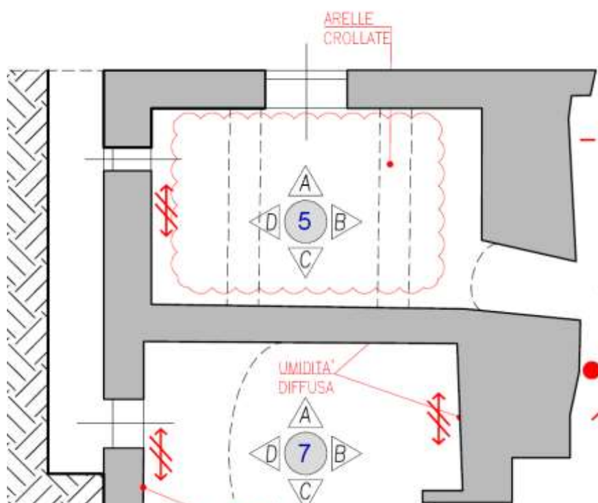
Figura 4-33. PALAZZO PARETO – PT – Particolare Planimetria Vano 5
