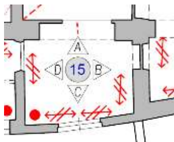
Figura 4-197. PALAZZO PARETO – P1 – Particolare Planimetria Vano 15
