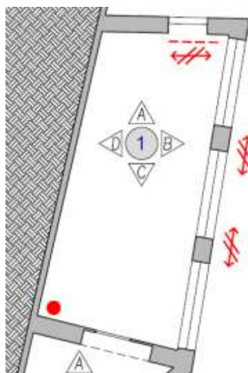
Figura 5-1. SERRA – Particolare planimetria Vano 1
