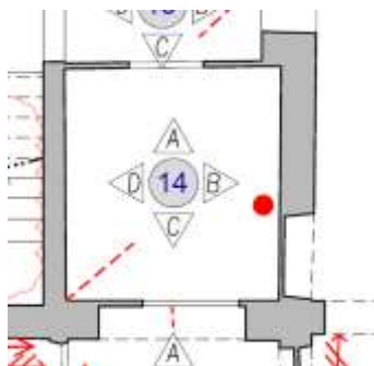
Figura 4-188. PALAZZO PARETO – P1 – Particolare Planimetria Vano 14
