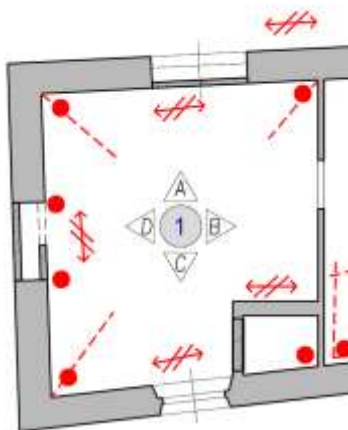
Figura 4-99. PALAZZO PARETO – P1 – Particolare Planimetria Vano 1
