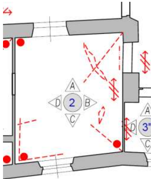
Figura 4-104. PALAZZO PARETO – P1 – Particolare Planimetria Vano 2
