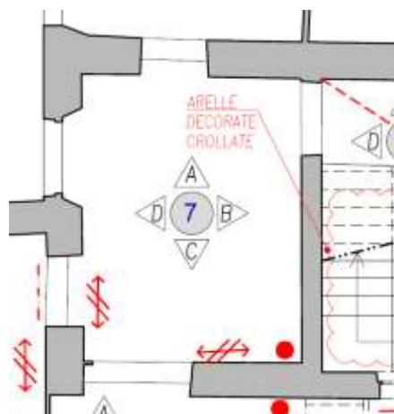
Figura 4-143. PALAZZO PARETO – P1 – Particolare Planimetria Vano 7
