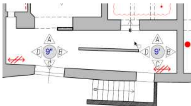
Figura 4-63. PALAZZO PARETO – PT – Particolare Planimetria Vano 9"
