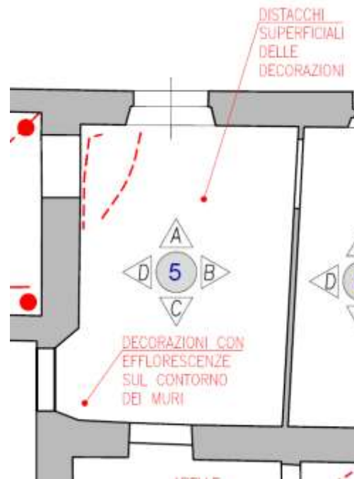
Figura 4-128. PALAZZO PARETO – P1 – Particolare Planimetria Vano 5
