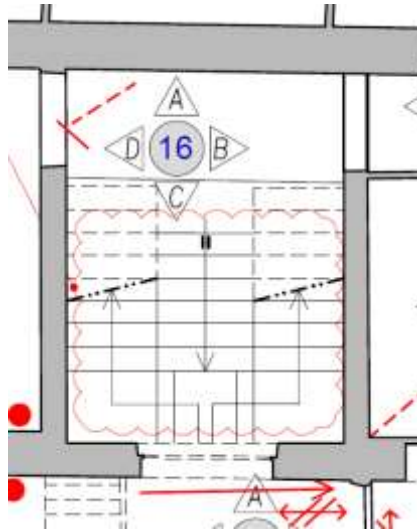
Figura 4-204. PALAZZO PARETO – P1 – Particolare Planimetria Vano 15
