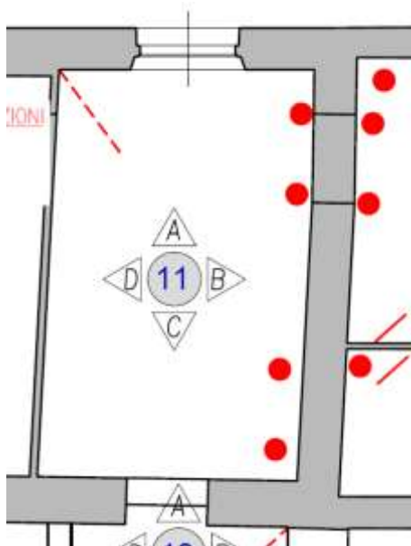
Figura 4-167. PALAZZO PARETO – P1 – Particolare Planimetria Vano 11
