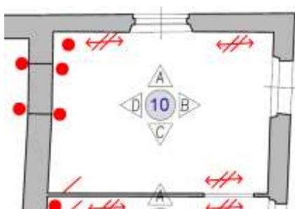
Figura 4-162. PALAZZO PARETO – P1 – Particolare Planimetria Vano 10
