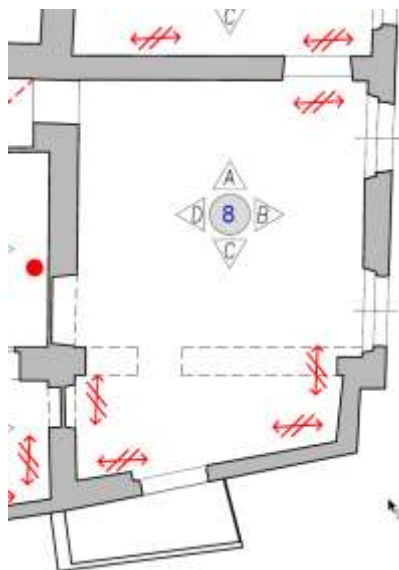
Figura 4-149. PALAZZO PARETO – P1 – Particolare Planimetria Vano 8
