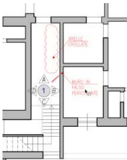
Figura 4-213. PALAZZO PARETO – P2 –Particolare planimetria Vano 1
