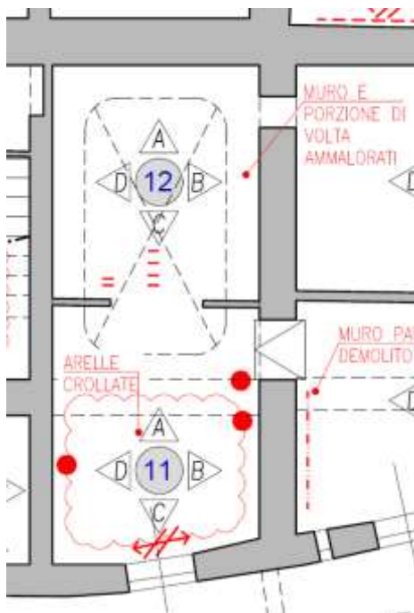
Figura 4-72. PALAZZO PARETO – PT – Particolare Planimetria Vano 11
