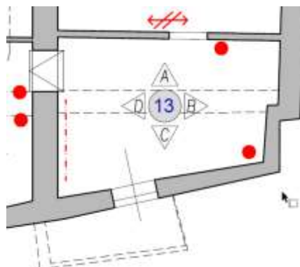
Figura 4-89. PALAZZO PARETO – PT – Particolare Planimetria Vano 13
