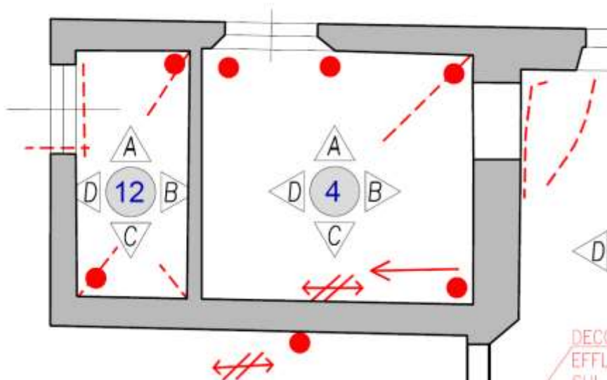
Figura 4-121. PALAZZO PARETO – P1 – Particolare Planimetria Vano 4
