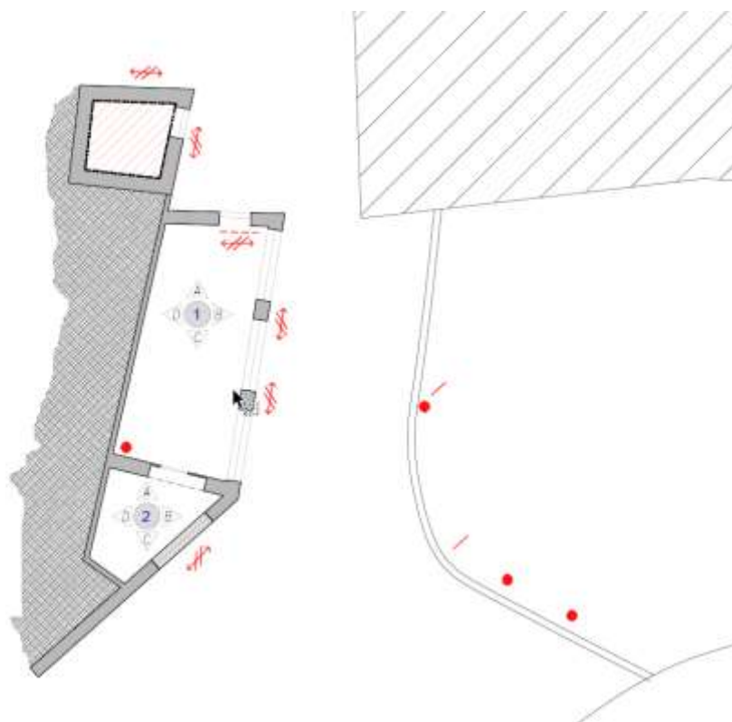
Figura 3-4. SERRA E TORRE - Pianta Piano Terra
