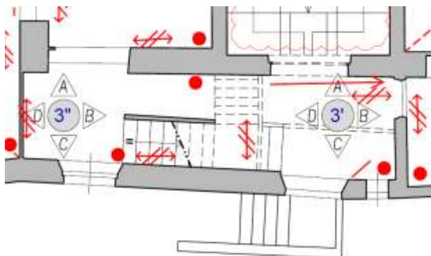
Figura 4-116. PALAZZO PARETO – P1 – Particolare Planimetria Vano 3"
