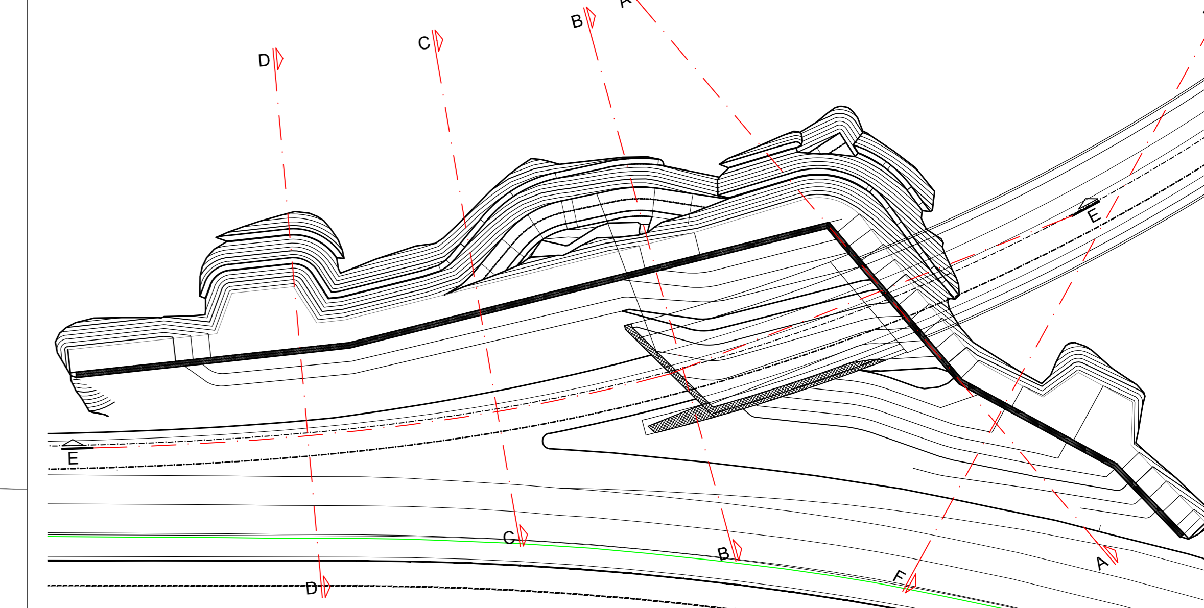
PLANIMETRIA SCALA 1:500
