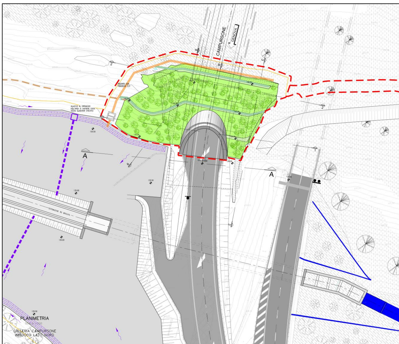
Figura 9 – Planimetria finale Imbocco Campursone Sud (fonte: elaborato 110721-LL1B-PES6-G21-GF21S-SSF00-D-AUA8415-1)
