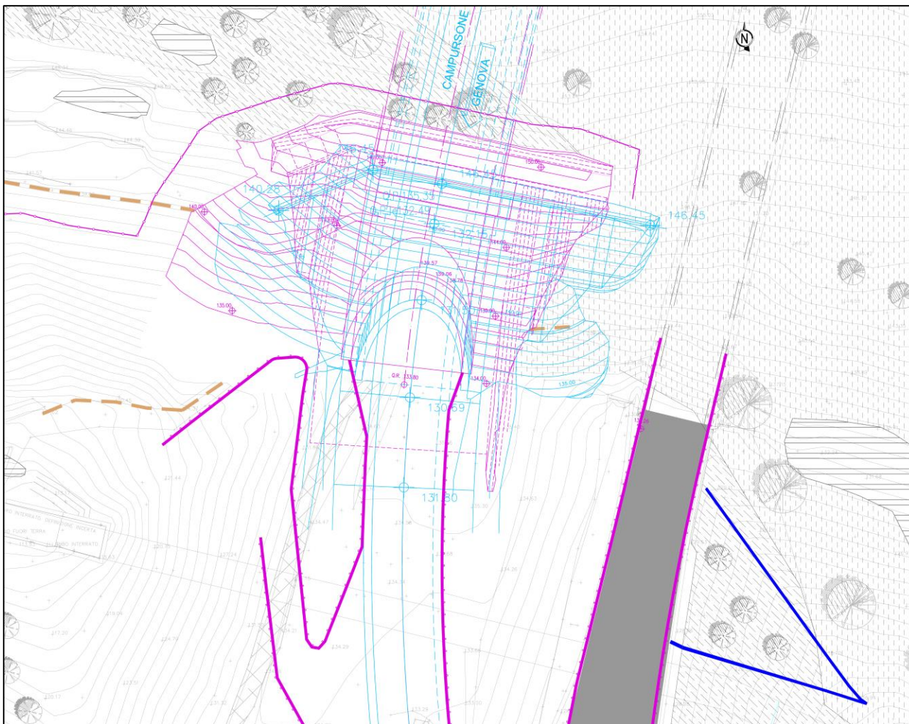
Figura 8 – estratto tavola 110721-LL1B-PE-S6-G21-GP21S-PAE00-D-AUA8403-2 (Progetto Esecutivo in magenta - Progetto Definitivo in ciano)
