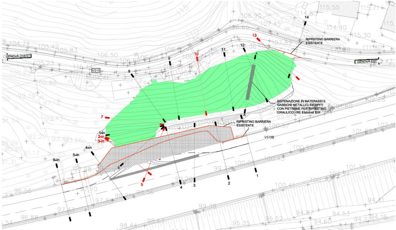
Figura 4-1. Planimetria VS18B con indicate le linee di sezione di riferimento
