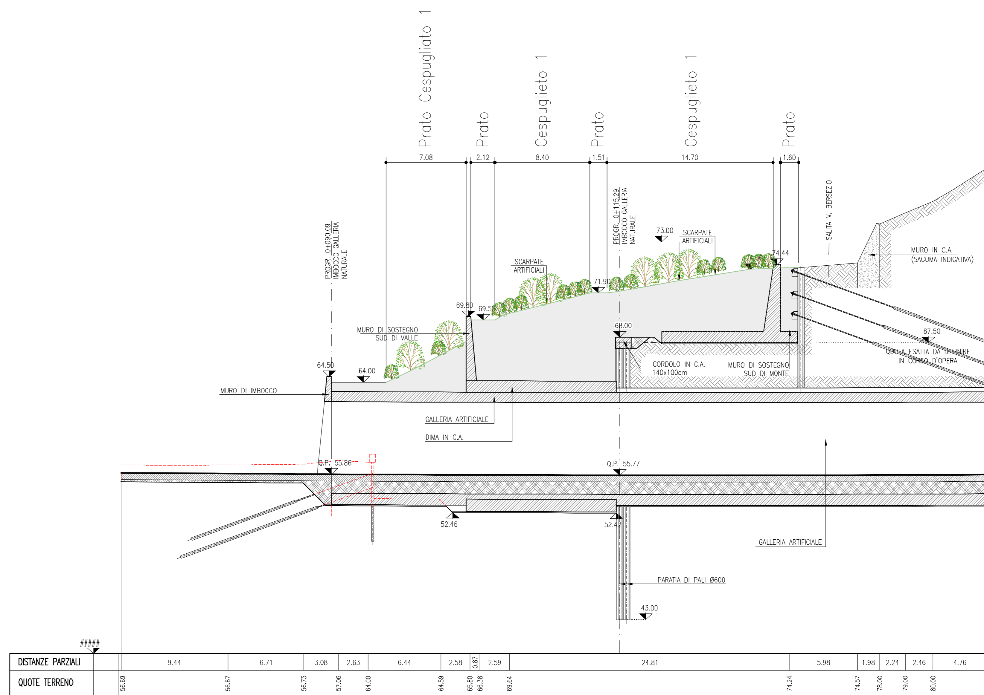
SEZIONE IN ASSE GALLERIA MORO 2 1:200
