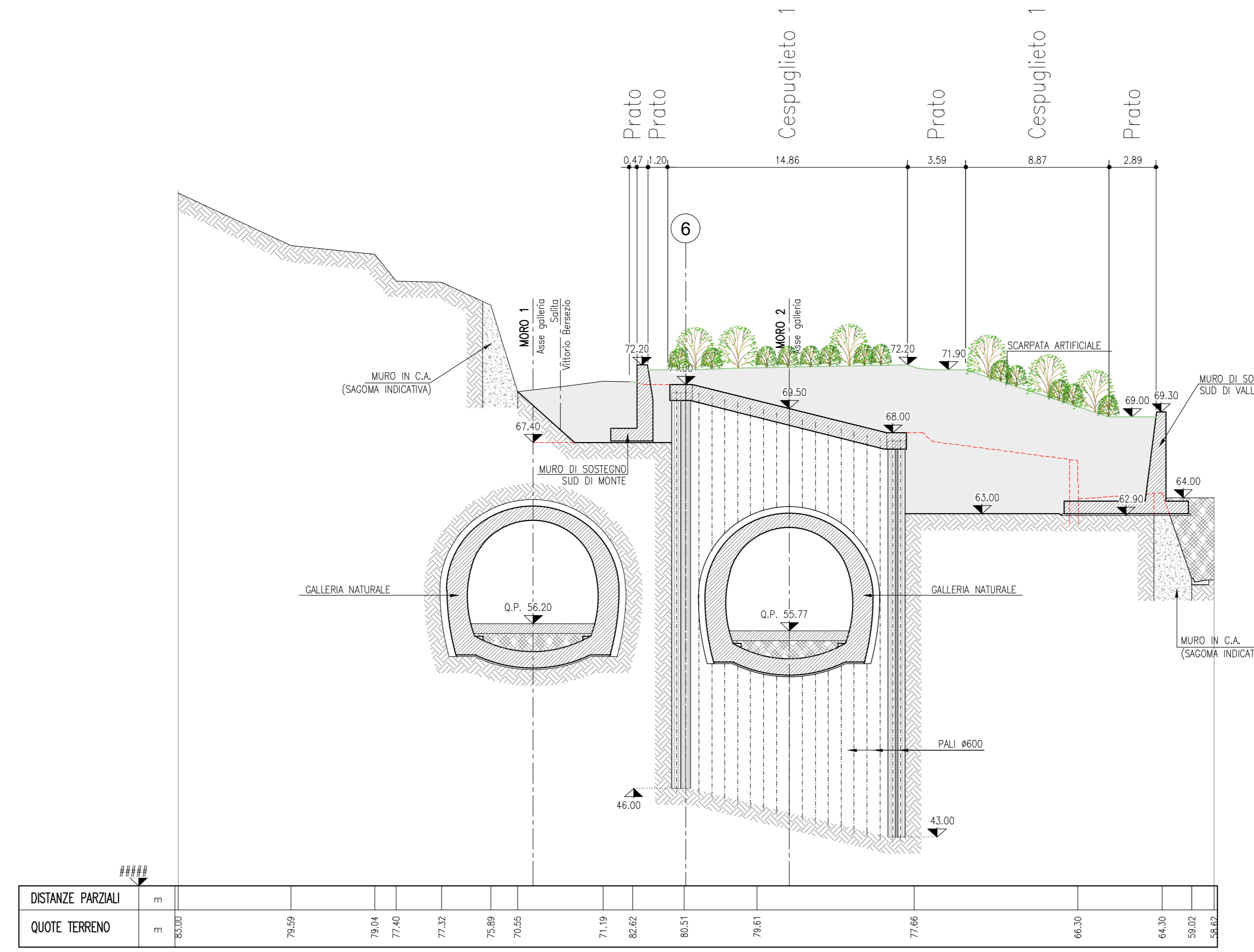
SEZIONE 5-5 1:200
