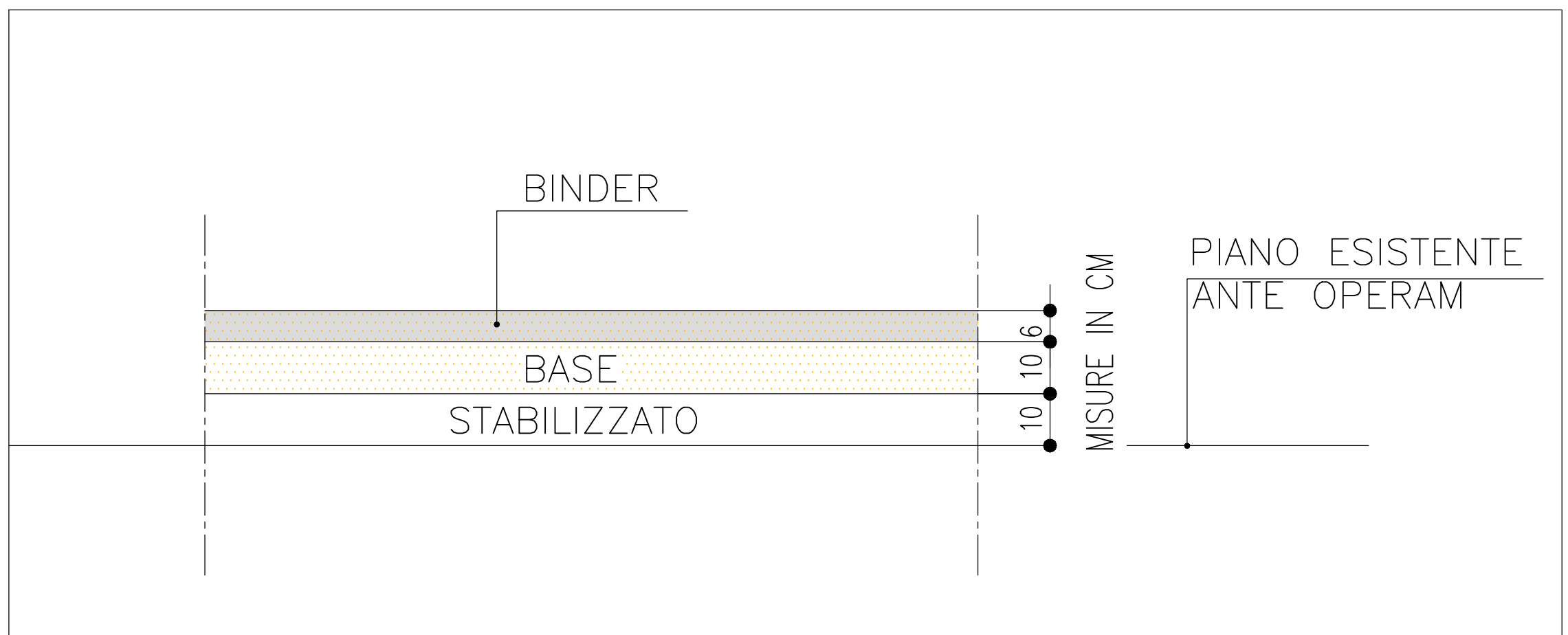
PARTICOLARE PAVIMENTAZIONE 1:20
