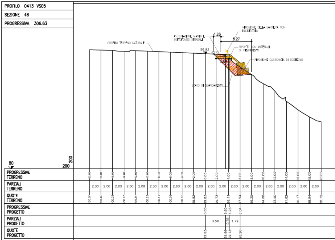
Figura 4-8. Sezione 48
