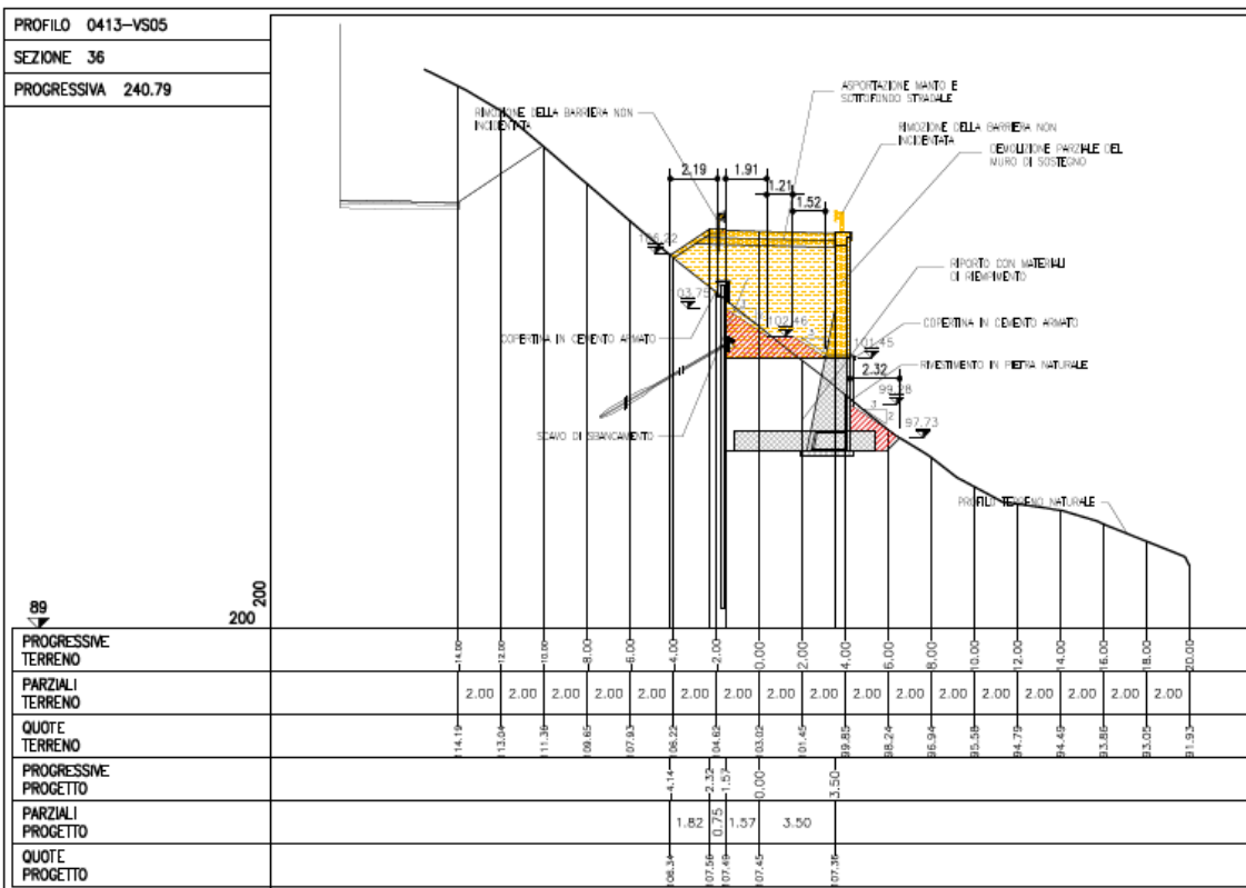
Figura 4-5. Sezione 36
