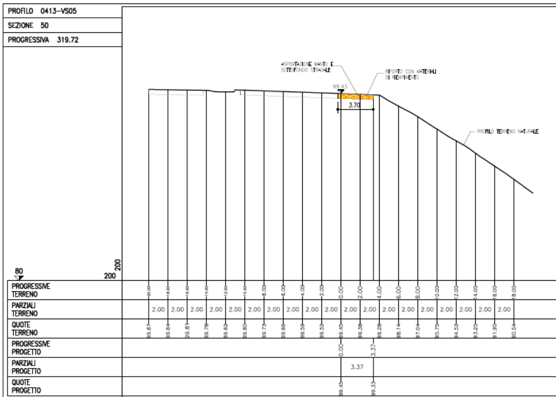
Figura 4-9. Sezione 50
