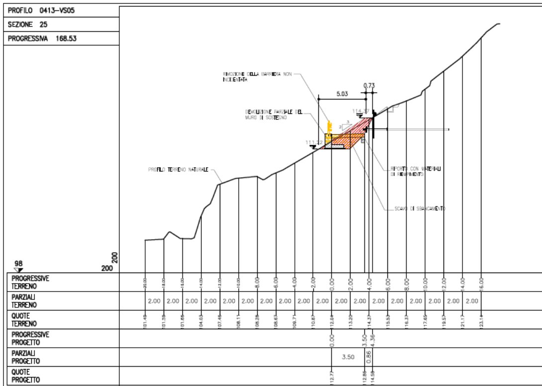
Figura 4-3. Sezione 25
