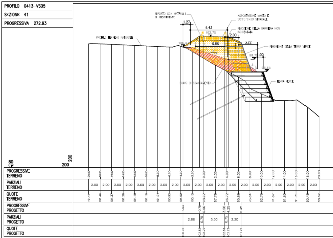
Figura 4-6. Sezione 41
