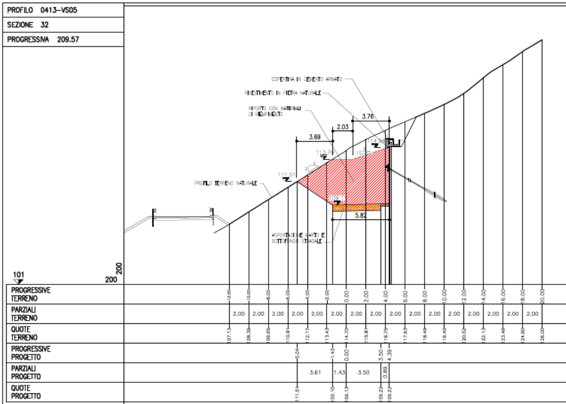
Figura 4-4. Sezione 32
