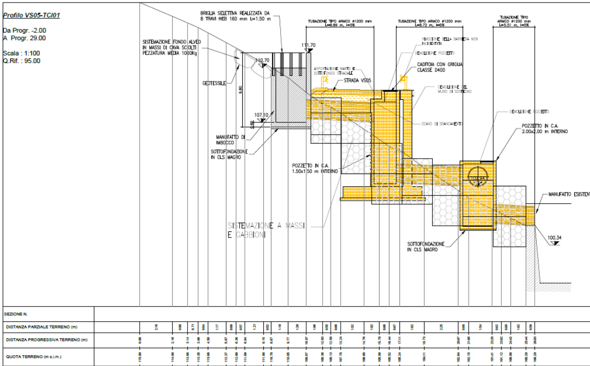
Figura 4-10. Sezione sistemazione tombino
