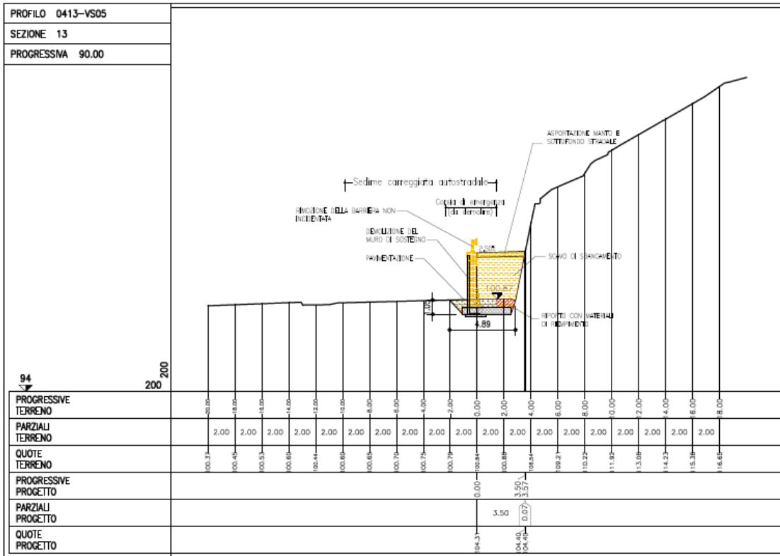
Figura 4-2. Sezione 13
