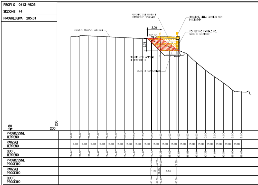
Figura 4-7. Sezione 44
