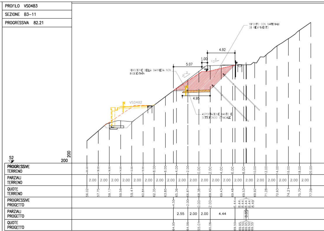
Figura 4-19. Sezione B3-11
