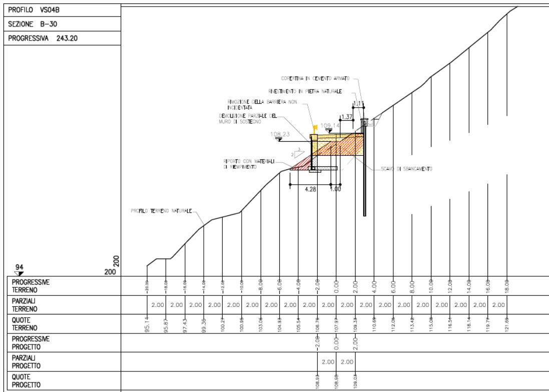
Figura 4-6. Sezione B-30
