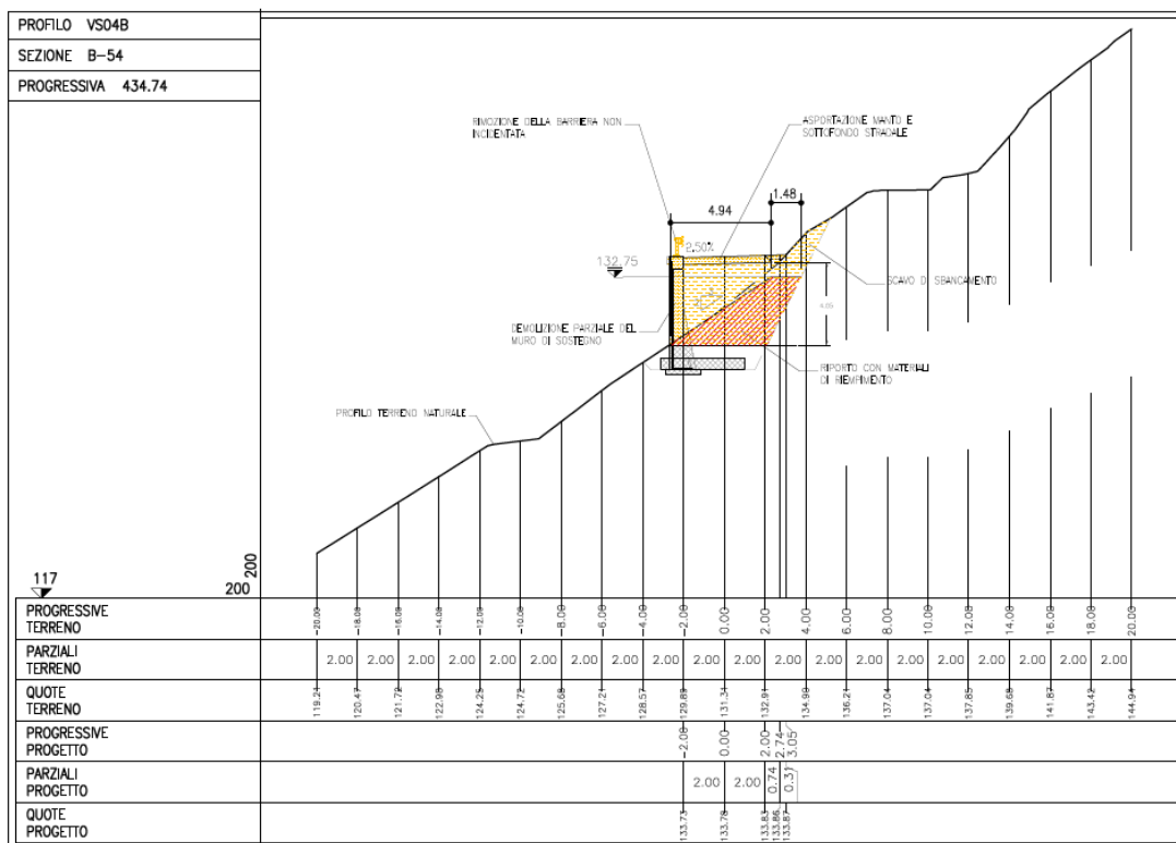
Figura 4-9. Sezione B-54
