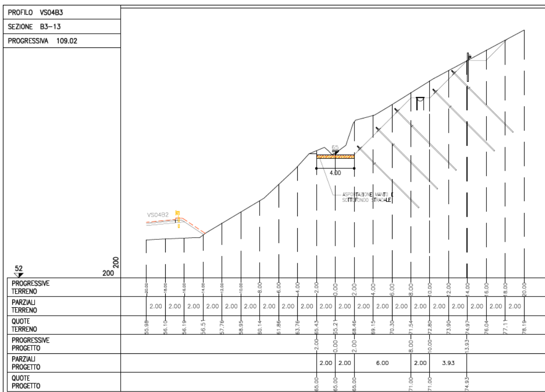
Figura 4-20. Sezione B3-13
