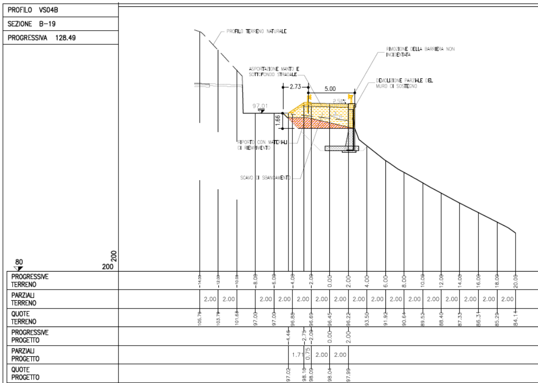
Figura 4-3. Sezione B-19
