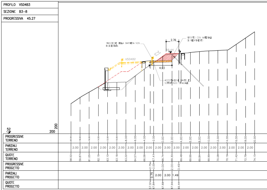
Figura 4-18. Sezione B3-8
