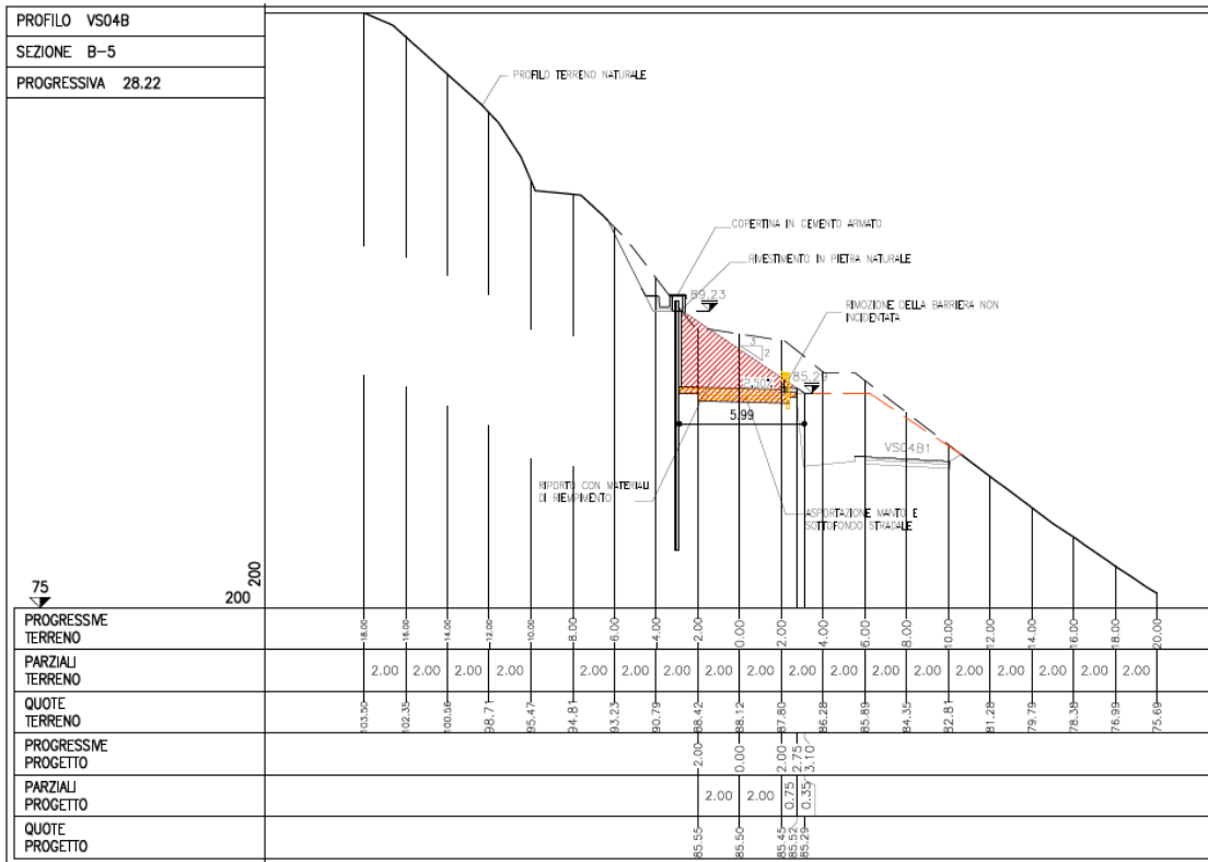
Figura 4-2. Sezione B-5
