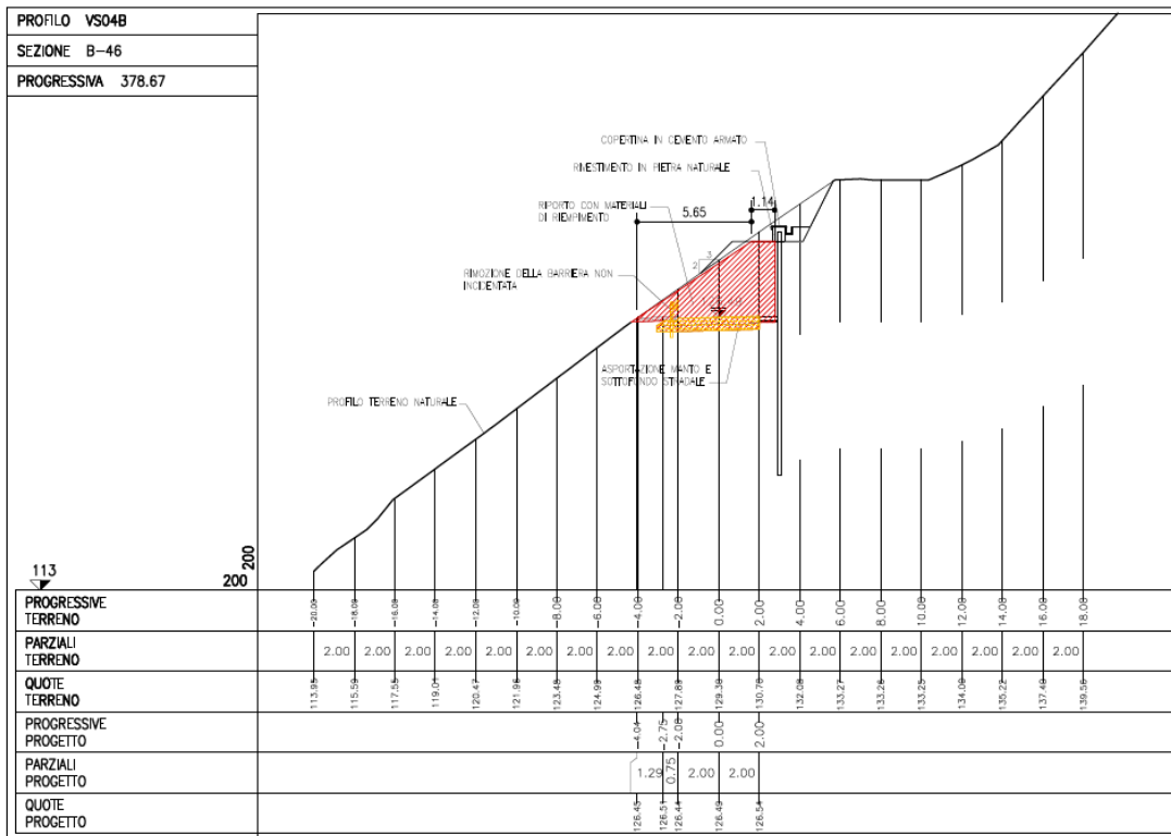
Figura 4-8. Sezione B-46
