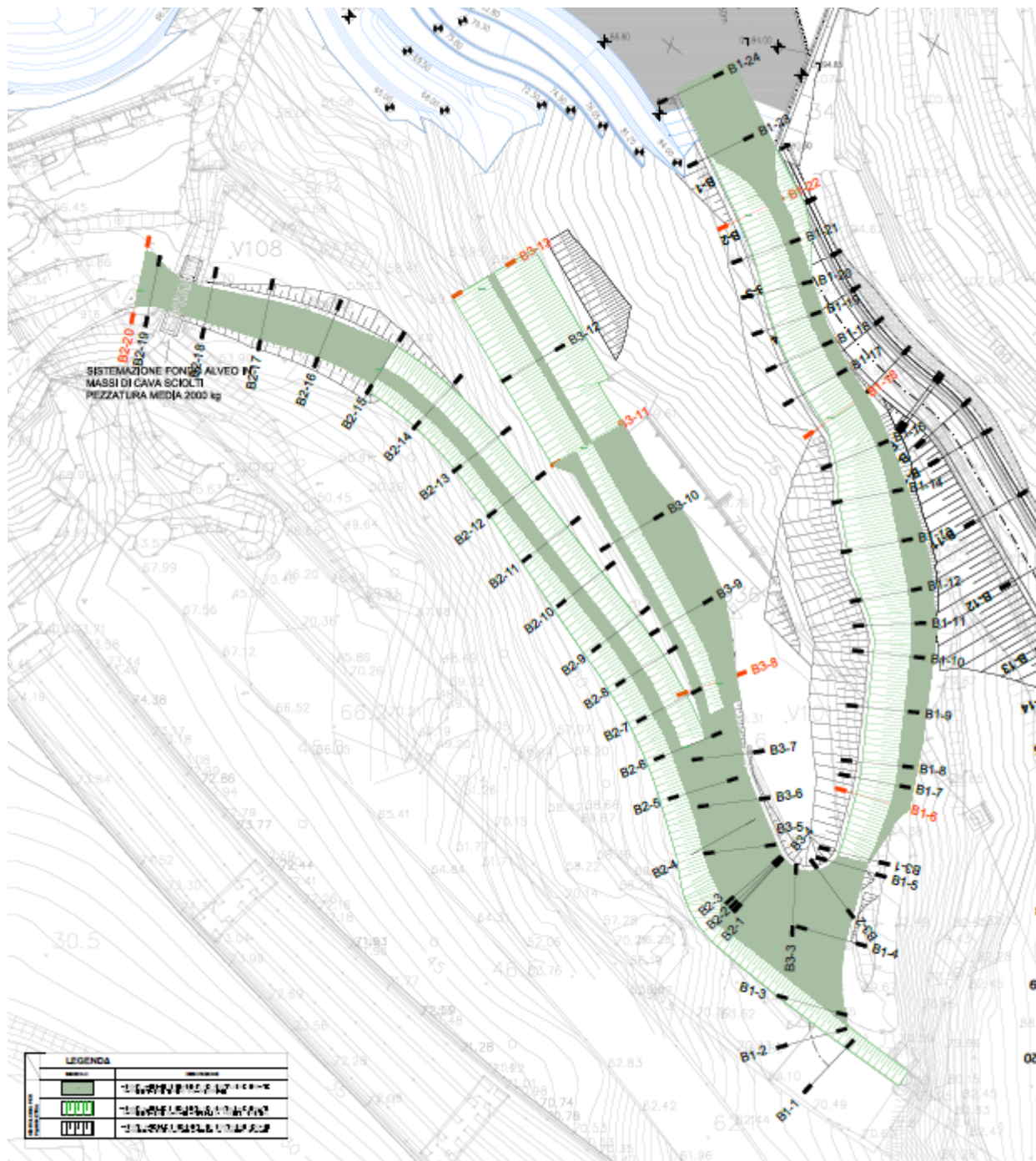
Figura 4-11. Planimetria VS04B1-B2-B3 con indicate le linee di sezione di riferimento
