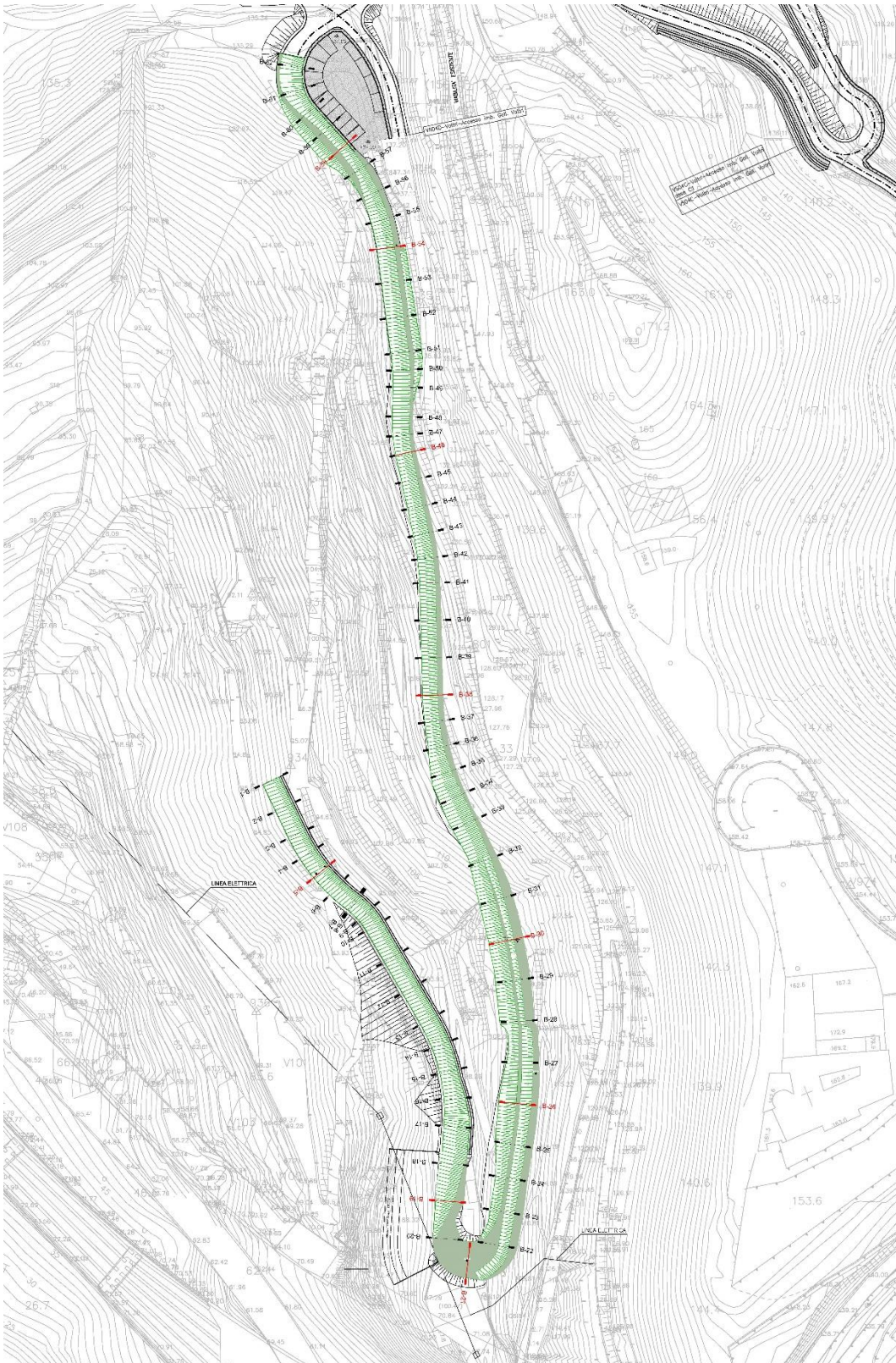
Figura 4-1. Planimetria VS04B con indicate le linee di sezione di riferimento
