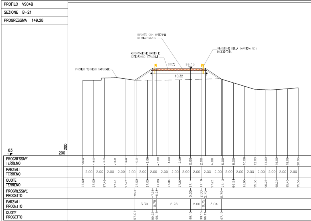
Figura 4-4. Sezione B-21
