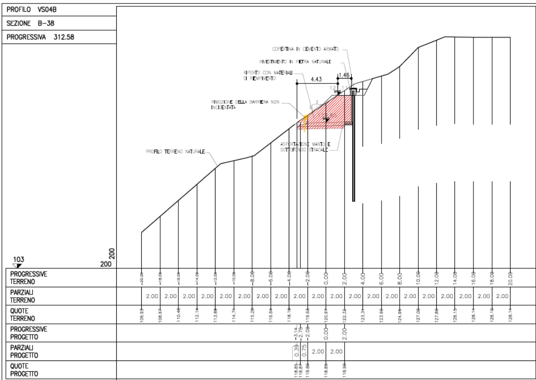
Figura 4-7. Sezione B-38
