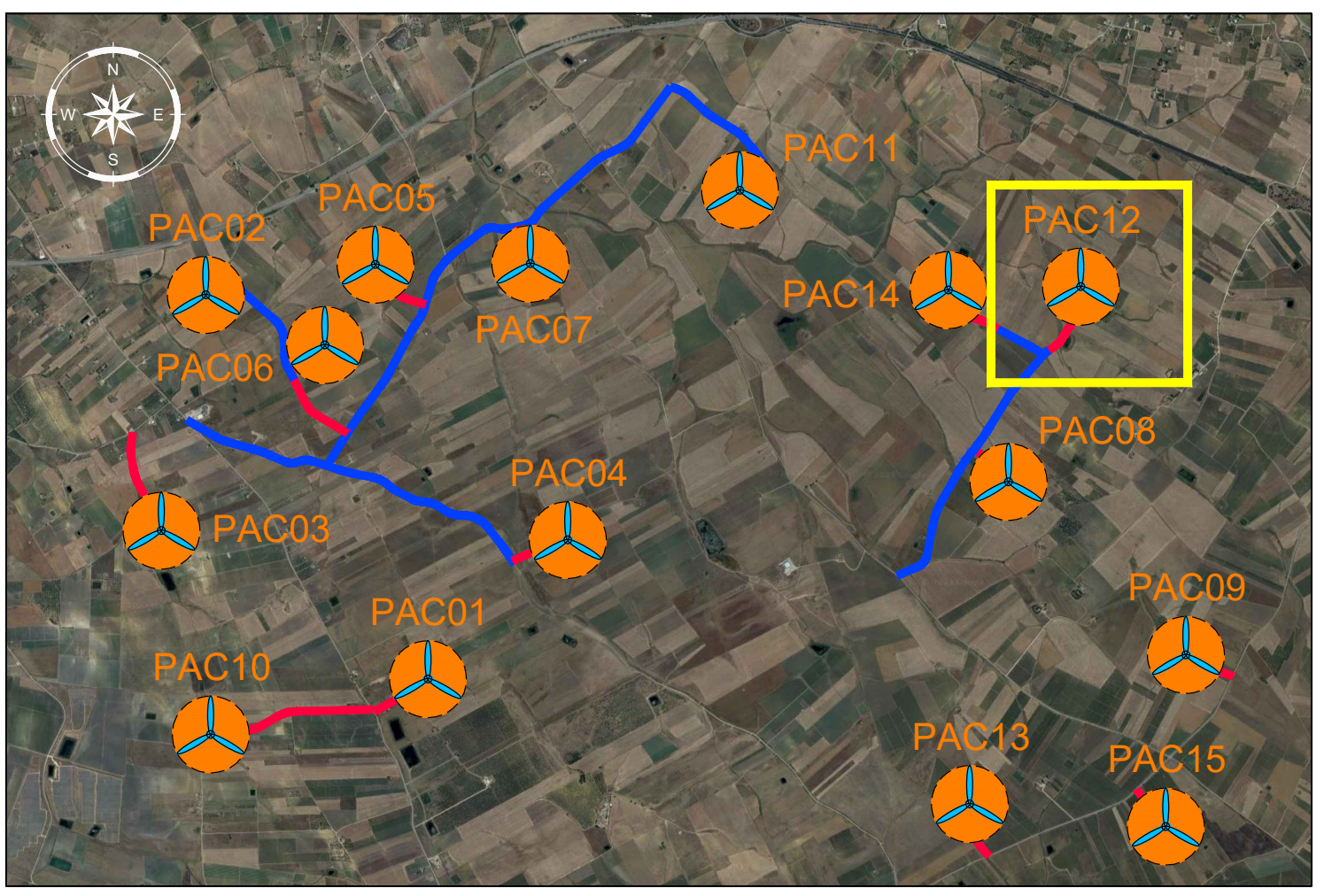
LEGENDA PIANTA CHIAVE ● PAZZOLA CON ROTORE EOLICO — PISTA DI ACCESSO ALLA PAZZOLA — VIABILITA' ESISTENTE DA ADEGUIARE
