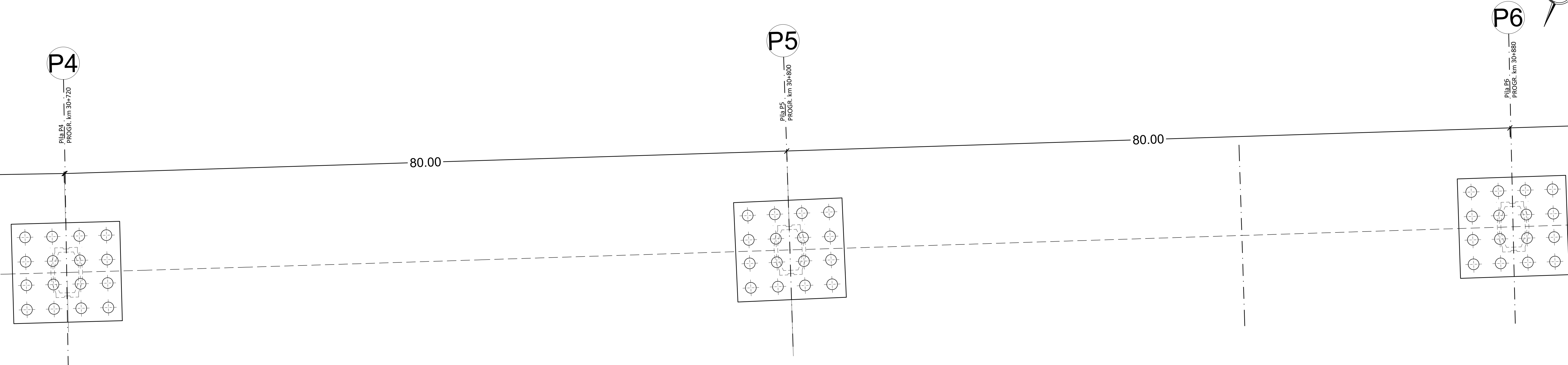
PIANTA OPERA FINITA (STRALCIO 3) SCALA 1:200
