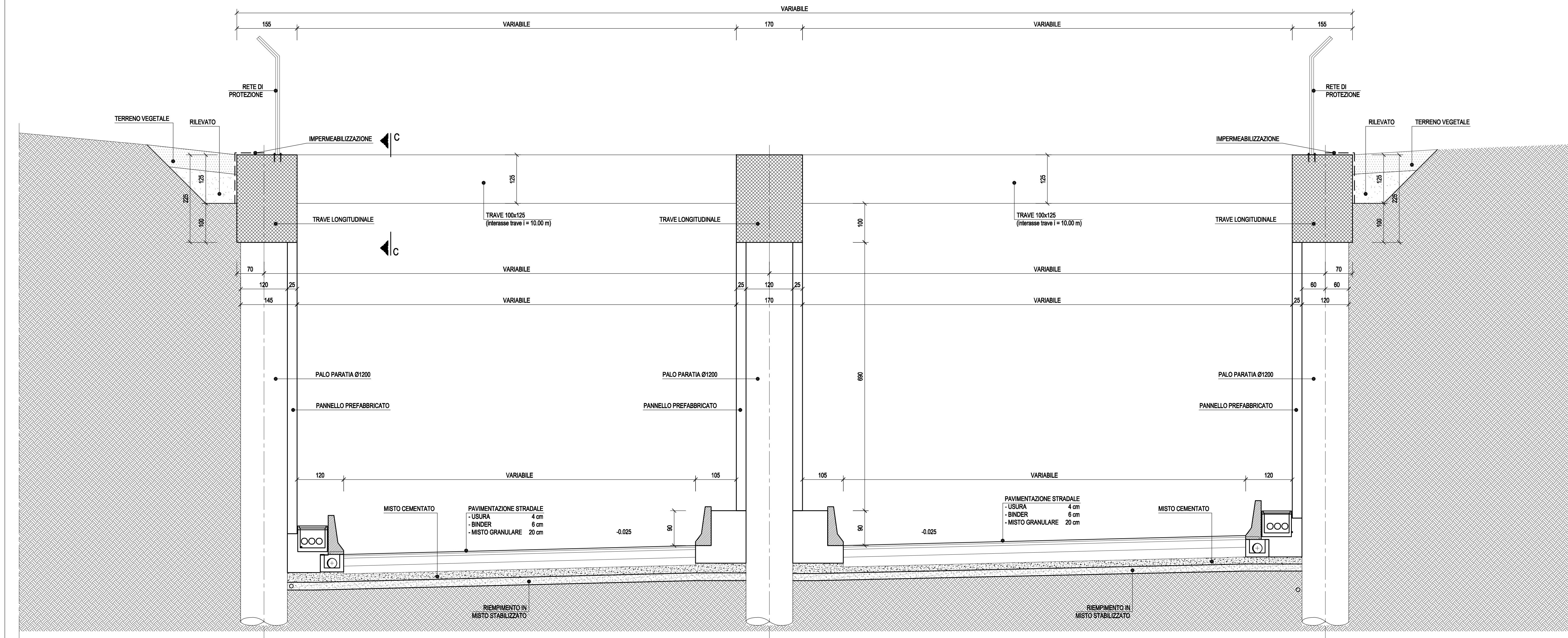
SEZIONE TIPO - TRATTI SCOPERTI (da progr. 2+955 a progr. 2+965 - da progr. 2+985 a progr. 3+300) SCALA 1:50
