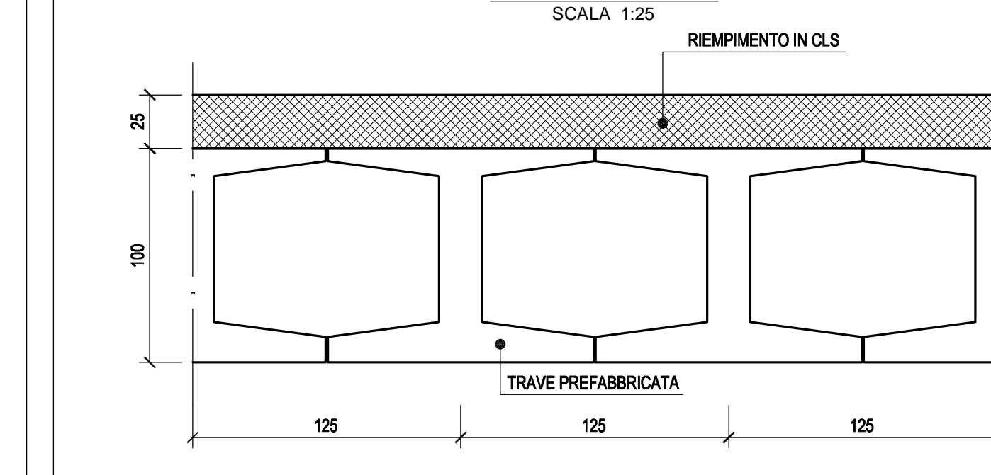
SEZIONE B-B SCALA 1:25
