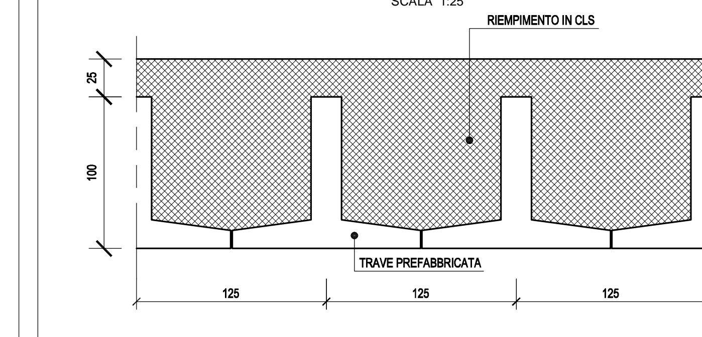
SEZIONE A-A SCALA 1:25
