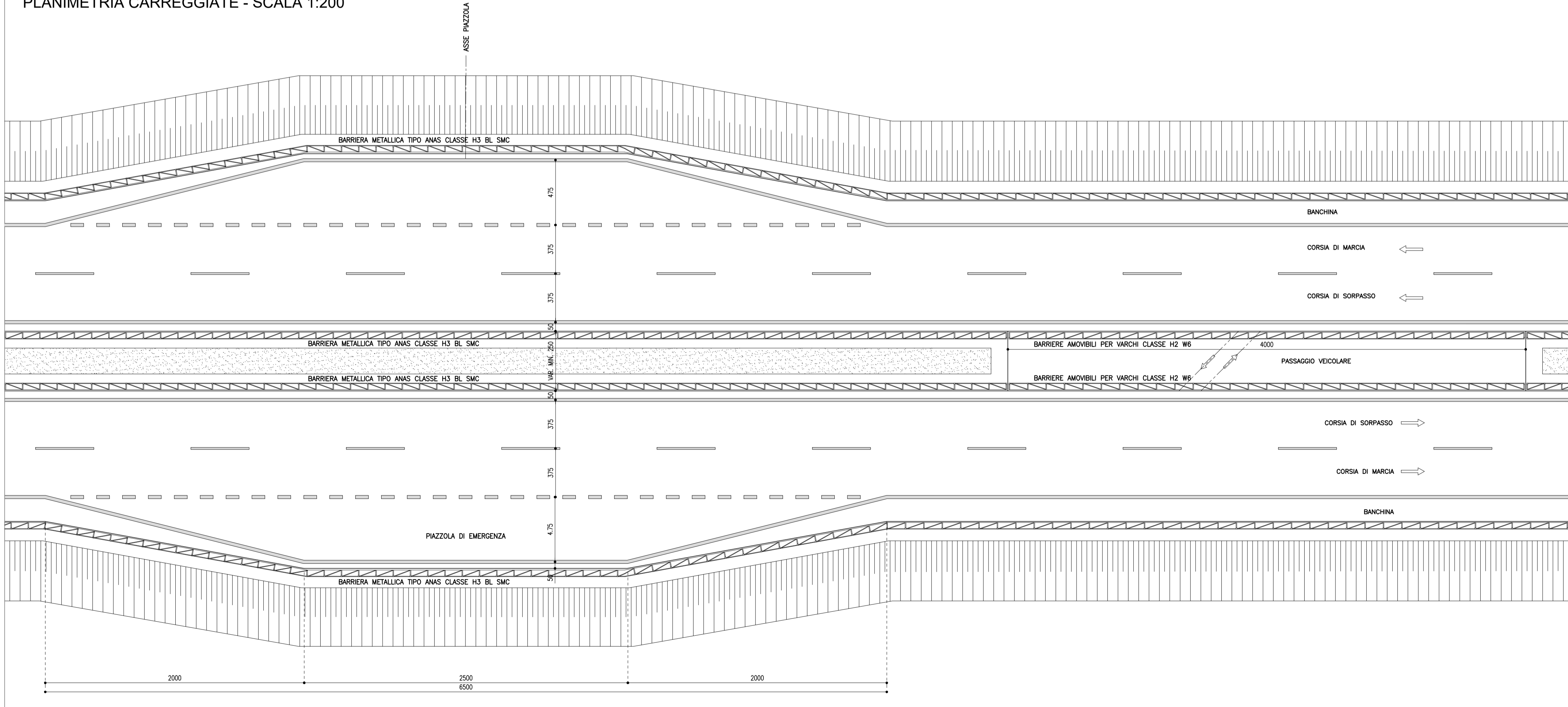
PLANIMETRIA CARREGGiate - SCALA 1:200
