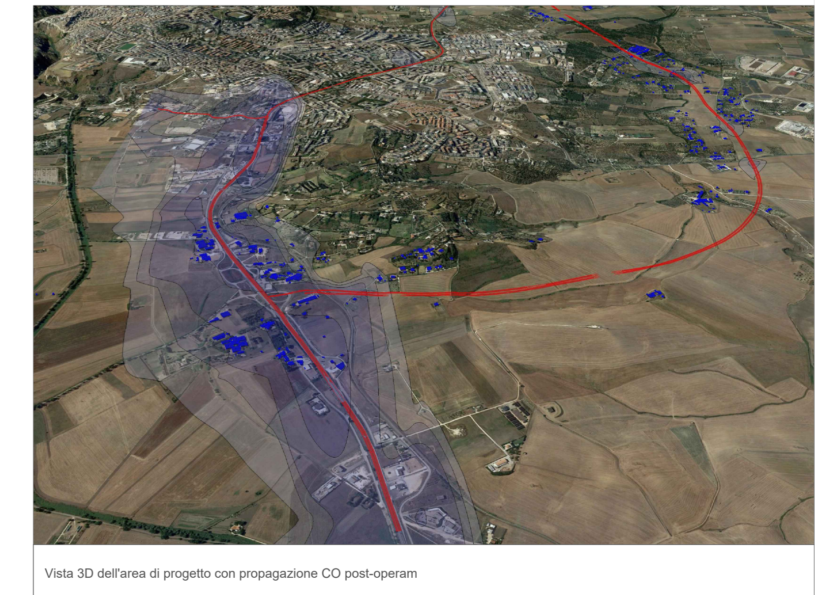
Vista 3D dell'area di progetto con propagazione CO post-operam
