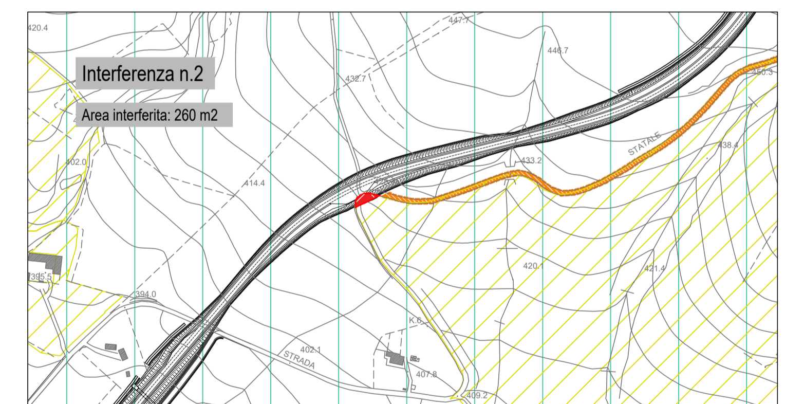
Planimetria e ortofoto Interferenza n.2
