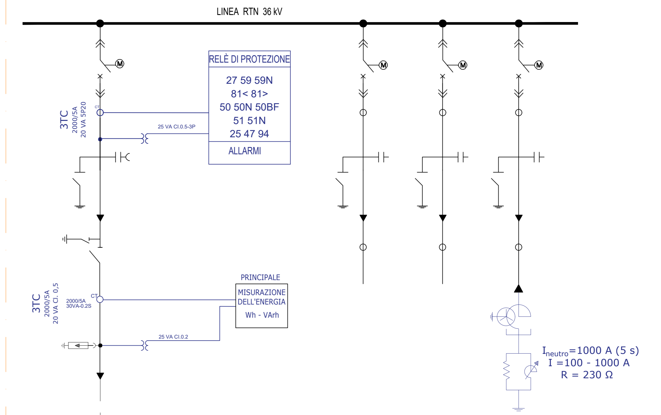
CABINA ENTE GESTORE RTN SOTTOSTAZIONE RTN (36kV)
