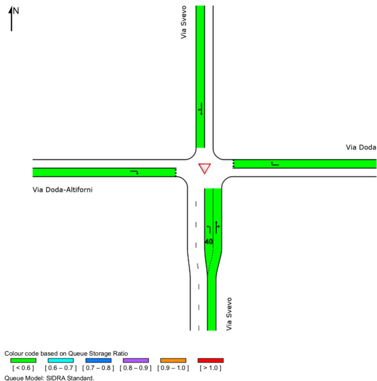
Figura 14 - Rapporto tra la lunghezza della coda e della rispettiva corsia per l'intersezione via Svevo - via Doda al 2040 nello scenario S1
