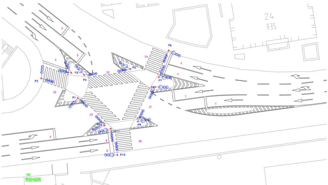
Figura 6 - Layout dell'intersezione K47 con denominazione dei relativi segnali semaforici
