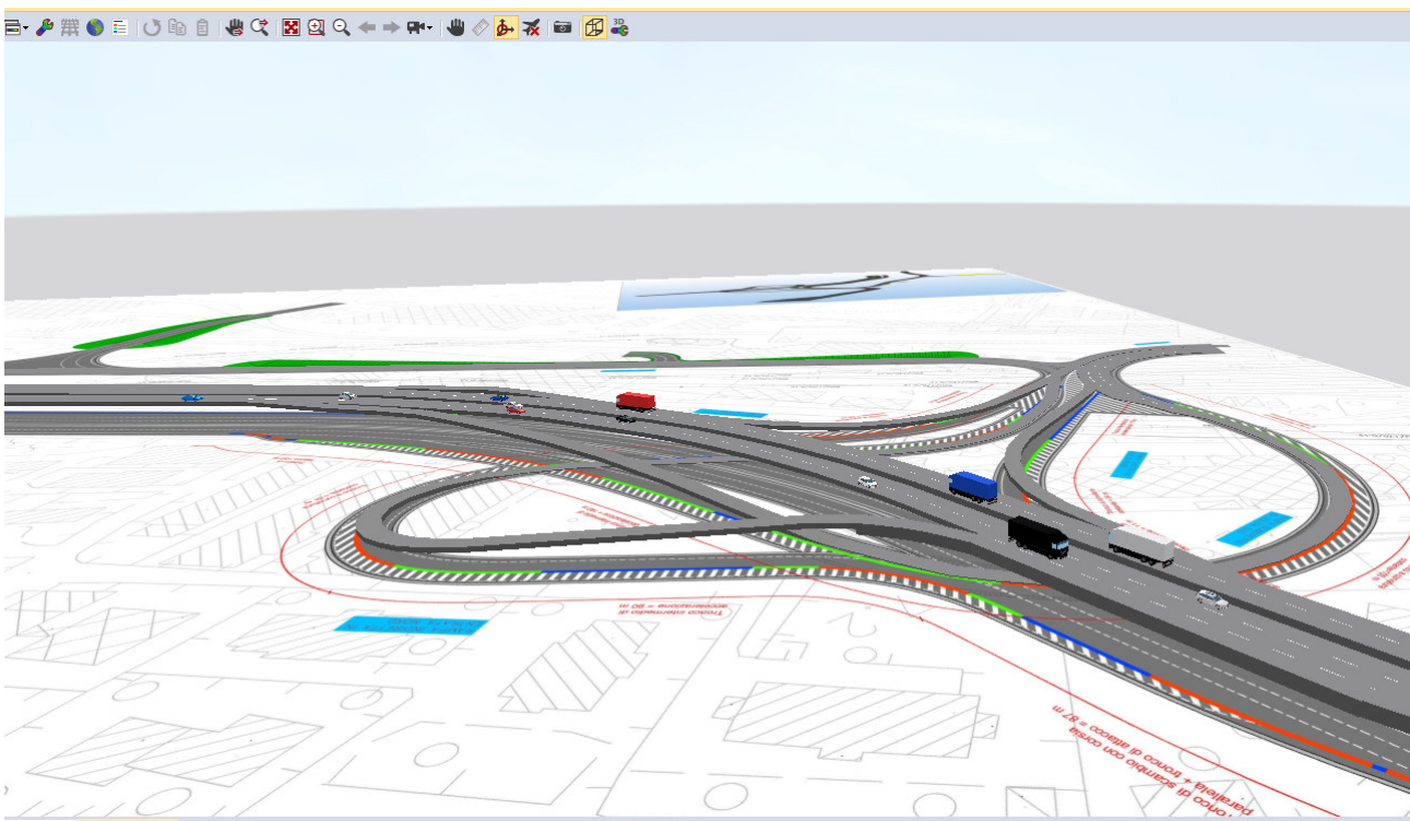
Figura 8 – Layout tridimensionale delle nuove rampe di collegamento con la GVT nello scenario di progetto
