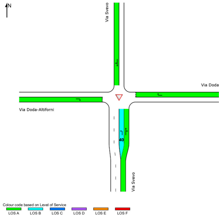
Figura 13 - LOS dell'intersezione via Svevo - via Doda al 2040 nello scenario S1
