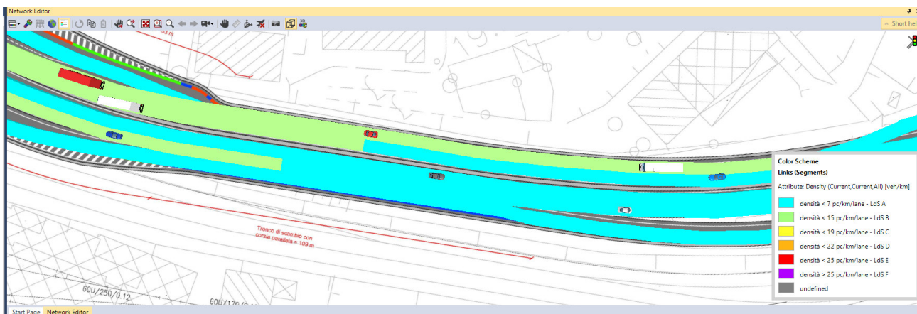
Figura 17 – Livelli di servizio nel tronco di scambio
