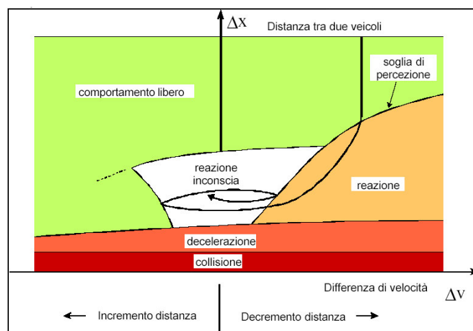
Figura 10 - Modello di successione dei veicoli secondo WIEDEMANN
