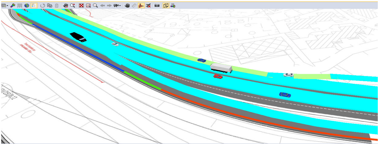
Figura 18 – Livelli di servizio nel tronco di scambio
