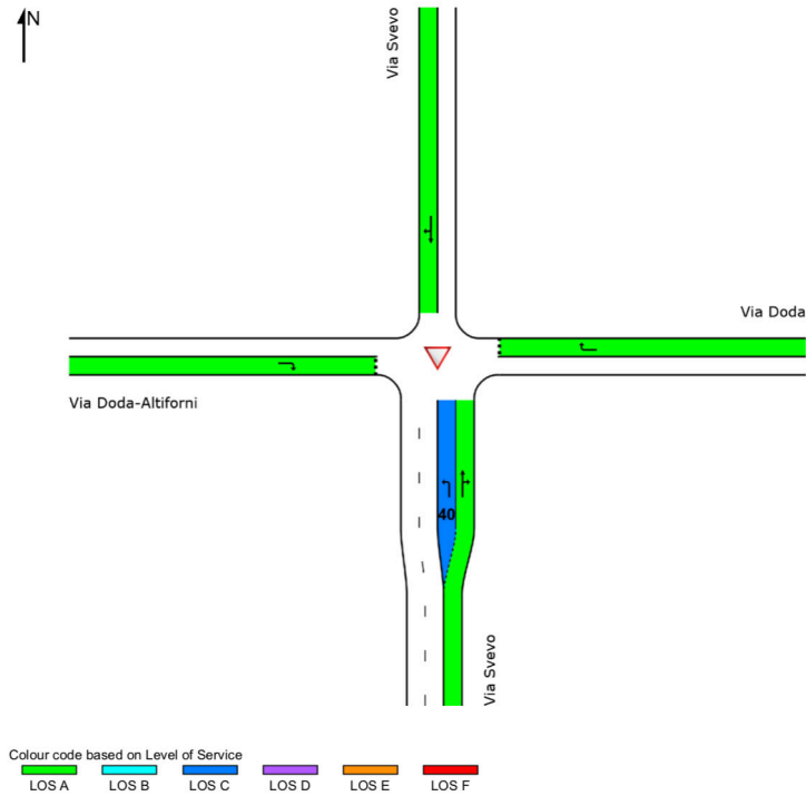
Figura 11 - LOS dell'intersezione via Svevo - via Doda al 2040 nello scenario S0
