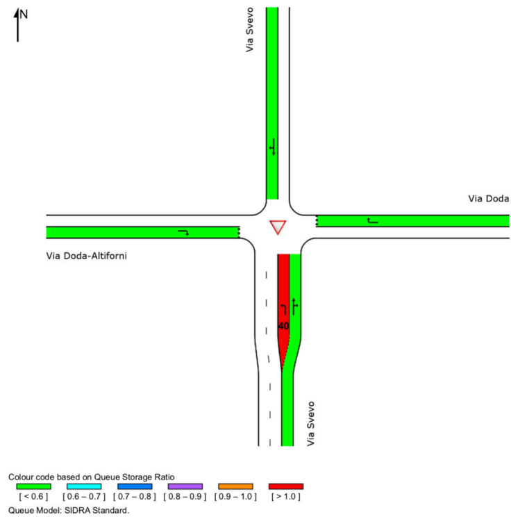
Figura 12 – Rapporto tra la lunghezza della coda e della rispettiva corsia per l'intersezione via Svevo - via Doda al 2040 nello scenario S0
