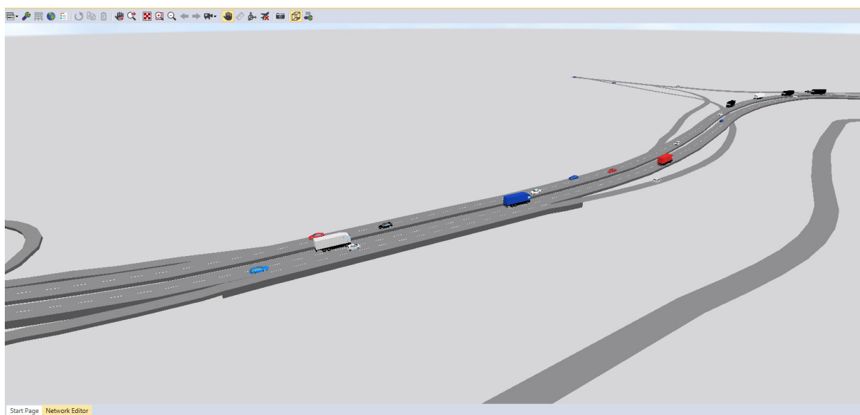
Figura 15 - Vista prospettica dell'intero modello
