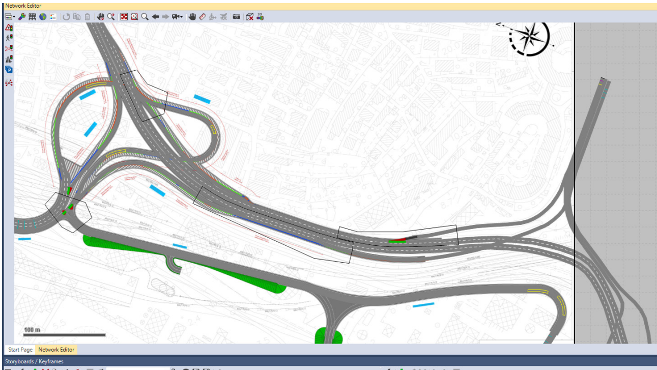
Figura 7 - Layout delle nuove rampe di collegamento con la GVT nello scenario di progetto
