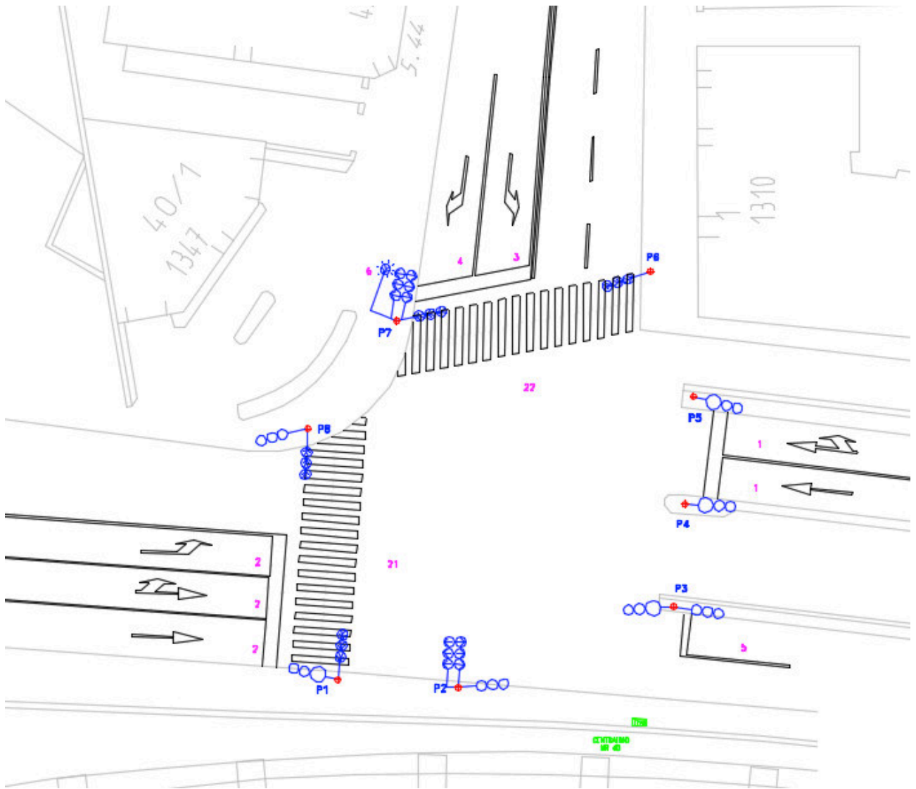
Figura 5 - Layout dell'intersezione K40 con denominazione dei relativi segnali semaforici
