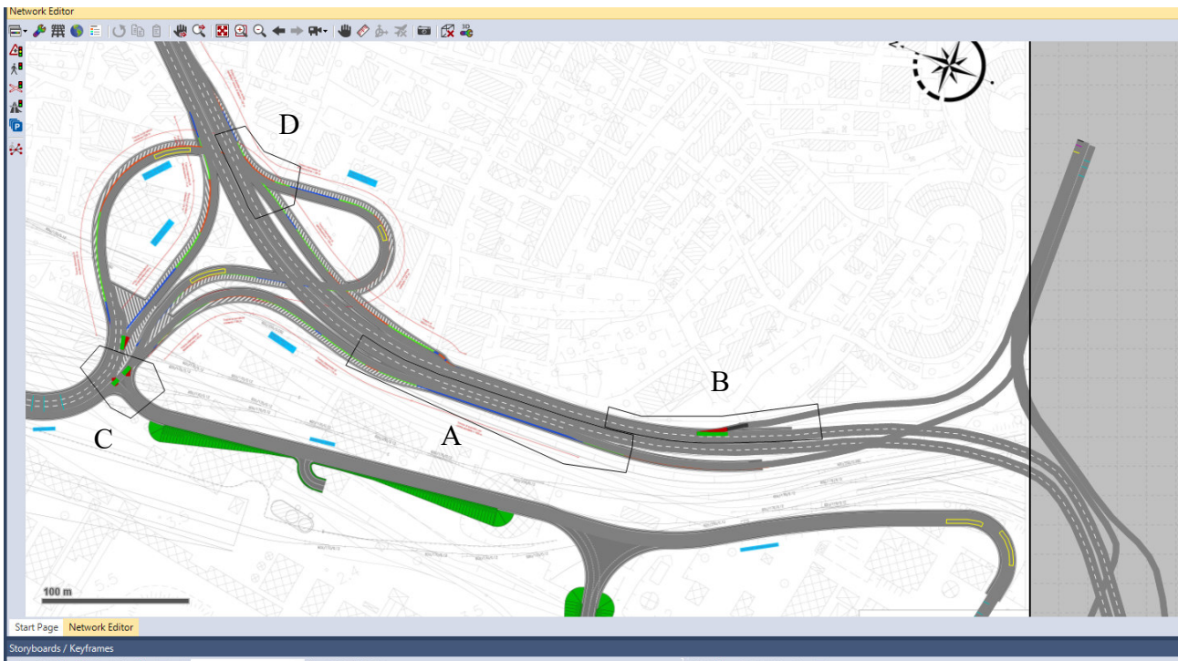
Figura 16 - Vista planimetrica del modello e delle aree di interesse
