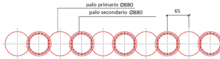
Figura 6-8: pianta pali secanti della paratia
