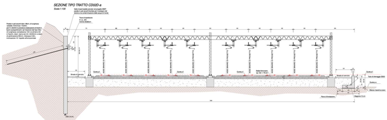
Figura 6-9: Sezione tipo nel tratto CD02D-a (paratia)
