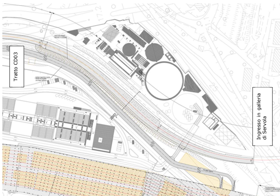
Figura 6-19: planimetria di dettaglio del tratto CD02C
