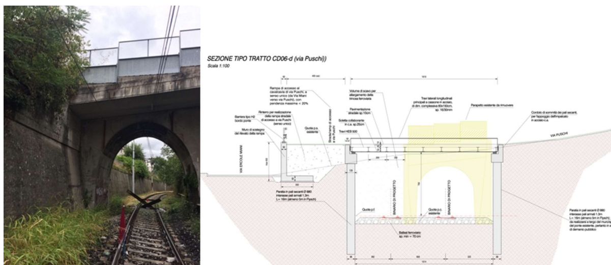
Figura 6-15: cavalcavia esistente, e sez. long. della nuova opera
