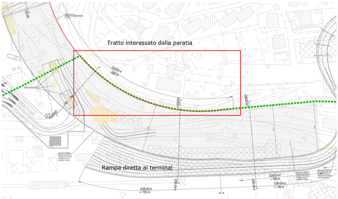
Figura 6-7: Zona Centrale – in evidenza il tratto interessato alla paratia
