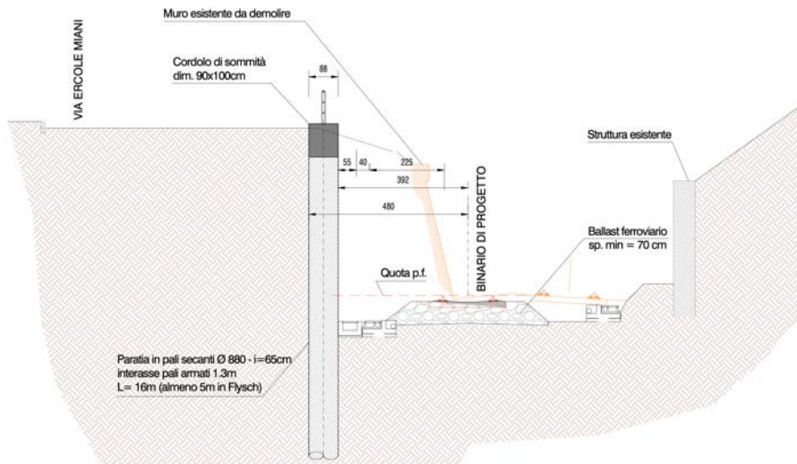
Figura 3-9 Sezione tipo del tratto in trincea lungo l'asta di manovra
