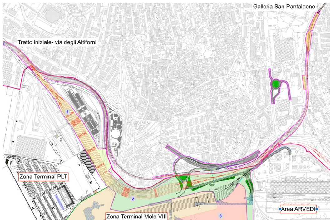
Figura 3-1 Planimetria dell'intervento
