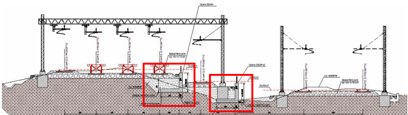
Figura 3-7 Sezione tipo in rilevato con evidenziati i muri di sostegno
