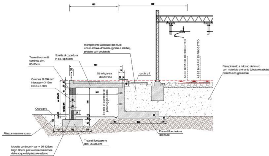
Figura 3-4 Sezione in corrispondenza della corsia di accesso al parcheggio
