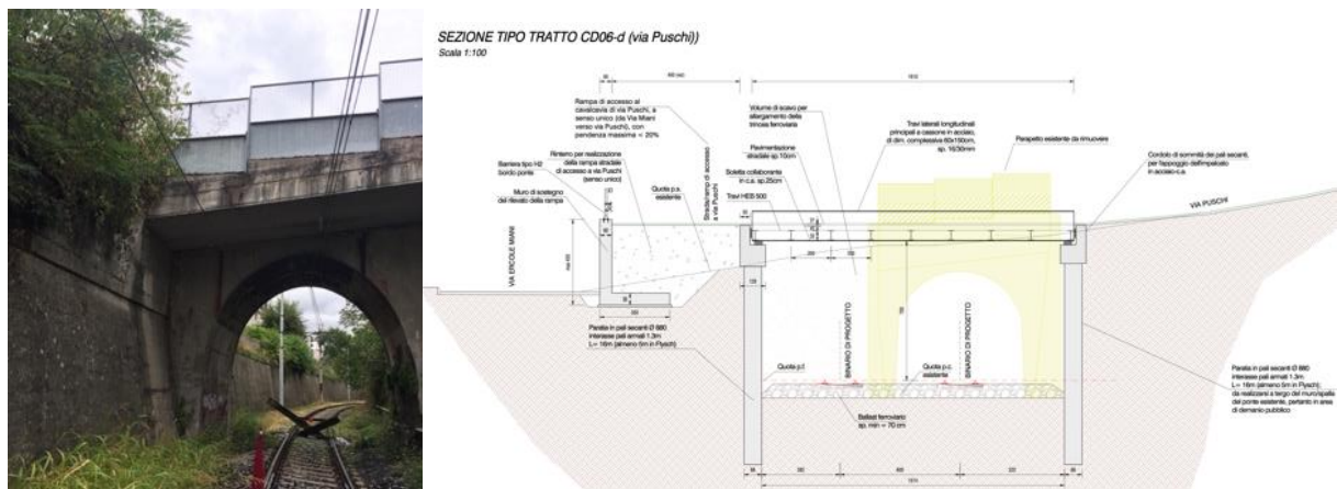
Figura 3-10 Cavalcavia esistente e opera di progetto
