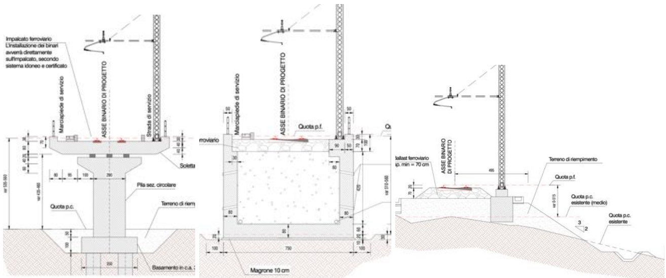
Figura 3-5 Sezioni tipo del tratto ferroviario su impalcato (a sx), su rilevato sostenuto (in centro) e su rilevato in terra (a dx)
