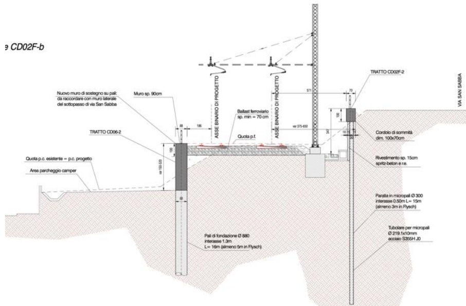
Figura 3-8 Sezione tipo del rilevato ferroviario sostenuta con paratie di pali e di micropali realizzate rispettivamente a valle e a monte
