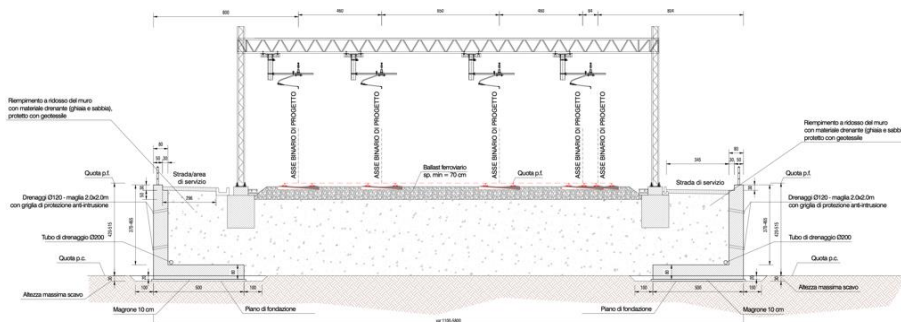
Figura 3-3 Sezione tipica in corrispondenza del tratto in rilevato con muri di sostegno
