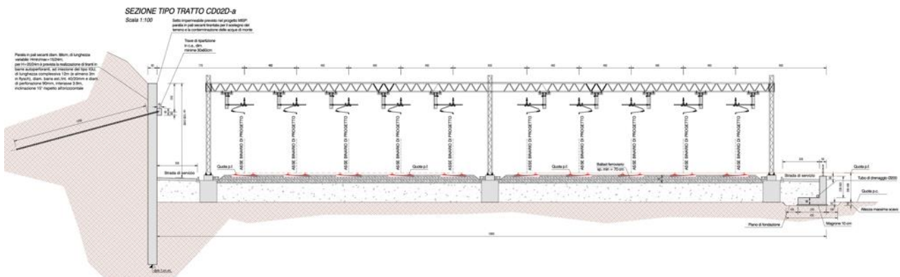
Figura 3-6 Sezione tipo nel tratto con terreno di monte sostenuto dalla paratia in pali secanti tirantata
