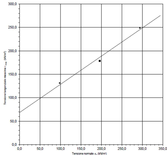
Figura 4-1: Verticale SG001 - Campione CR1 – Prova a taglio diretto
