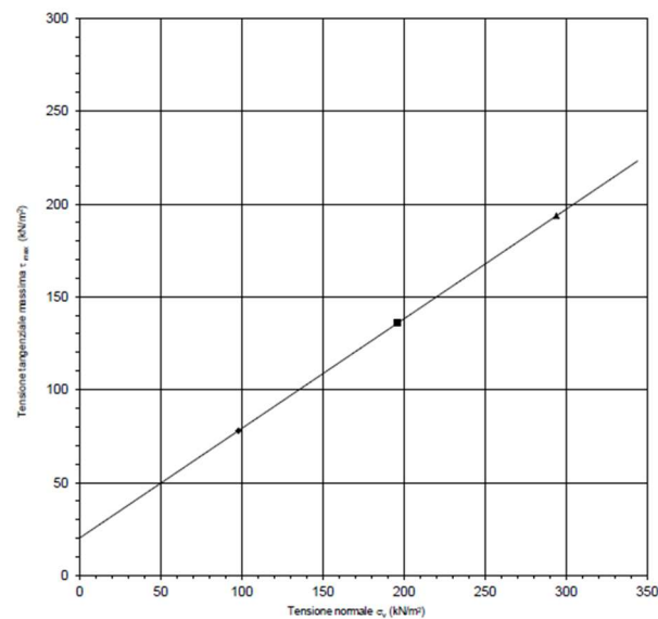
Figura 4-2: Verticale SG001 - Campione CI1 - Prova a taglio diretto.
