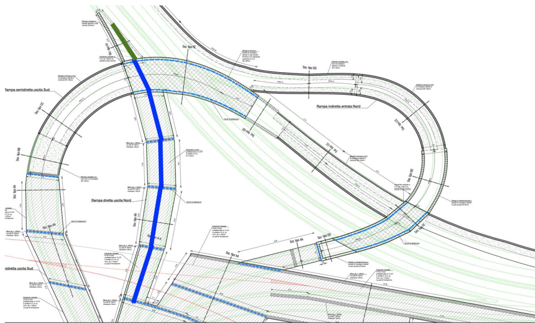
Figura 7-5: planimetria con evidenziata la rampa diretta uscita Nord
