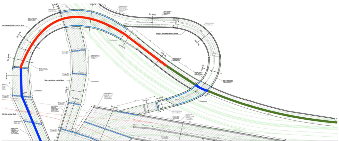
Figura 7-3: planimetria con evidenziata la rampa semidiretta uscita Sud
