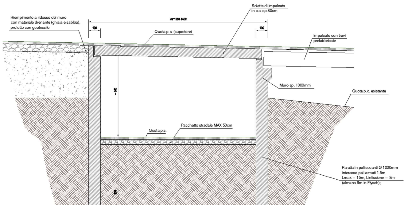
Figura 7-6: sezione tipo su scavalco rampa in uscita Sud
