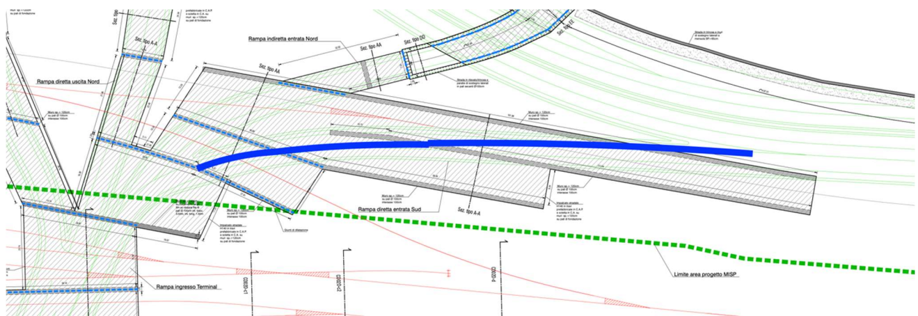
Figura 7-8: planimetria con evidenziata la rampa diretta uscita Sud
