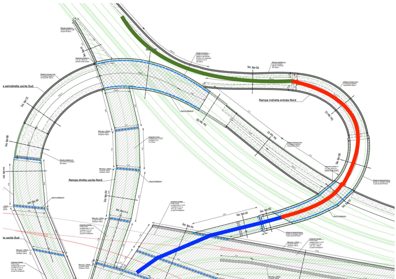
Figura 7-7: planimetria con evidenziata la rampa indiretta in entrata Nord
