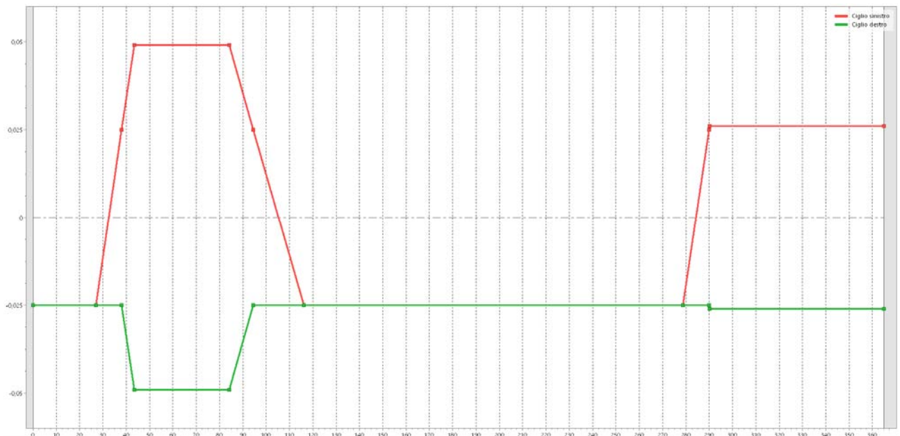
Figura 40: Andamento delle sopraelevazioni – Rampa terminal
