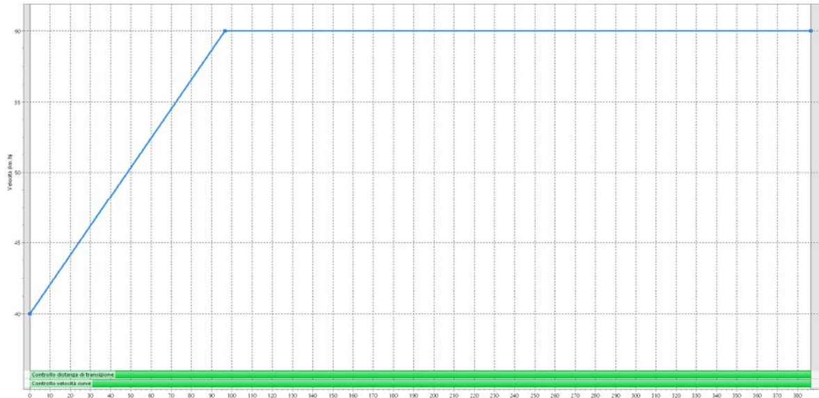
Figura 15: Diagramma delle velocità - Rampa diretta in entrata sud
