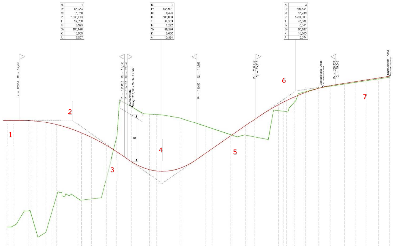
Figura 56: Andamento altimetrico dell'asse stradale - Rampa indiretta in entrata nord
