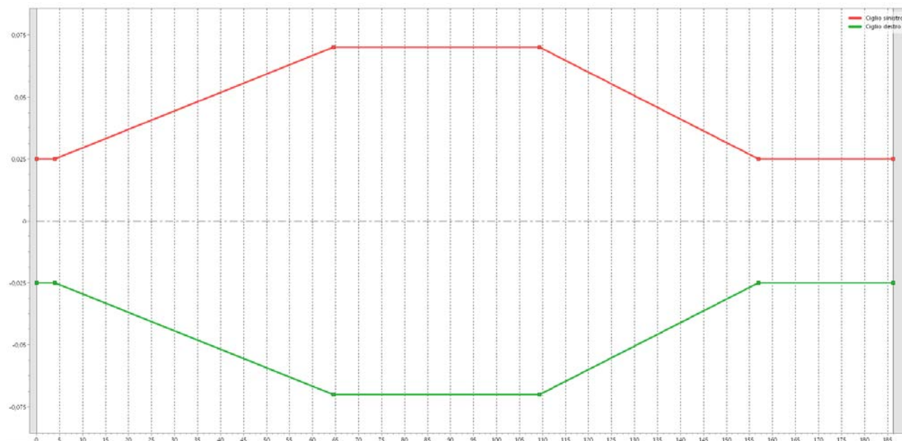
Figura 29: Andamento delle sopraelevazioni - rampa diretta in uscita nord
