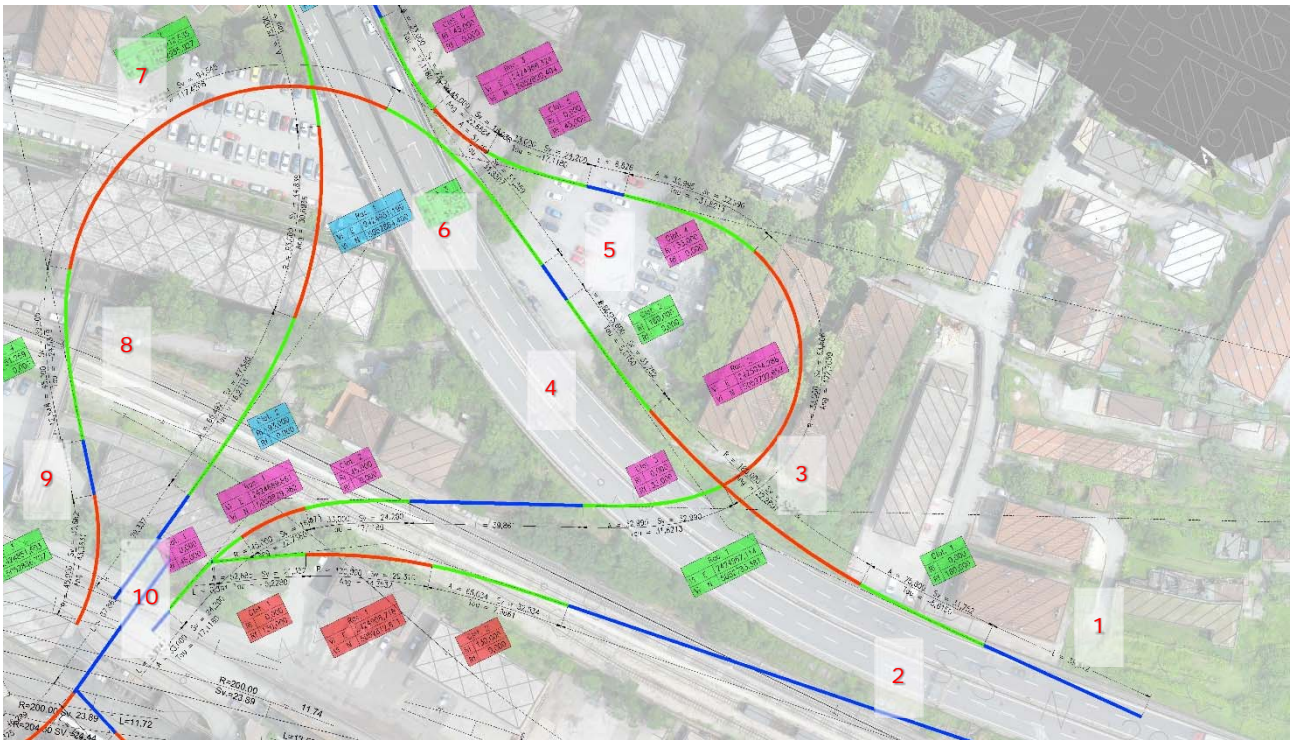
Figura 19: Andamento planimetrico dell'asse stradale - Rampa semidiretta in uscita sud
