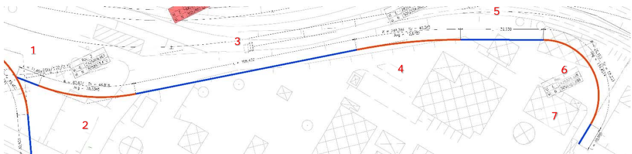
Figura 44: Andamento planimetrico dell'asse stradale - Svincolo in direzione dell'area ARVEDI
