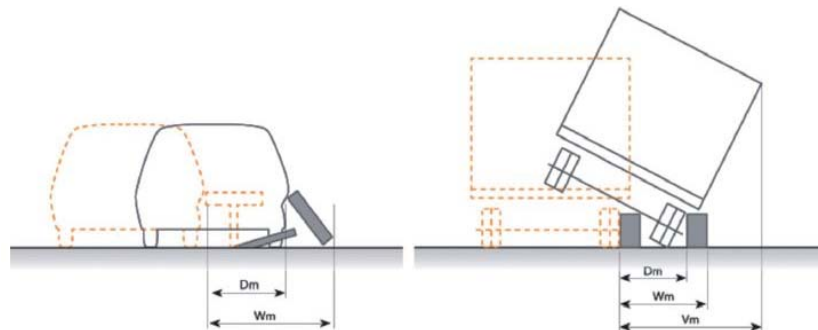
Figura 82: Schemi per la misura dei parametri geometrici
