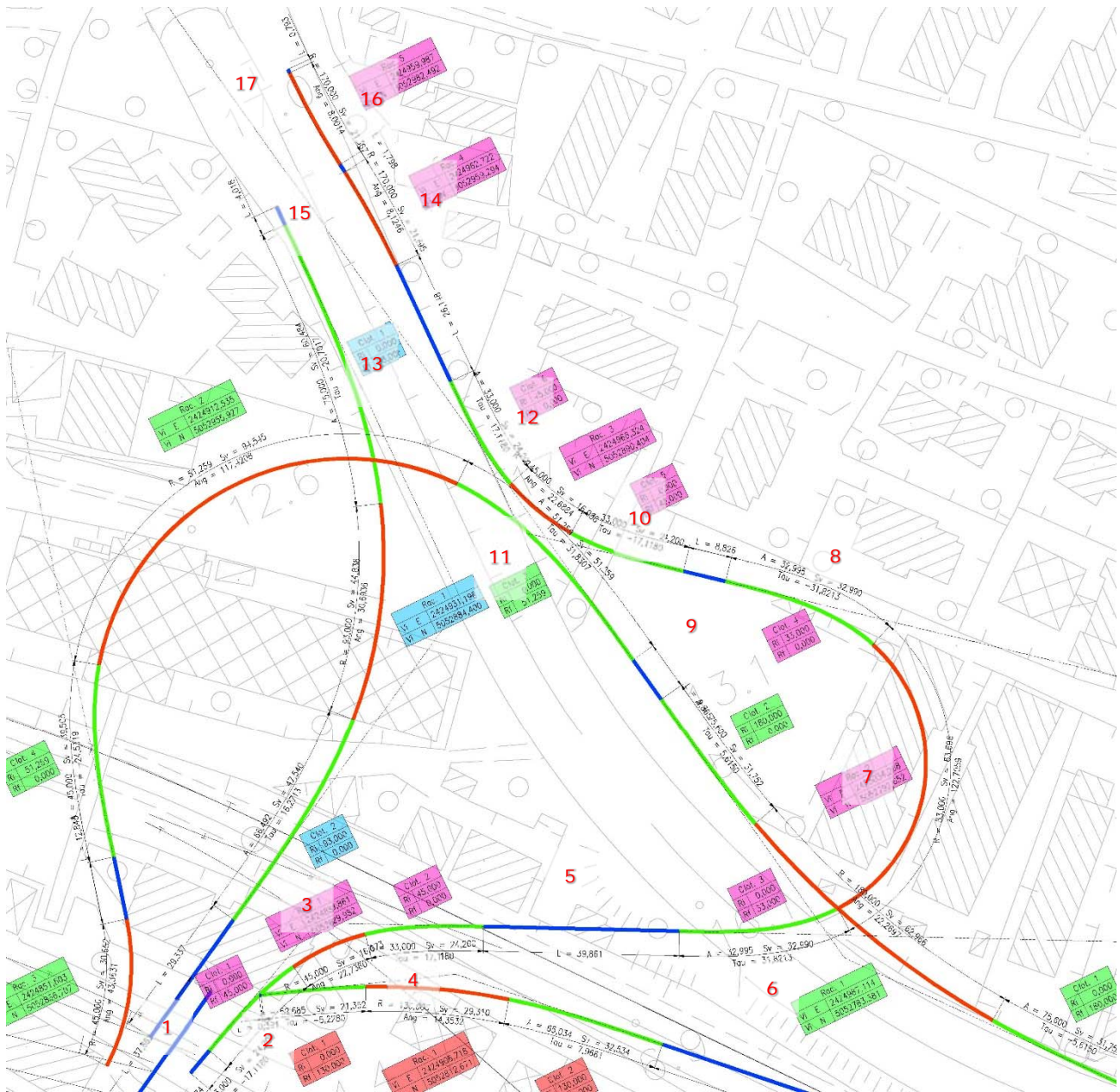
Figura 31: Andamento planimetrico dell'asse stradale - Rampa indiretta in entrata nord
