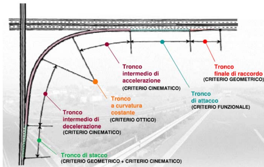
Figura 11: Geometria generica di una rampa
