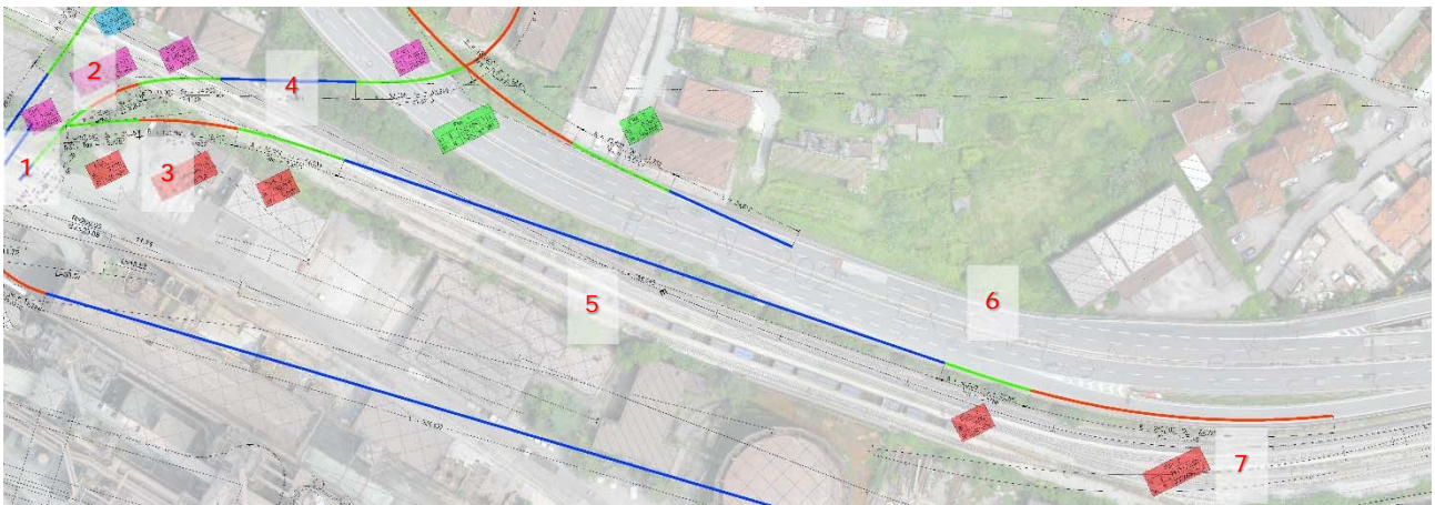
Figura 6: Andamento planimetrico dell'asse stradale - Rampa diretta in entrata sud
