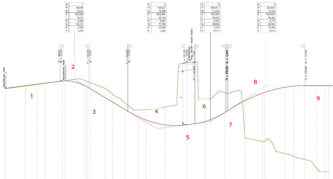
Figura 50: Andamento altimetrico dell'asse stradale - Rampa semidiretta in uscita sud
