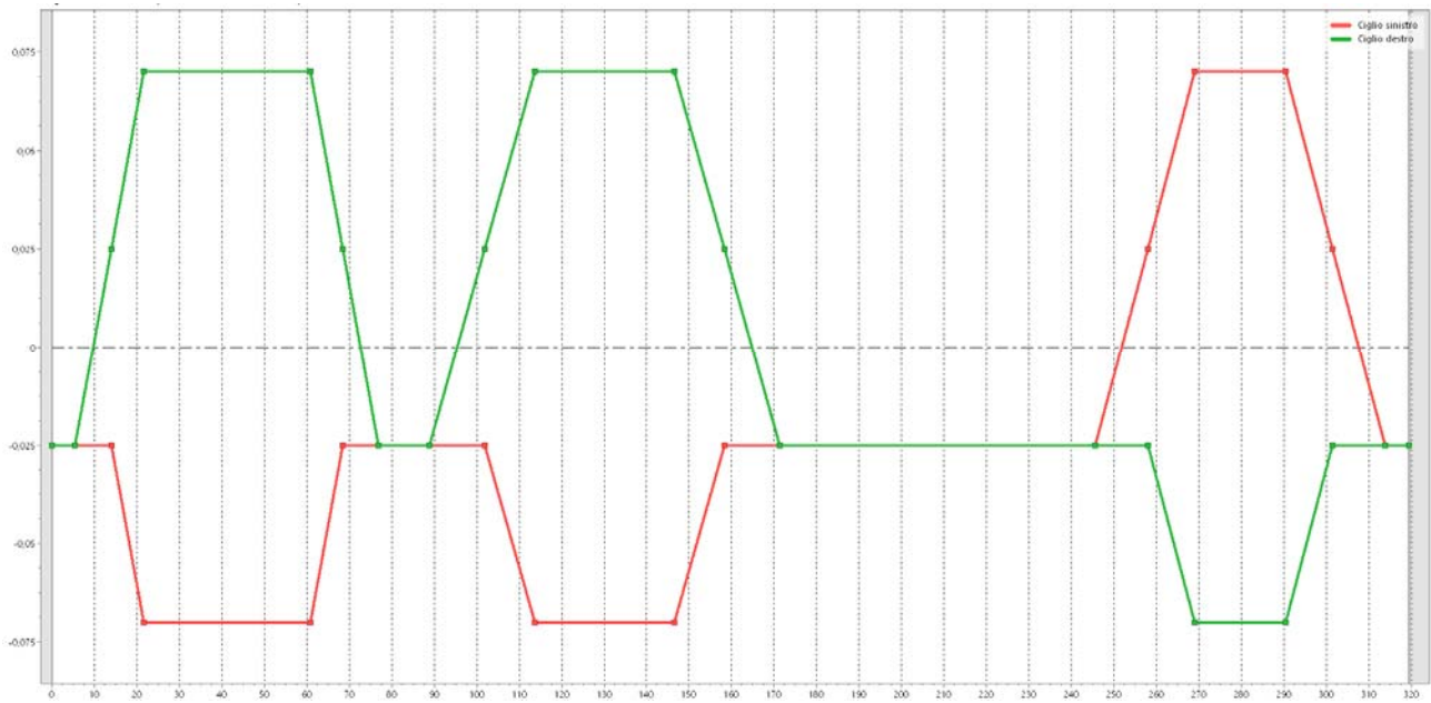
Figura 46: Andamento delle sopraelevazioni - Svincolo in direzione dell'area ARVEDI
