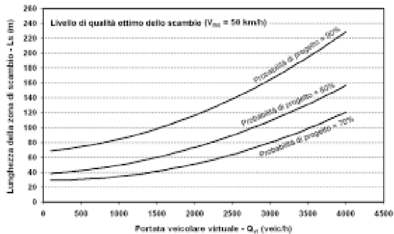
Figura 14: Abaco di dimensionamento dei tronchi di scambio
