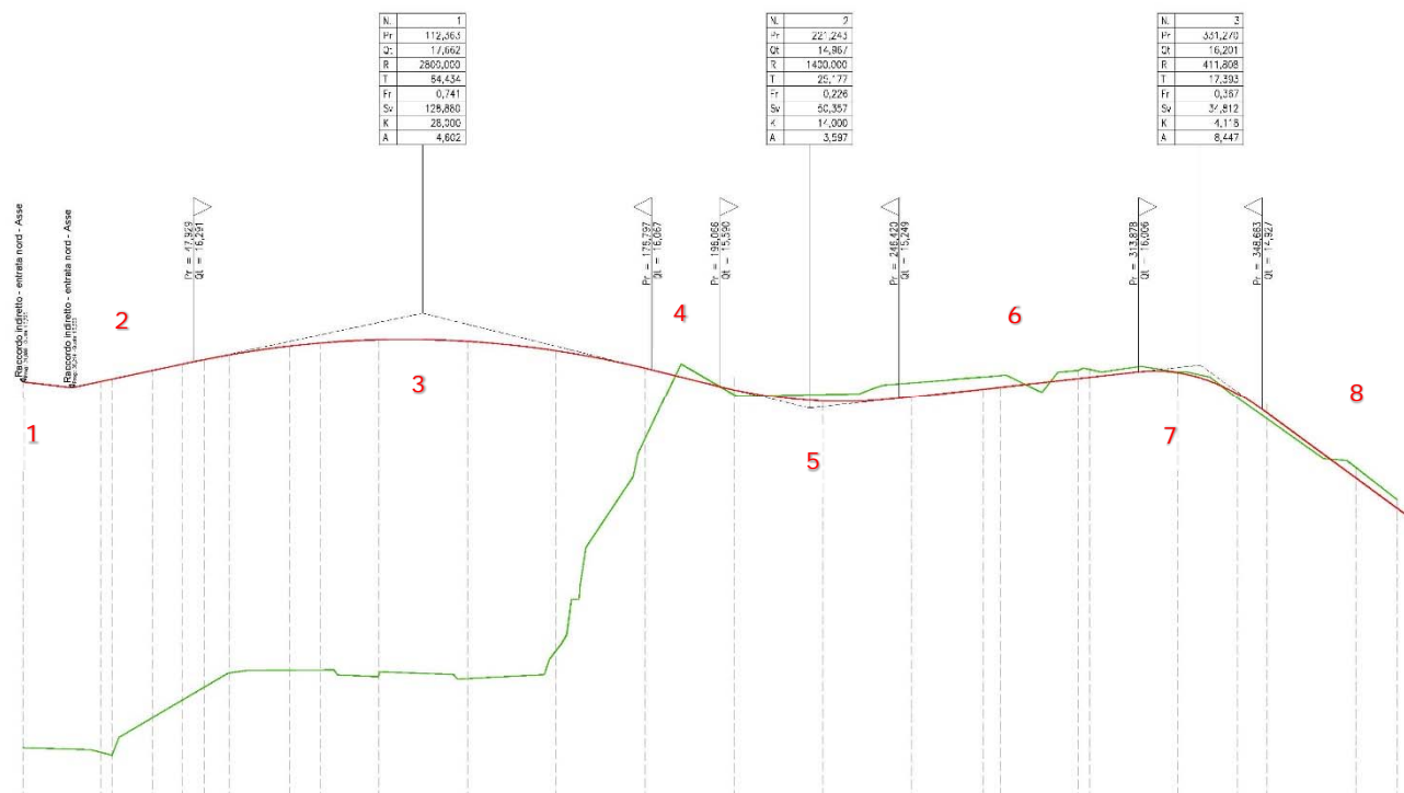
Figura 47: Andamento altimetrico dell'asse stradale - Rampa diretta in entrata sud
