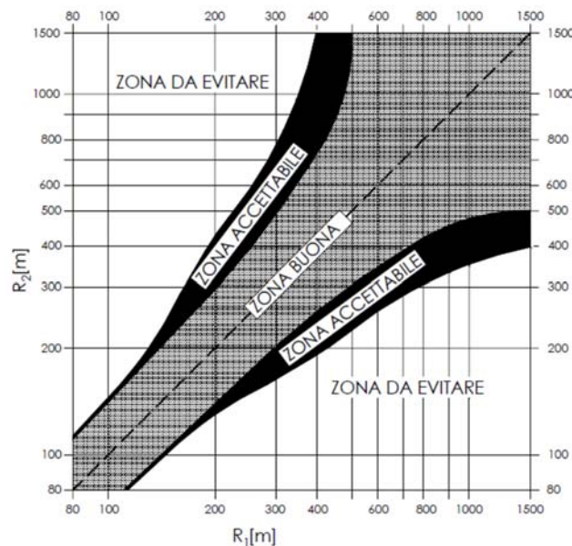
Figura 9: Abaco del rapporto tra curve consecutive
