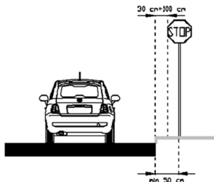
Figura 31: Distanza del segnale dalla banchina
