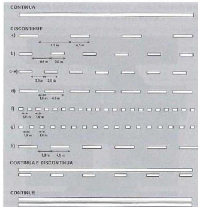
Figura 33: Tipologia e caratterizzazione delle strisce longitudinali (parte 1)
