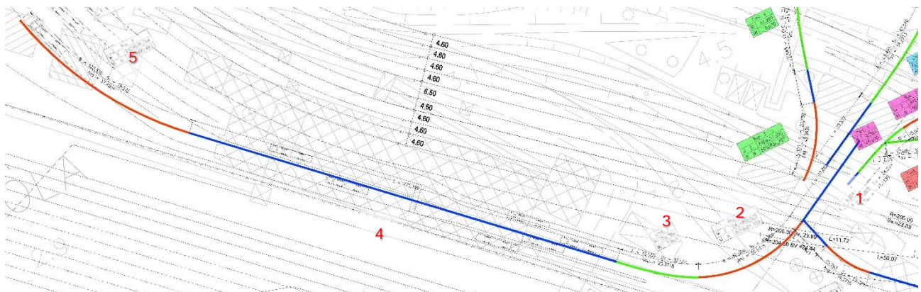
Figura 38: Andamento planimetrico dell'asse stradale - Rampa terminal
