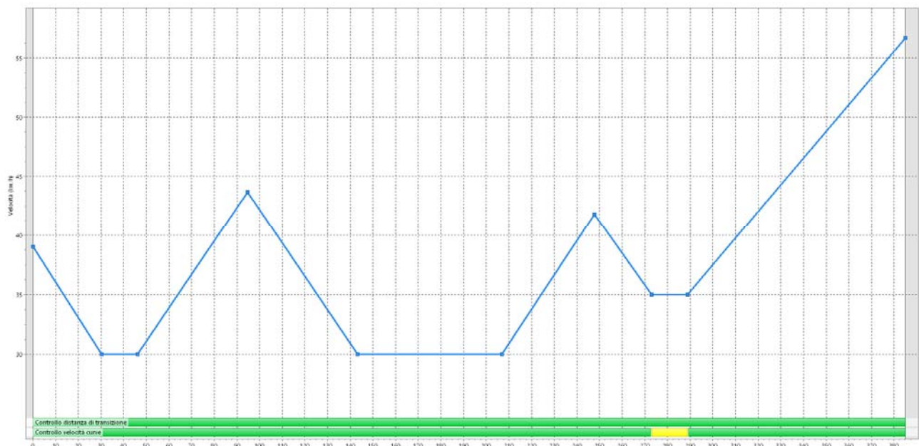
Figura 35: Diagramma delle velocità - Rampa indiretta in entrata nord
