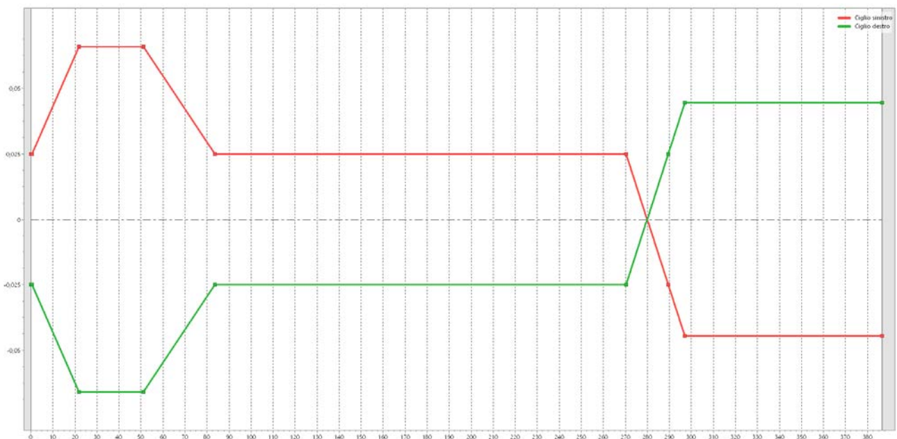
Figura 17: Andamento delle sopraelevazioni - Rampa diretta in entrata sud
