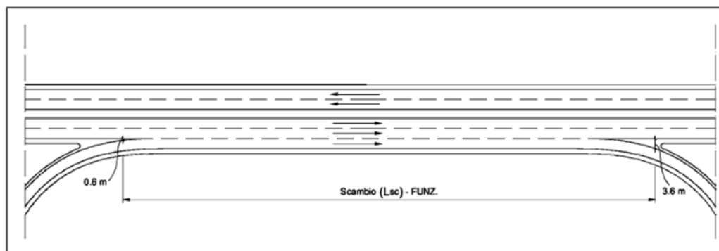
Figura 13: Schema di un tronco di scambio
