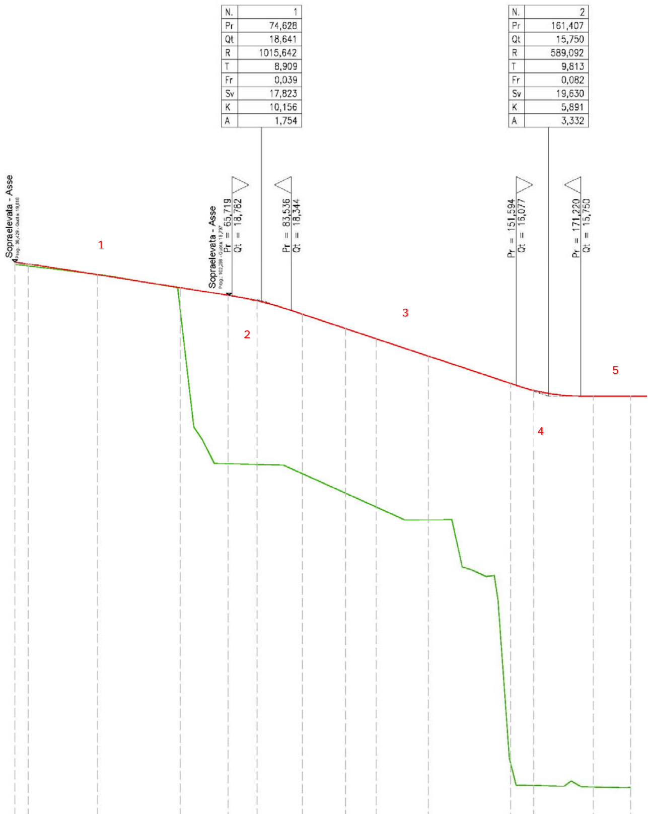
Figura 53: Andamento altimetrico dell'asse stradale - Rampa diretta in uscita nord
