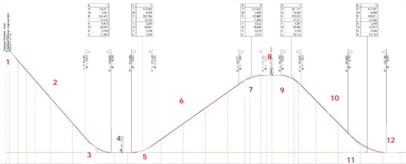
Figura 61: Andamento altimetrico dell'asse stradale - Rampa di ingresso all'area ARVEDI
