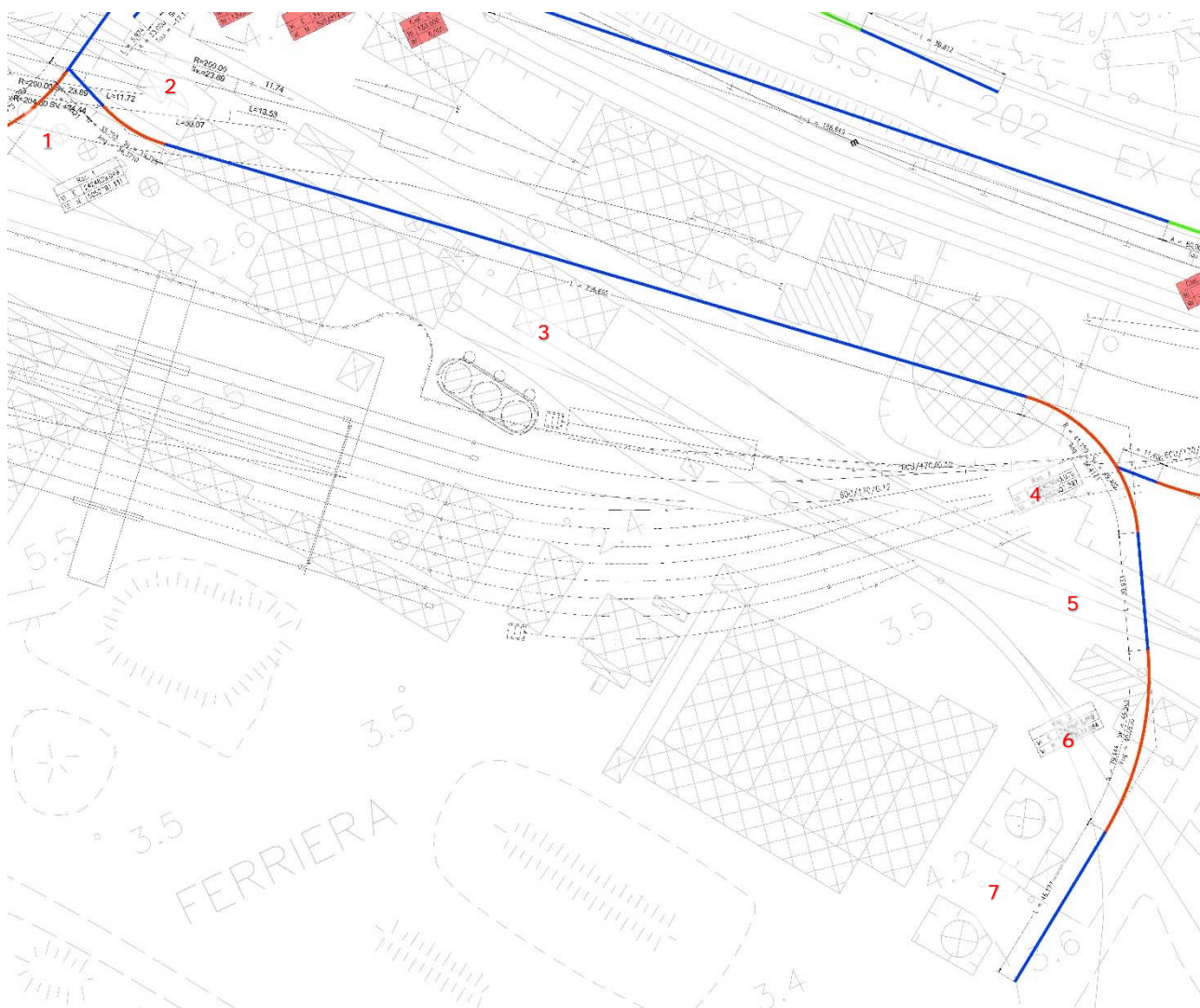
Figura 41: Andamento dell'asse stradale - Ingresso all'area ARVEDI
