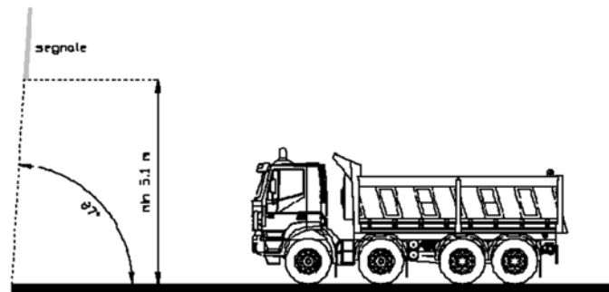
Figura 32: Altezza e inclinazione del segnale
