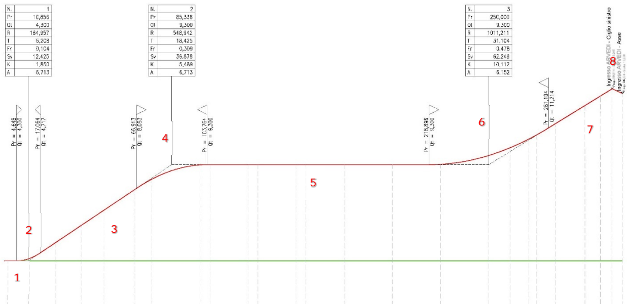
Figura 63: Andamento altimetrico dell'asse stradale - Rampa di svincolo per l'area ARVEDI
