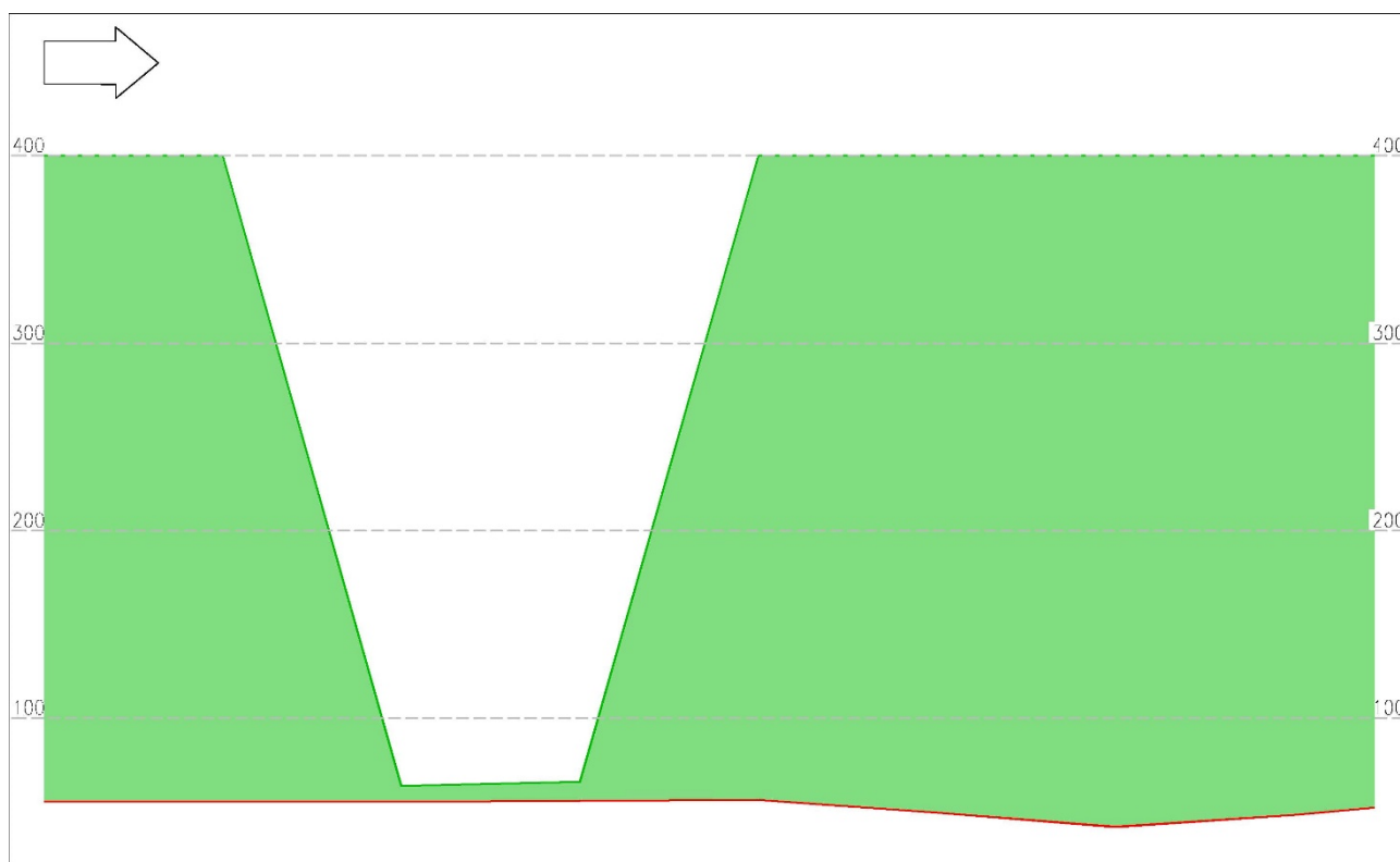
Figura 70: Verifica visibilità per l'arresto - Rampa diretta in uscita nord
