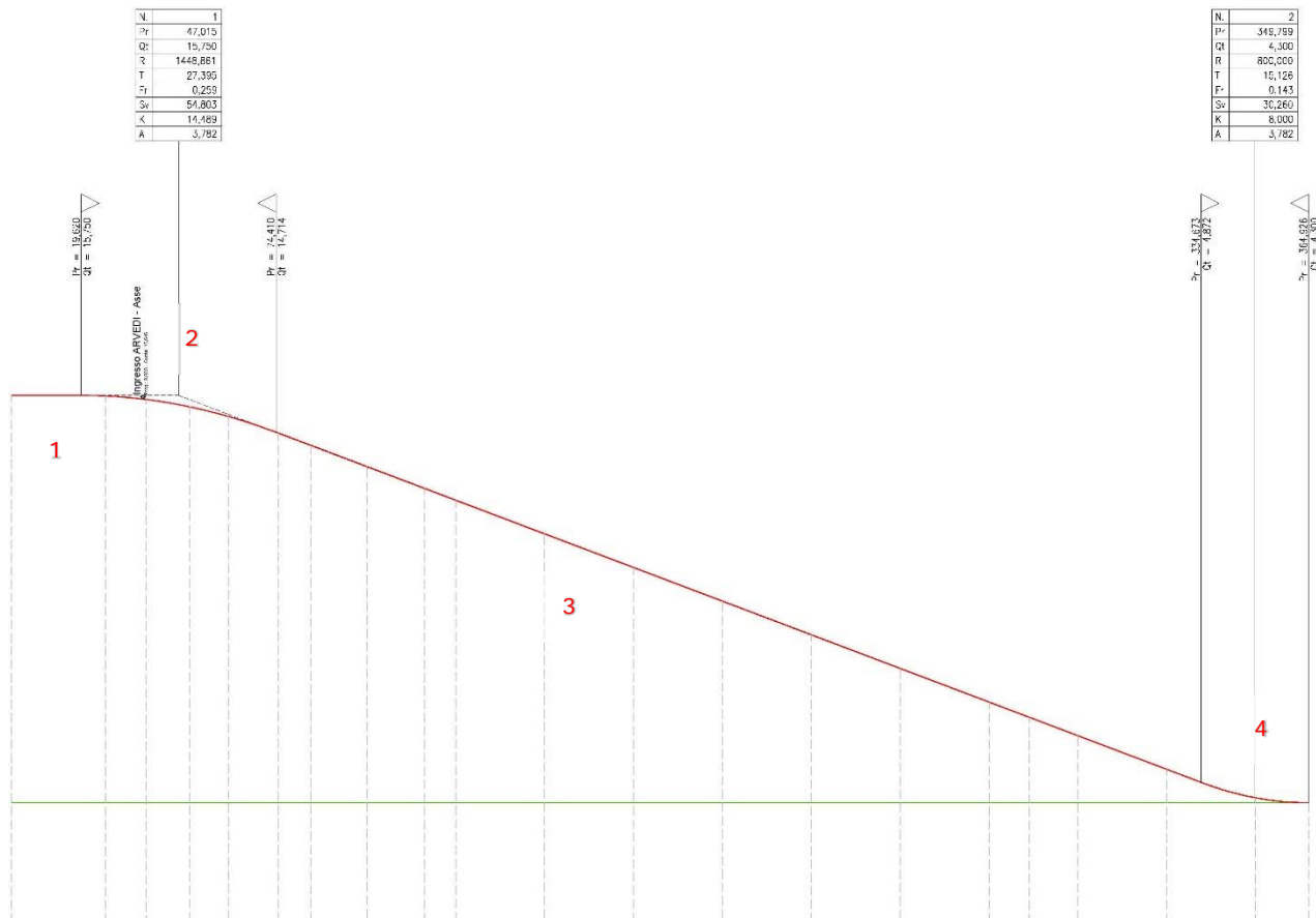
Figura 59: Andamento altimetrico dell'asse stradale - Rampa di accesso al Terminal
