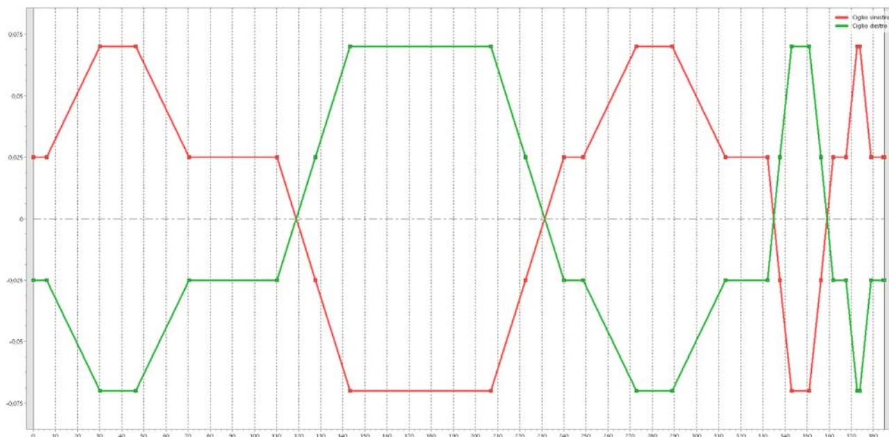
Figura 36: Andamento delle sopraelevazioni - Rampa indiretta in entrata nord
