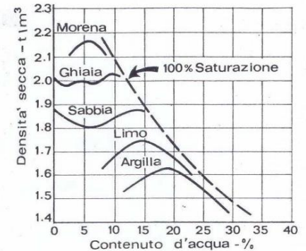
Figura 48 Curva di compattazione da prove di laboratorio in terreni incoerenti
