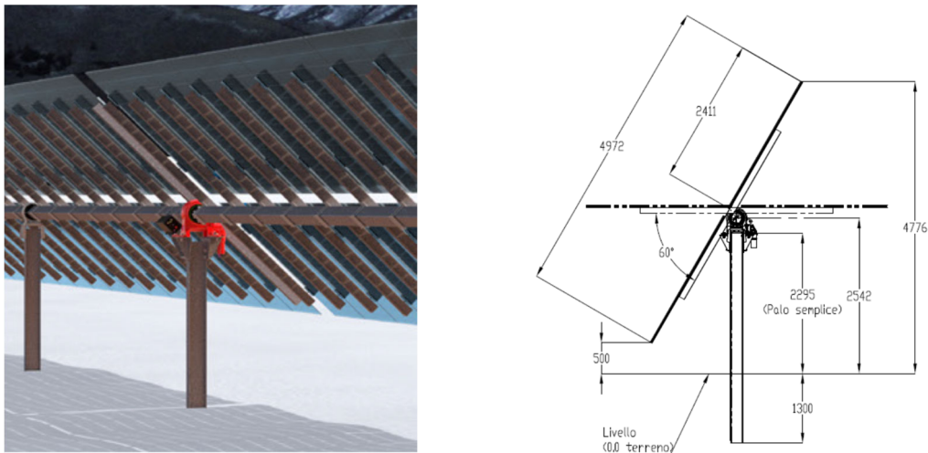
Figura 6.3: esempi di inseguitori monoassiali
