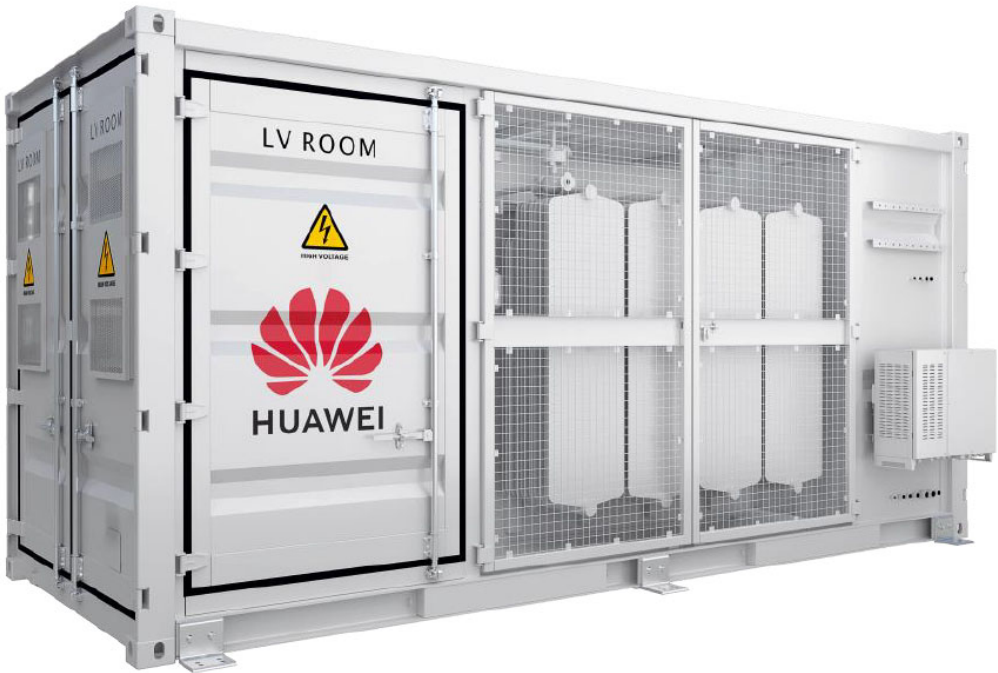
Figura 6.4:Stazione di energia
