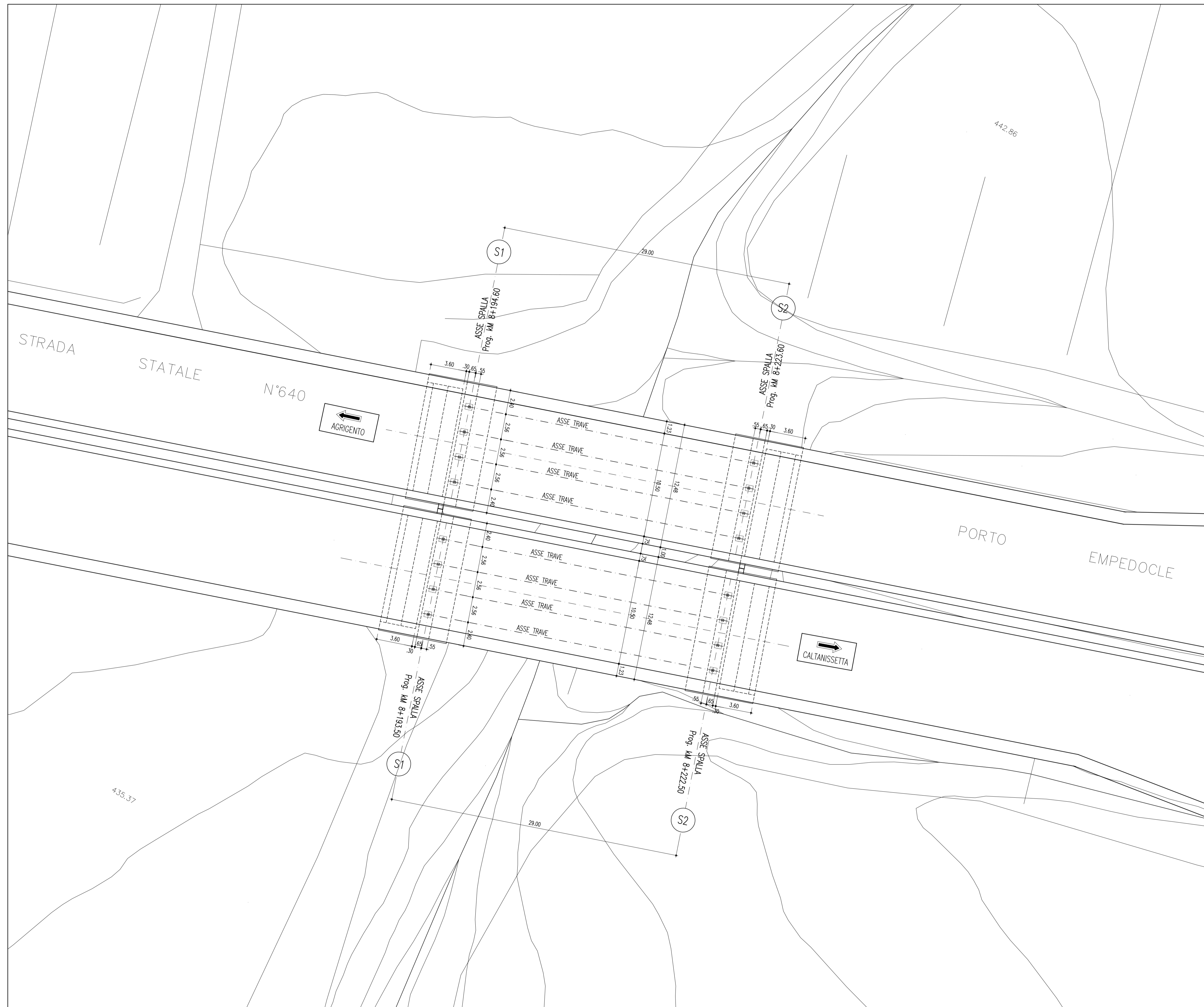
PIANTA IMPALCATO SCALA 1 : 200
