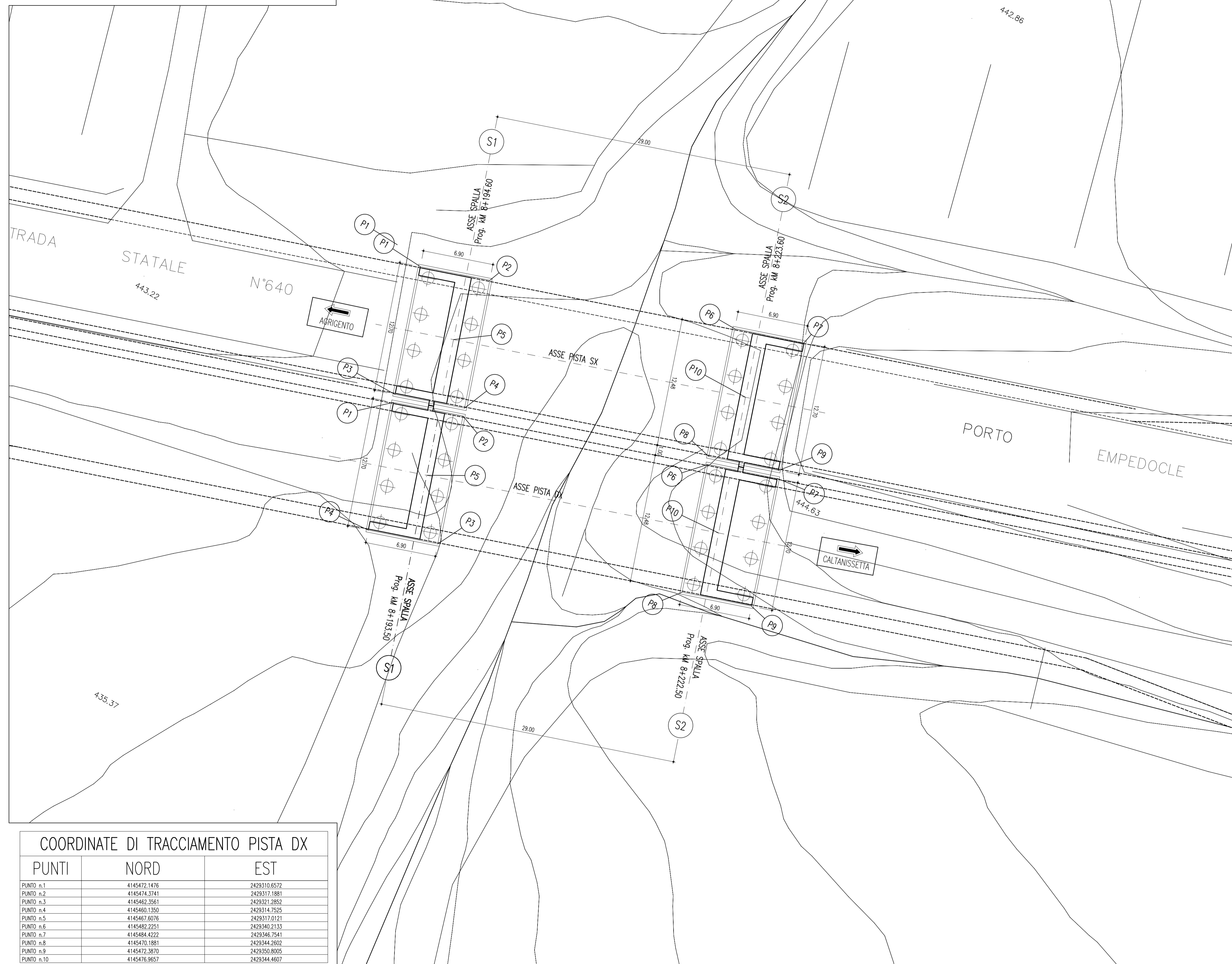
PIANTA FONDAZIONI SCALA 1 : 200
