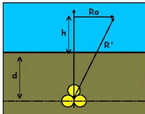
Figura 4-1: Schema e distanze di cavi interrati posati a trifoglio
