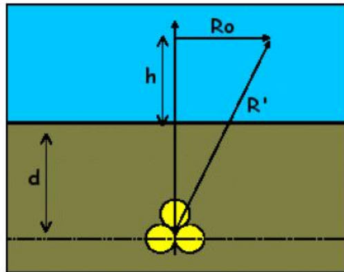
Figura 4-2: Schema e distanze di cavi interrati posati a trifoglio
