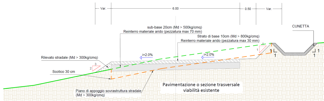
Figura 3-6: Sezioni stradali tipo. Estratto elaborato "GRE.EEC.D.99.IT.W.17279.00.080 - Tipico sezione stradali con particolari costruttivi"
