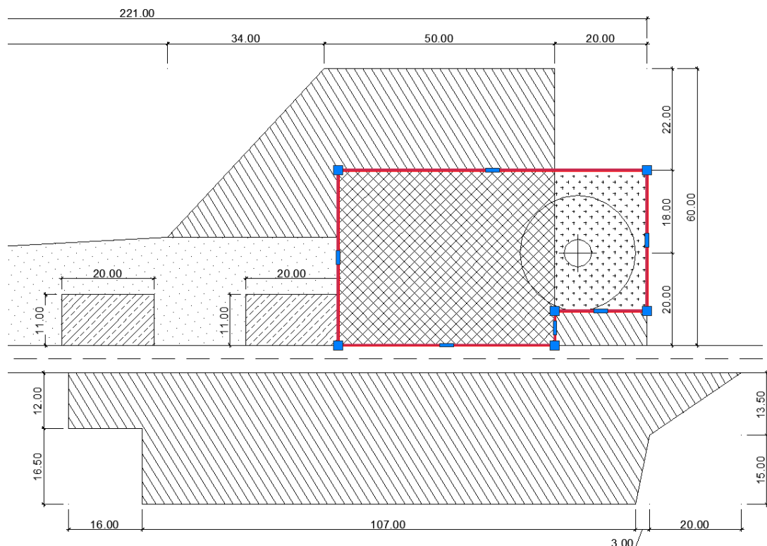
Figura 3-4: Piazzola – parte definitiva
