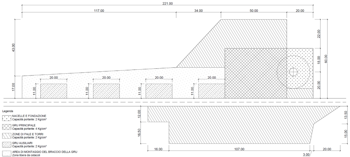
Figura 3-3: Dimensioni piazzola montaggio e di esercizio
