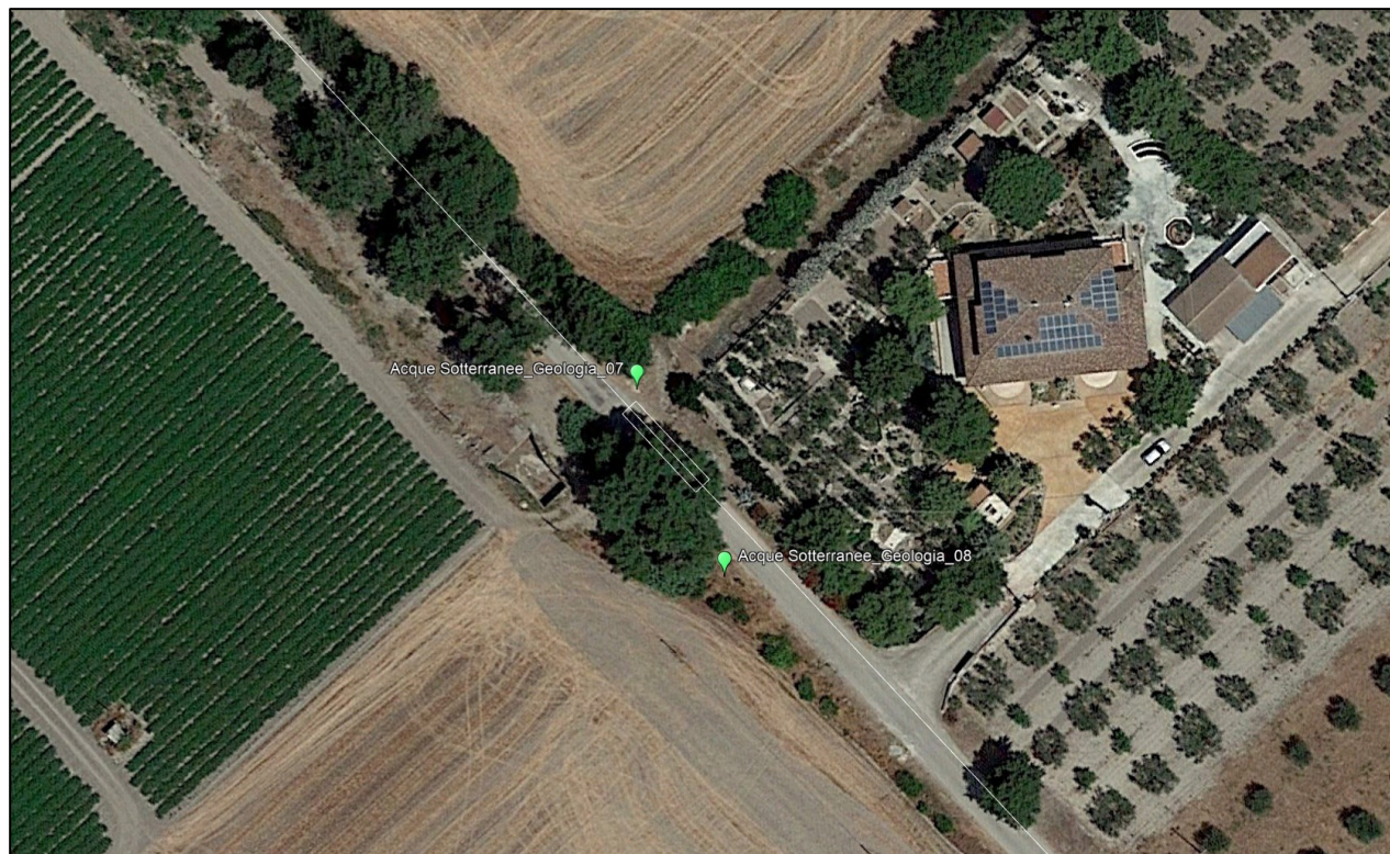
Figura 14: Secondo riquadratura su base satellitare dei punti di monitoraggio delle acque sotterranee e geologia (puntatori verdi) rispetto al layout di impianto (in bianco).
